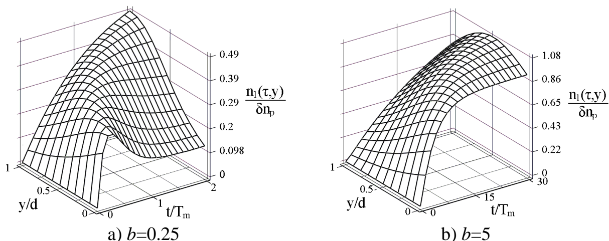
Рисунок 2.7 – Пространственно-временные профили нормированной амплитуды первой гармоники показателя преломления, где b=T_p/T_m , T_m = 1/K^2 D_m – время диффузии мономера, T_p – время полимеризации.
