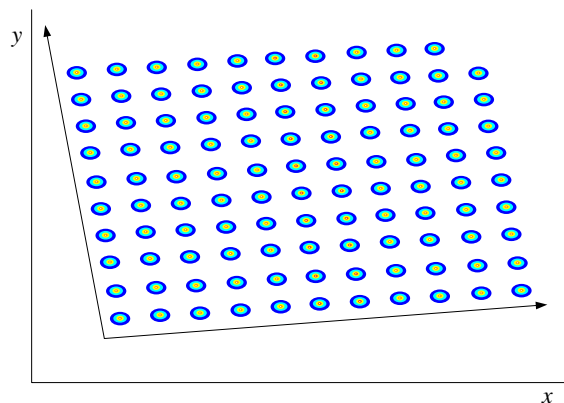
Рис. 2.46 — Картина выходного поля на выходе 2D–AWG-демультиплектора
