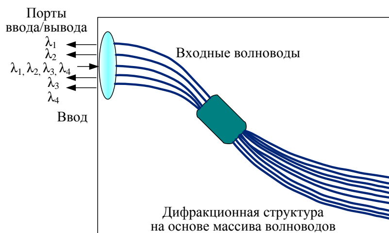
Рис. 2.36 — Многопортовый разветвитель
