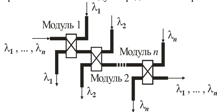
Рис. 2.16 — Мультиплексор/демультиплексор на основе интерферометров Маха — Цендера
