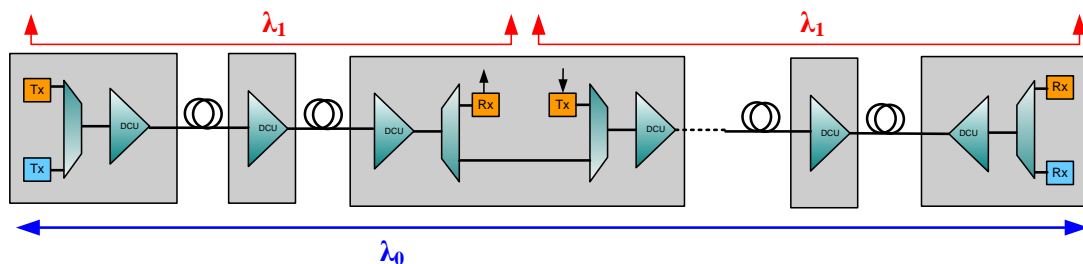
Рис. 2.44 — Конфигурация «многоточка — многоточка»
