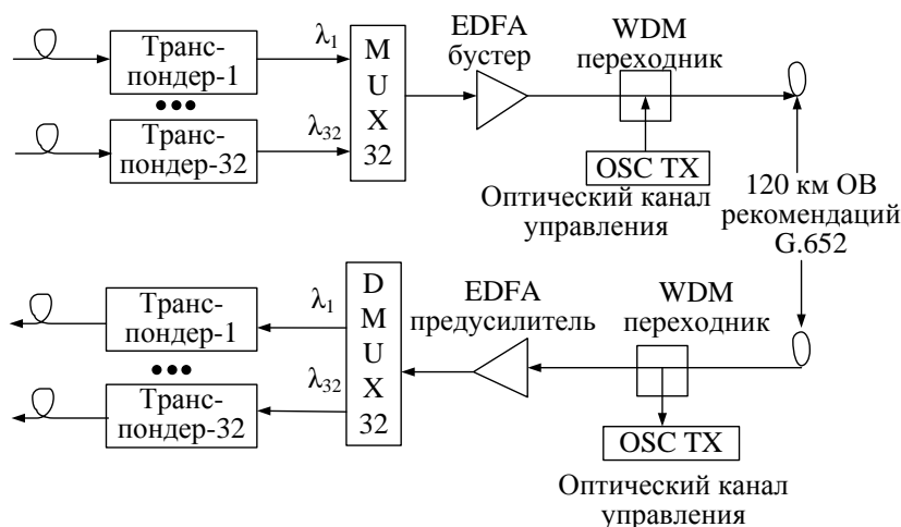
Рис. 1.13 — Структура ОТМ OptiX BWS 320G
