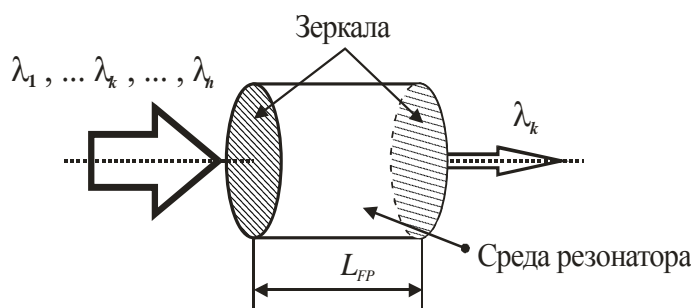
Рис. 2.26 — Конструкция фильтра на основе резонатора Фабри — Перо: L — длина резонатора
