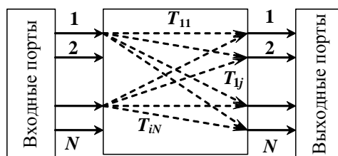
Рис. 1.20 — Структурная схема AWG
