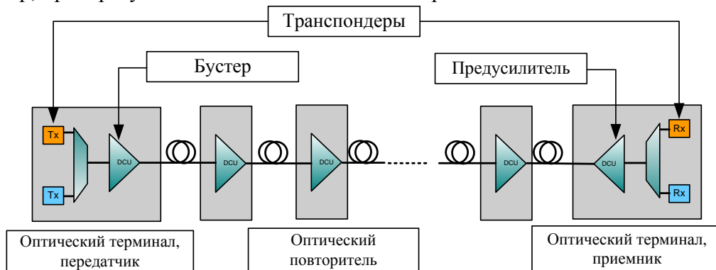
Рис. 2.43 — Конфигурация «точка — точка»
