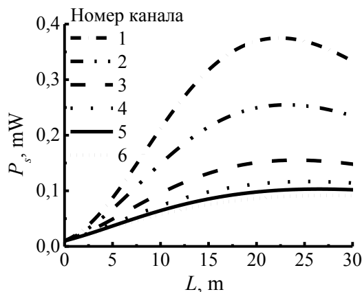
Рис. 2.7 — Зависимость мощности сигнала от длины волокна
