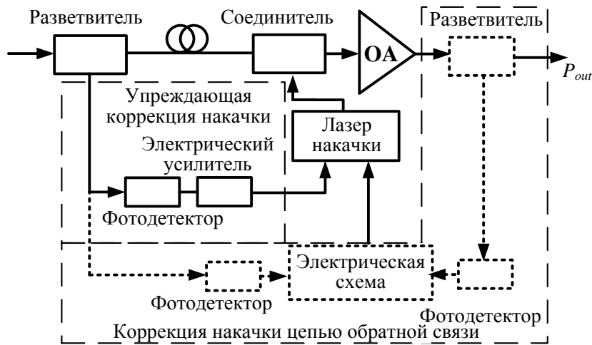
Рис. 1.11 — Электрическая стабилизация коэффициента усиления EDFA
