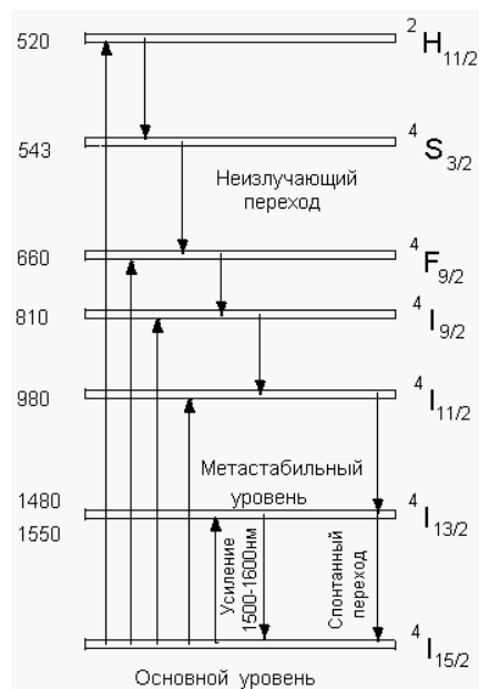
Рис. 2.1 — Диаграмма энергетических уровней для ионов \text{Er}^{3+}
