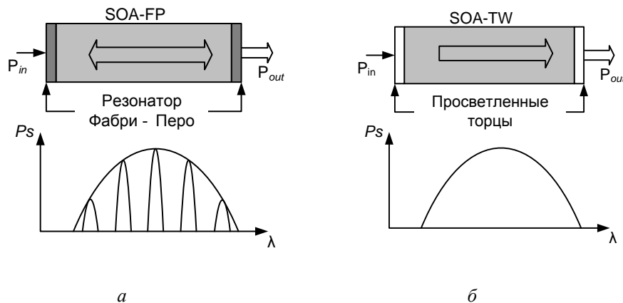
Рис. 1.4 — Схема построения полупроводниковых усилителей
