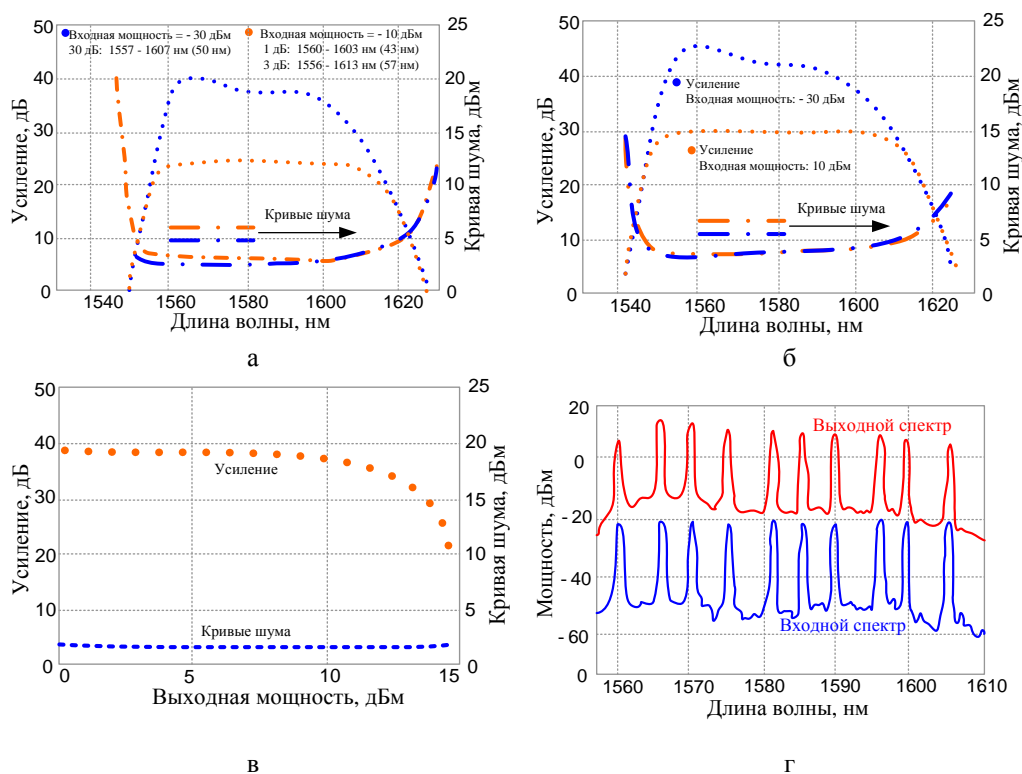
Рис. 2.12 — Зависимость коэффициента усиления и коэффициента шума (а, б), коэффициента усиления и коэффициента шума от входной мощности сигнала (в), входного и выходного сигналов (г) от длины волны для усилителя диапазона L
