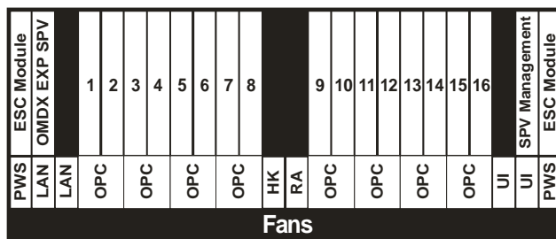
Рис. 2.25 — Конфигурация стойки
