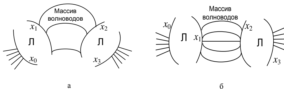
Рис. 2.37 — Конфигурация AWG (а) и XWG (б)
