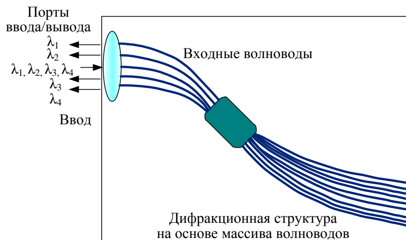
Рис. 2.36 — Многопортовый разветвитель
