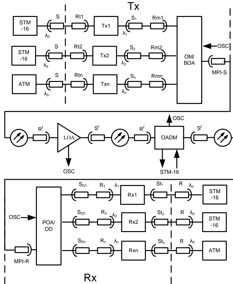
Рис. 1.1 — Структурная схема волоконно-оптической системы связи со спектральным уплотнением каналов [4]:
