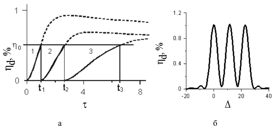
Рис. 2.35 — Динамика дифракционной эффективности (а) и зависимость нормированной дифракционной эффективности от расстройки Брегга (б) для трех последовательно записываемых НДР
