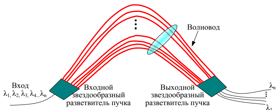
Рис. 1.19 — Структура AWG-демультиплексора
