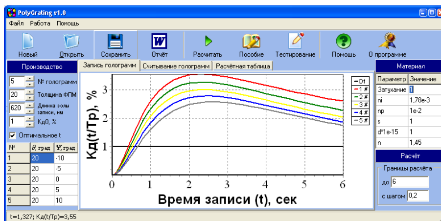
Рис. 4.15 — Главное окно программы PolyGrating
