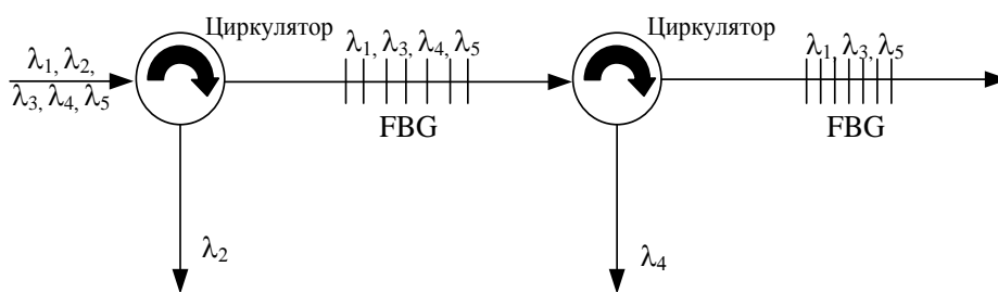
Рис. 1.15 — Схема демultipлексора WDM на основе решетки Брэгга
