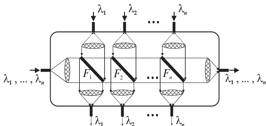
Рис. 2.14 — Мультиплексор/демультиплексор на основе многоступенчатой системы тонкопленочных фильтров: F_1, F_2, \dots, F_n — набор фильтров, настроенных на свою длину волны
