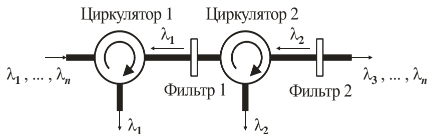
Рис. 2.17 — Демультиплексор на основе циркулятора
