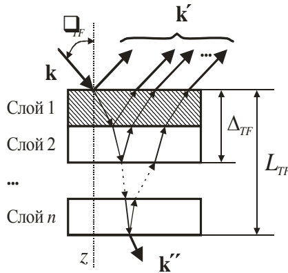
Рис. 2.19 — Брегговское отражение
