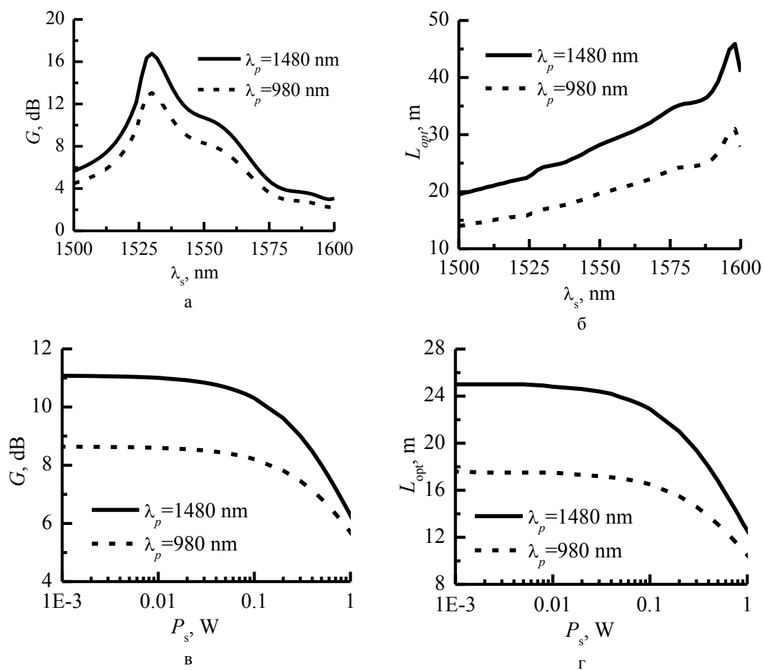
Рис. 2.6 — Зависимость коэффициента усиления и оптимальной длины волокна от длины волны и мощности сигнала
