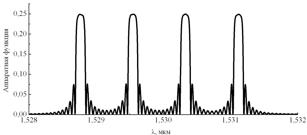
Рис. 2.23 — Аппаратная функция демультиплектора на основе интерференционных фильтров
