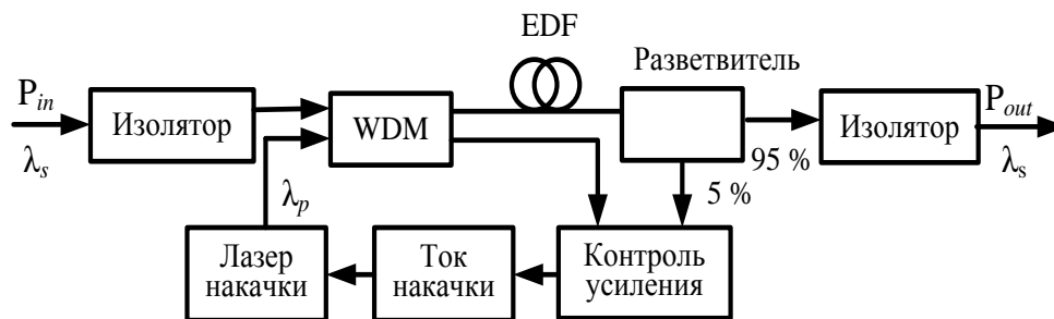
Рис. 1.5 — Функциональная схема DFA
