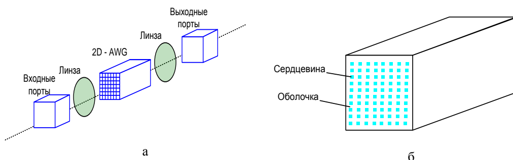
Рис. 2.45 — Схема двумерного мультиплексирования: а — схема; б — устройство 2D-AWG
