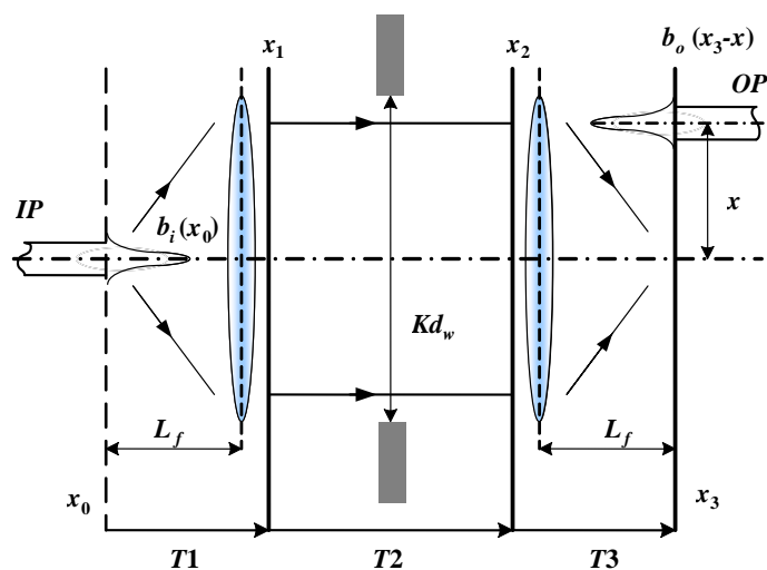
Рис. 2.40 — Соответствие операторов преобразования физическому прохождению сигнала
