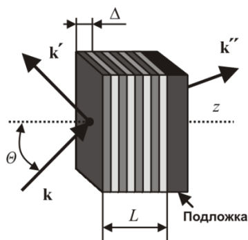
Рис. 2.13 — Конструкция интерференционного фильтра:
