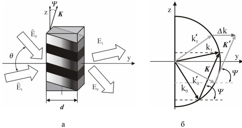
Рис. 2.33 — Пространственная геометрия (а) и векторная диаграмма (б) нестационарного взаимодействия световых волн с голографической решеткой в ФПМ для несимметричной модели записи
