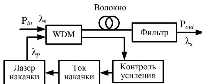
Рис. 1.7 — Схема волоконного рамановского оптического усилителя
