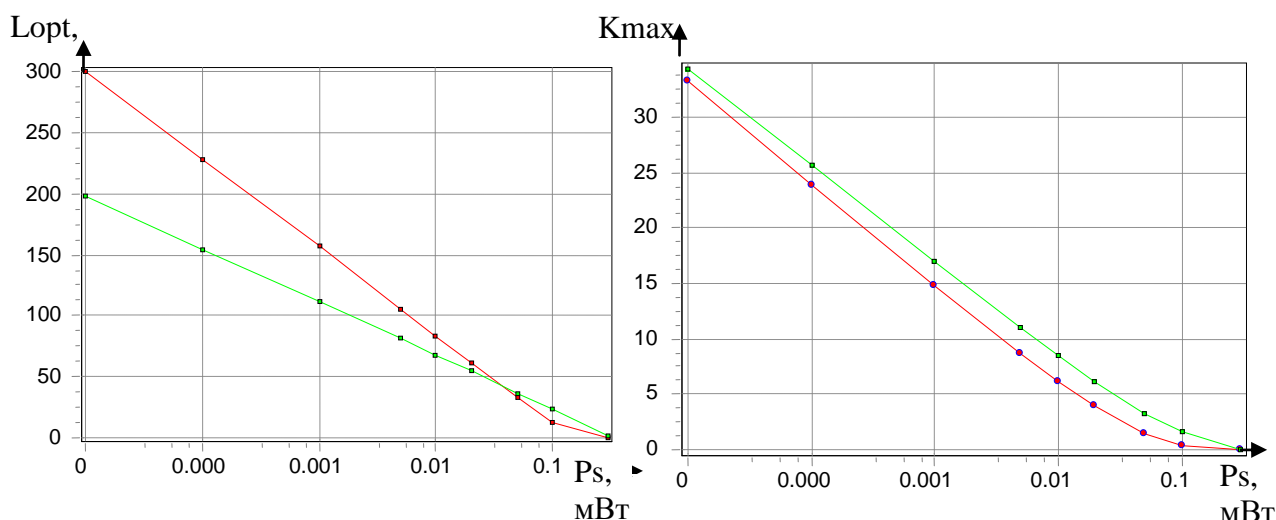
Рисунок 3.1.1 - Зависимость L_{opt}(P_s) и K_{max}(P_s)
