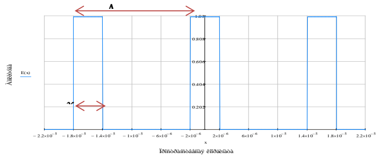
Рисунок 2.5 – График функции пропускания амплитудного транспаранта с периодом \Lambda = 16 мкм
