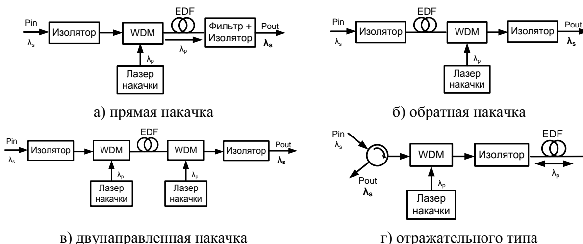
Рисунок 1.8. Основные схемы построения EDFA.
