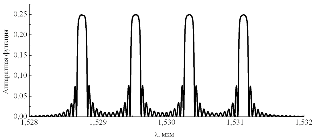
Рисунок 2.11 – Аппаратная функция демультимплектора на основе интерференционных фильтров.
