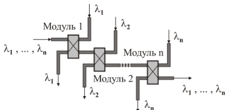
Рисунок 2.4 – Мультиплексор/демультиплексор на основе интерферометров Маха-Цендера.
