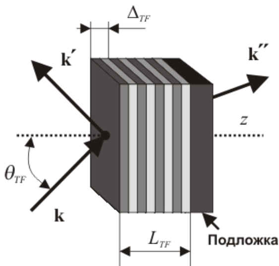
Рисунок 2.1 – Конструкция интерференционного фильтра, где n_1 и n_2 – показатели преломления слоев, L_{TF} – толщина структуры, \Delta_{TF} – период структуры, \mathbf{k} , \mathbf{k}' , \mathbf{k}'' – волновые вектора падающей, отражённой и прошедшей световых волн, \theta_{TF} – угол падения волн.
