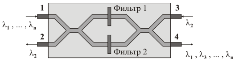
Рисунок 2.3 – Модуль мультиплексирования/демультиплексирования одного канала, на основе интерференционных фильтров и интерферометра Маха-Цендера.
