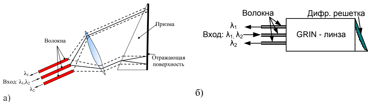
Рисунок 1.12 Схема демультиплексора WDM (а) – на отражательной призме, (б) – на отражательной плоской решетке
