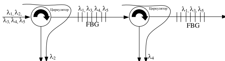
Рис. 1.11 -Схема демультиплексора WDM на основе решеток Брэгга
