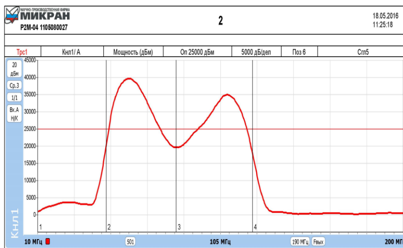
Рисунок 2.5– Анализ спектра излучения в широкополосном режиме
