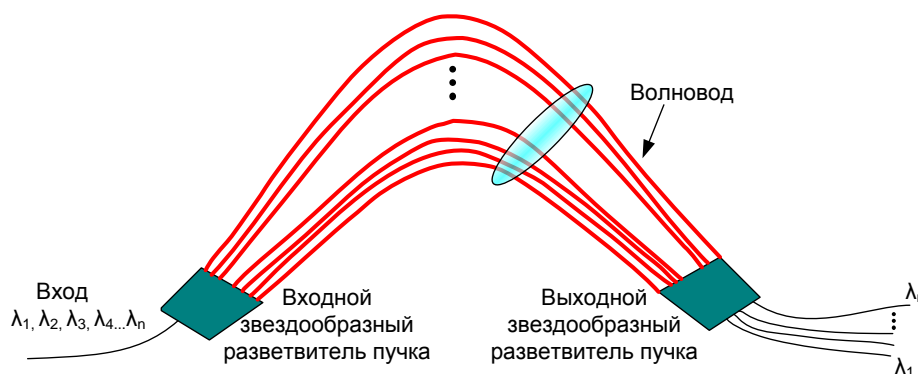
Рис. 1.15 - Структура AWG демультиплексора
