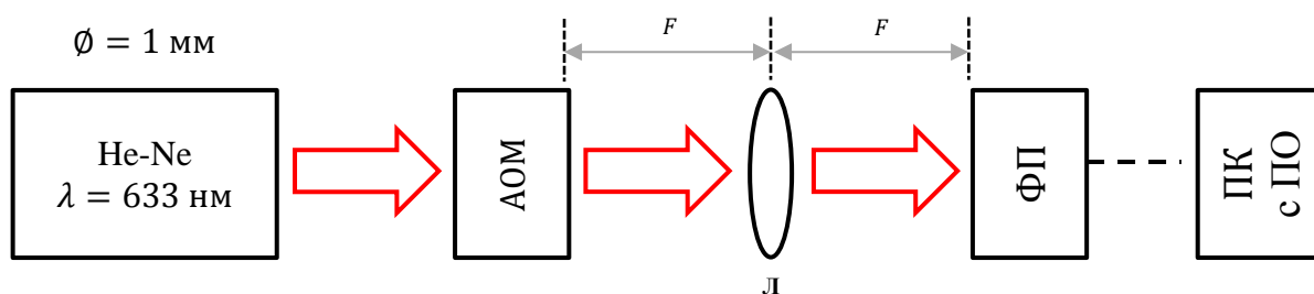
Рисунок 2.1 – Схема экспериментальной установки для измерения полосы частот
