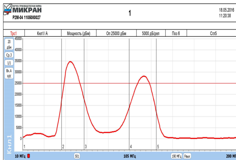
Рисунок 2.4 – Частотная характеристика АОАС в узкополосном режиме
