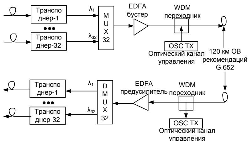
Рис. 1.9 - Структура OTM OptiX BWS 320G
