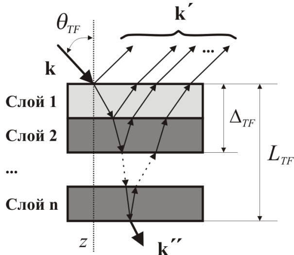
Рисунок 2.7 – Брэгговское отражение
