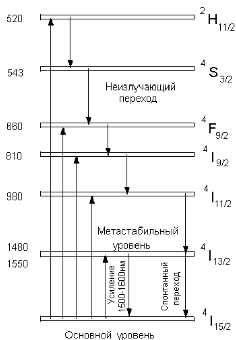
Рисунок 1.6- Диаграмма энергетических уровней для ионов Er^{3+} .
