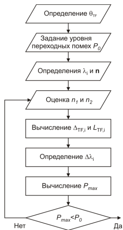
Рисунок 2.10 – Блок-схема построения демультимплектора на основе интерференционных фильтров.
