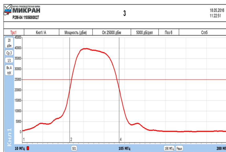
Рисунок 2.6 – Частотная характеристики в режиме слияния дифракционных максимумов частотной характеристики
