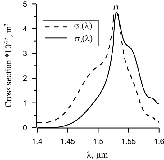
Рисунок 2.2 - Эффективные сечения поглощения ( \sigma_a ) и излучения ( \sigma_e ).
