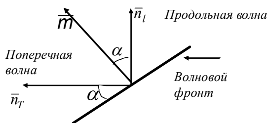
Рисунок 1 – Ориентация упругой волны в анизотропном кристалле
