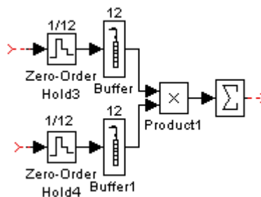
Рисунок 2.8 – Реализация корреляционного приемника
