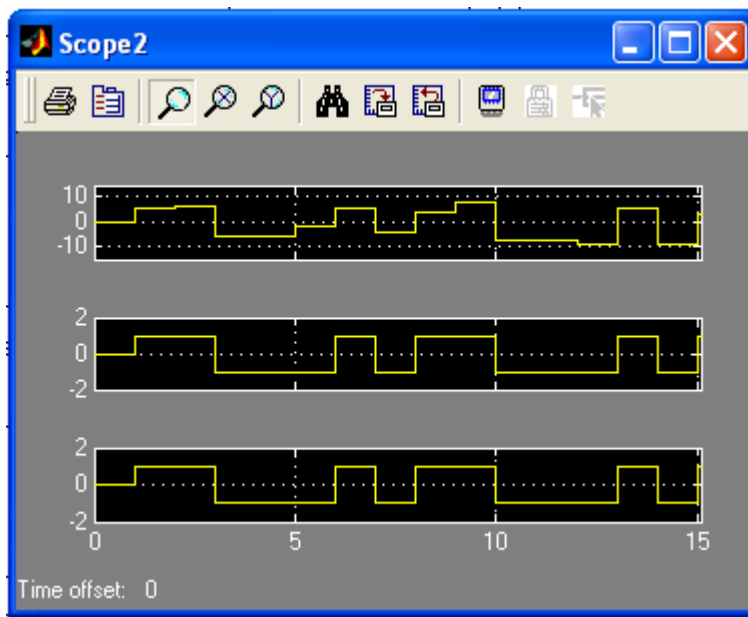
Рисунок 3.5 - Фрагменты осциллограмм на выходе коррелятора 1-го канала до и после нормирования по амплитуде и передаваемые биты в отсутствие шумов канала распространения
