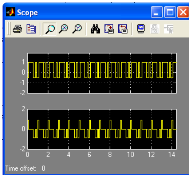
Рисунок 3.1 - Фрагменты осциллограмм повторяющейся композитной комплекснозначной расширяющей последовательности 1-го канала
