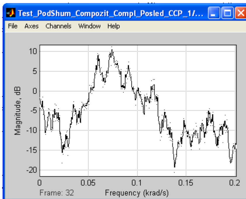
Рисунок 3.4 - Спектрограмма сигнала 4-х канального модема передачи на основе композитных комплекснозначных последовательностей в отсутствие шумов канала распространения
