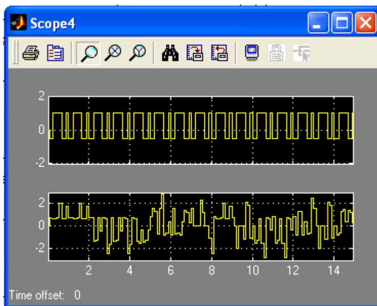
Рисунок 3.3 - Фрагменты осциллограмм отсчетов накапливаемых в плечах коррелятора 1-го канала в отсутствие шумов канала распространения
