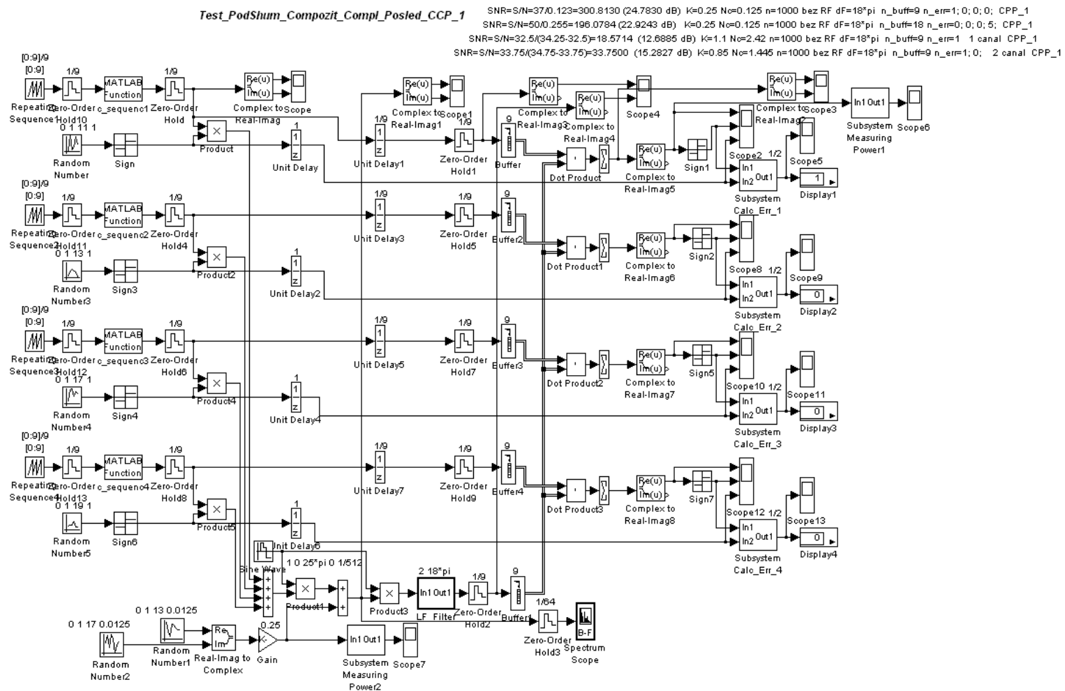
Рисунок 2.1 – Функциональная модель 4-х канального модема на основе композиционных комплекснозначных последовательностей
