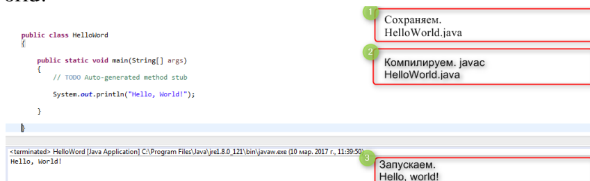
Рисунок 1.16 – Запуск программы, написанной на языке Java
