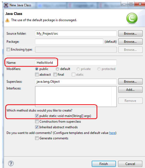
Рисунок 1.10 – Создание нового класса
