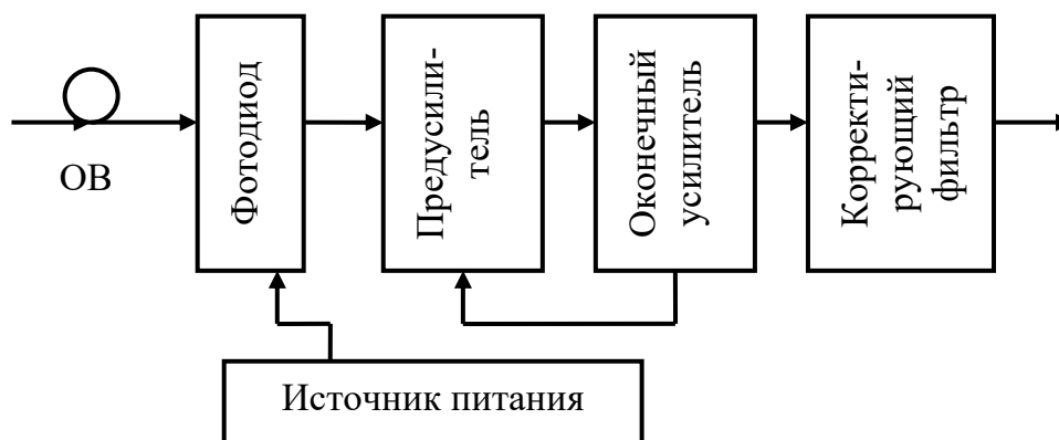
Рисунок 1.2 – Схема фотоприемного устройства
