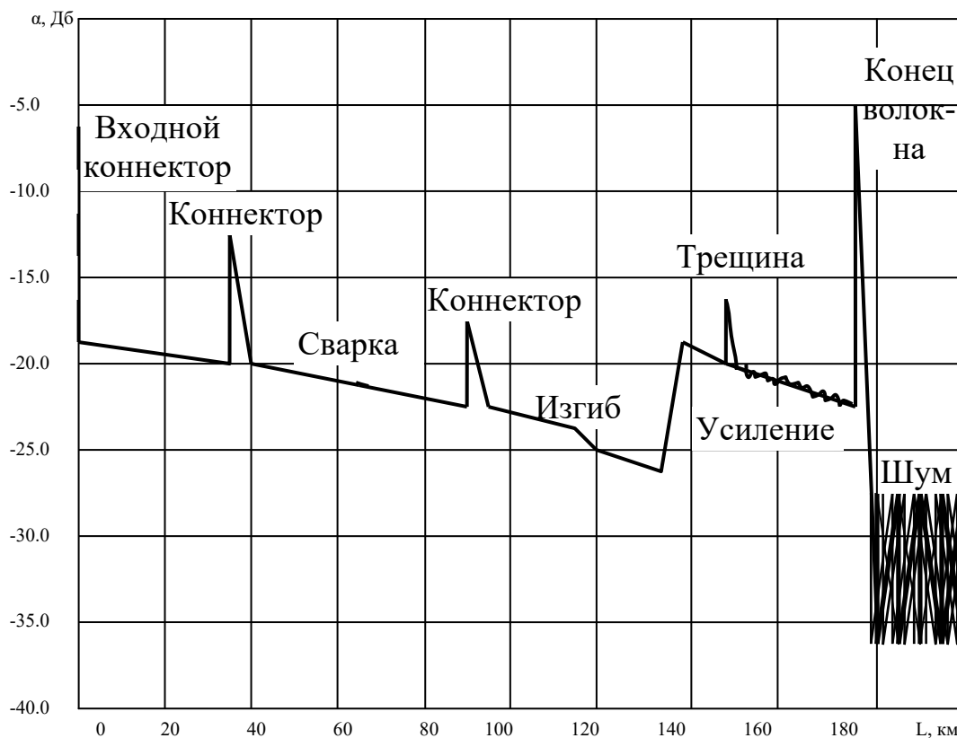
Рисунок 8.2 – Типичная рефлектограмма ВОЛС
