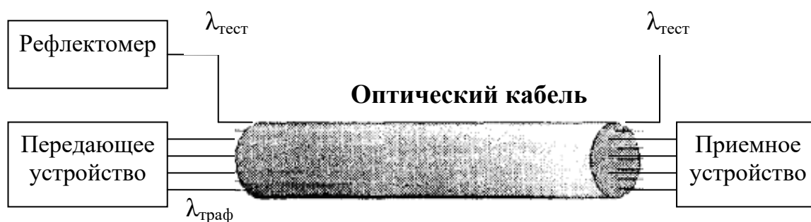
Рисунок 10.1 – Метод контроля оптического кабеля по пассивному волокну
