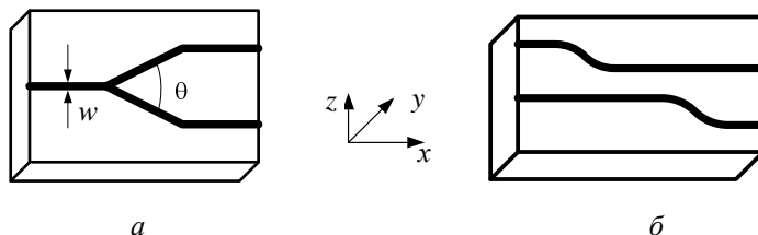
Рис. 3.8. Канальные волноводные Y-разветвитель (а) и направленный ответвитель (б)
