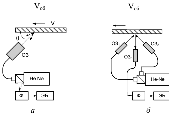
Рис. 4.15. Схемы лазерных доплеровских измерителей скорости: а — с опорным световым сигналом; б — дифференциального типа
