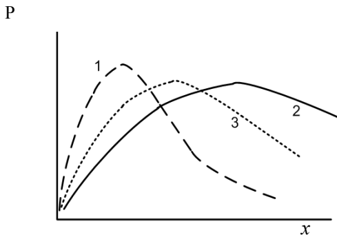
Рис. 4.9. Вид зависимостей выходного сигнала датчика с отражательной диафрагмой от деформации диафрагмы для разных способов укладки передающих и приемных ВС в жгуте (см. рис. 4.8)
