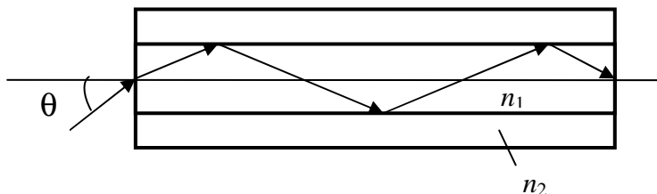
Рис. 3.13. Распространение светового луча в волоконном световоде
