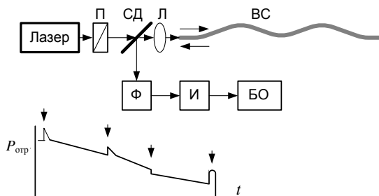
Рис. 8.5. Схема измерения распределения неоднородностей по длине ВС методом импульсной временной рефлектометрии:
