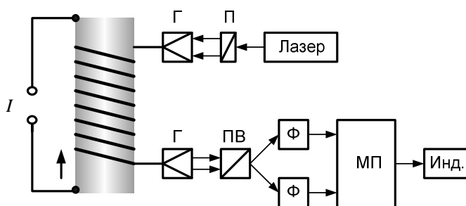
Рис. 5.4. Схема ВО измерителя тока:
