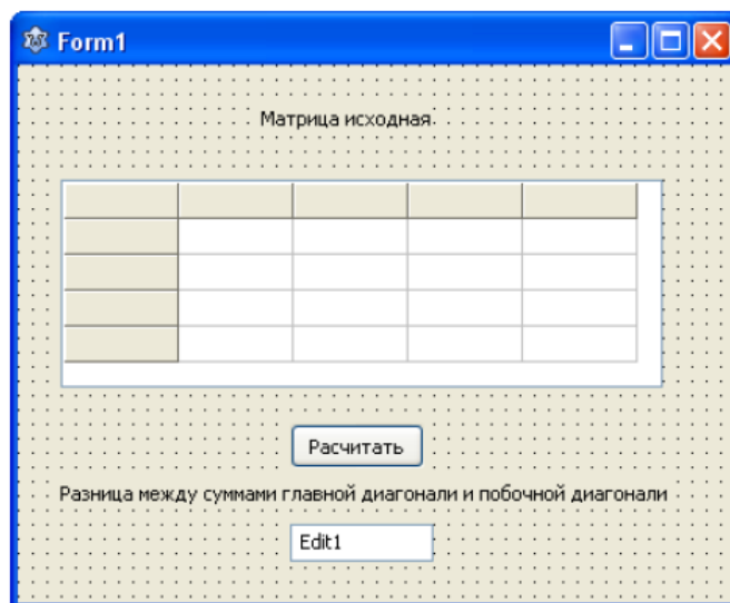
Рис. 9.1 - Интерфейс программы
