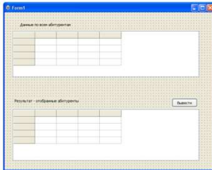
Рис. 8.1 – Интерфейс программы
