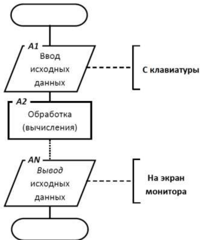
Рис. 3.1 – Линейный алгоритм
