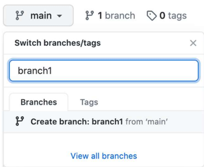
Рис. 28. — Создание ветки
