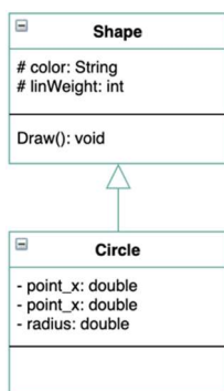
Рис. 16. — Наследование
