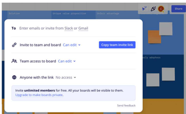
Рис. 4. — Добавление участников
