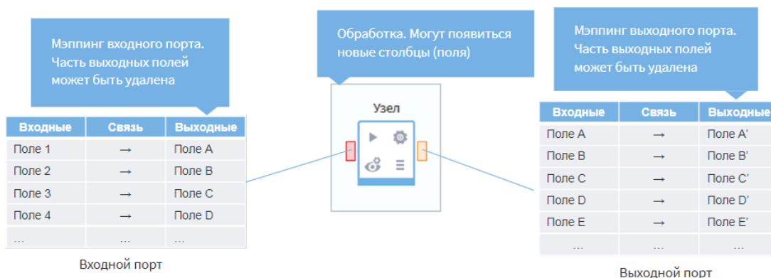
Рисунок 2.30 – Пример мэппинга полей
