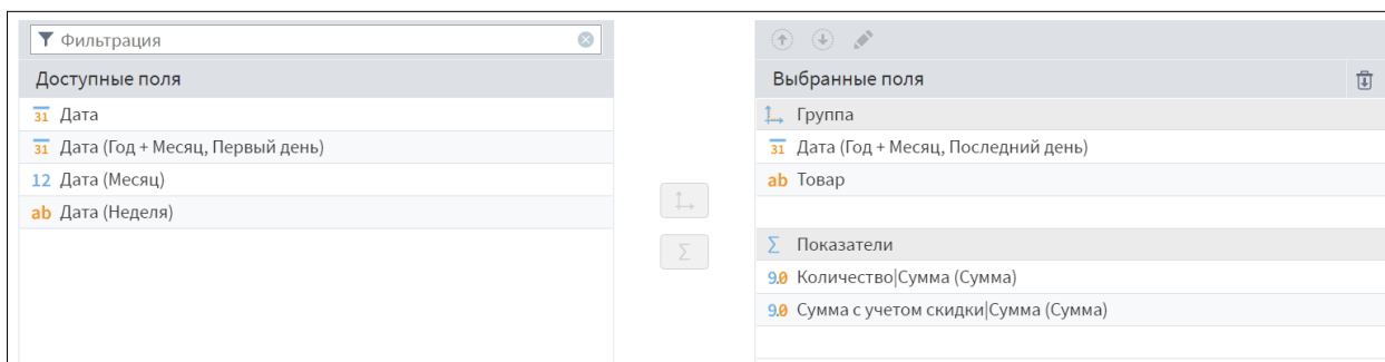
Рисунок 3.20 – Пример настройки узла Группировка
