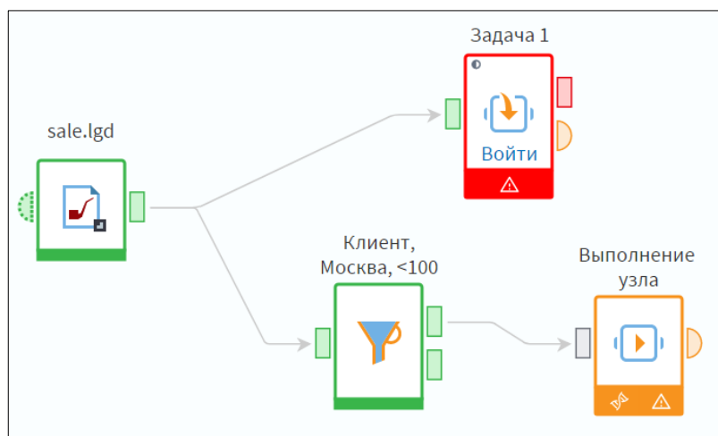
Рисунок 2.77 – Создание подмодели Задача 1
