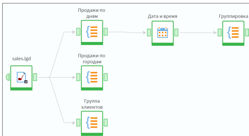
Рисунок 3.19 – Пример установления связей между узлами
