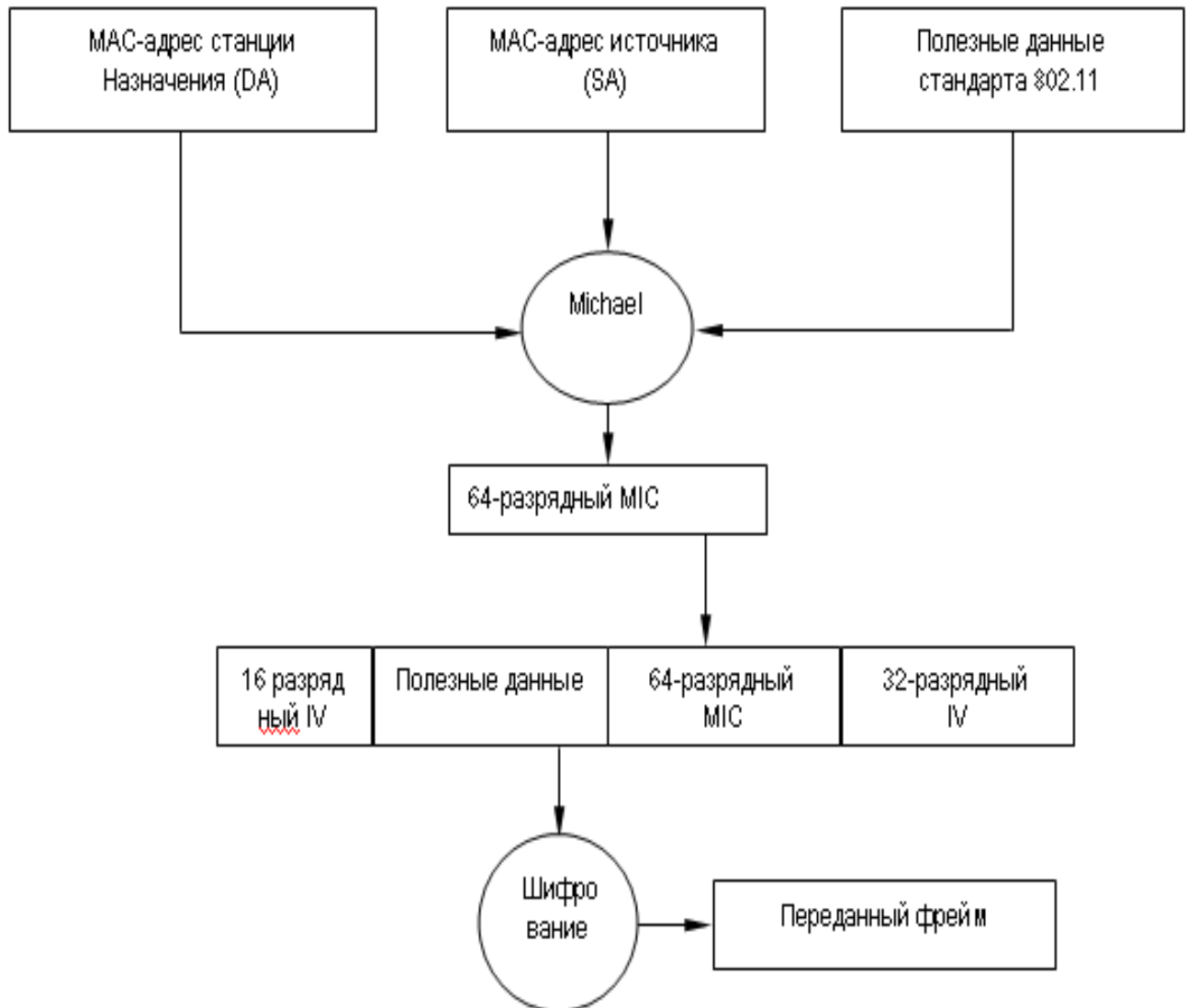
Рис. 30. Работа алгоритма MIC
