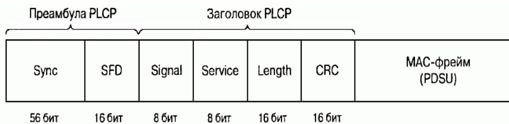
Рис. 16 Короткий PPDU технологии HR-DSSSS
