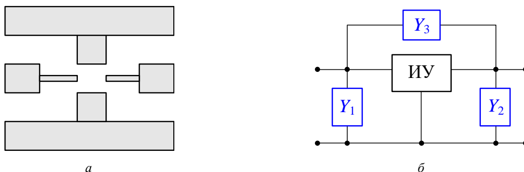
Рисунок 3.2 – Эскиз стандарта деэмбеддинга «Open» (а) и ЭС (б)
