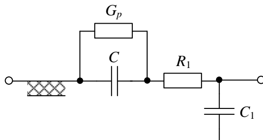
Рисунок 2.5 – Структура ЭС-модели МДМ конденсатора, учитывающая распределённые эффекты
