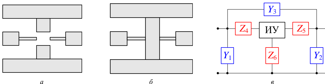
Рисунок 3.3 – Эскиз стандартов деэмбеддинга «Open» (а), «Short» (б) и ЭС (в)
