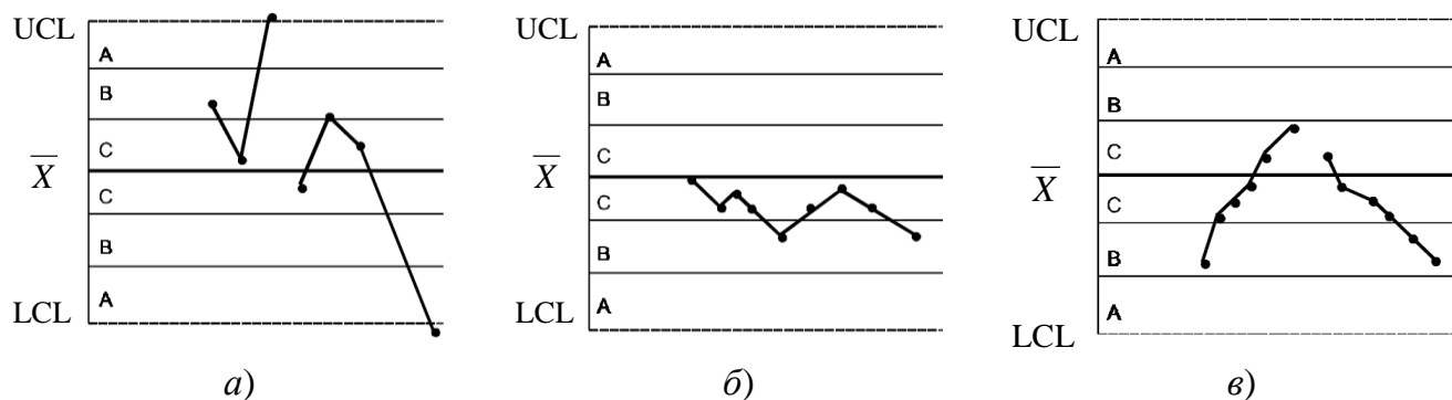
Рисунок 1.4 – Примеры критериев неуправляемого процесса для контрольных карт:
