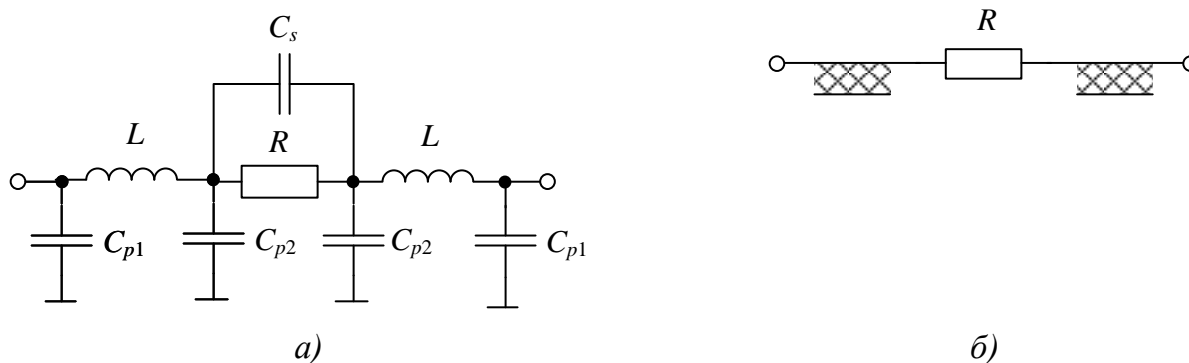
Рисунок 2.3 – Структуры ЭС-модели монолитного резистора, учитывающие распределённые эффекты
