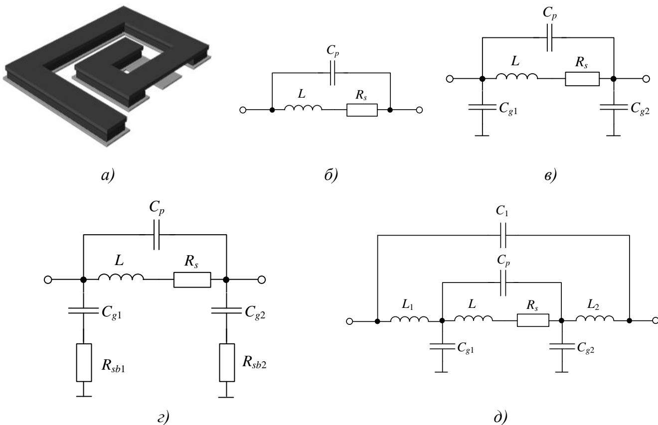
Рисунок 2.6 – Внешний вид (а) и структуры ЭС (б, в, г, д) спиральной катушки индуктивности
