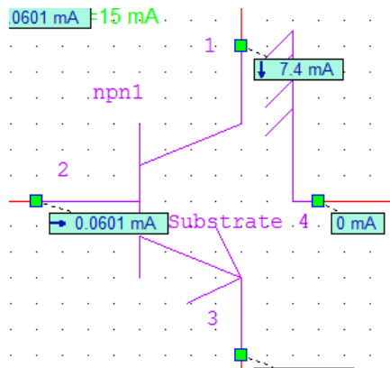
Фрагмент цепи с рассчитанными узловыми токами.
