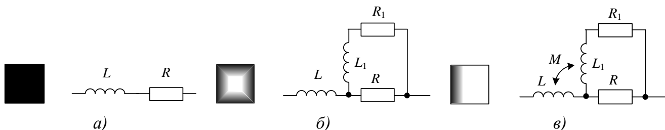
Рисунок 2.7 – Распределение плотности тока в сечении проводника катушки индуктивности и фрагмент ЭС для моделирования при а) низких частотах, б) скин-эффекте, в) эффекте близости
