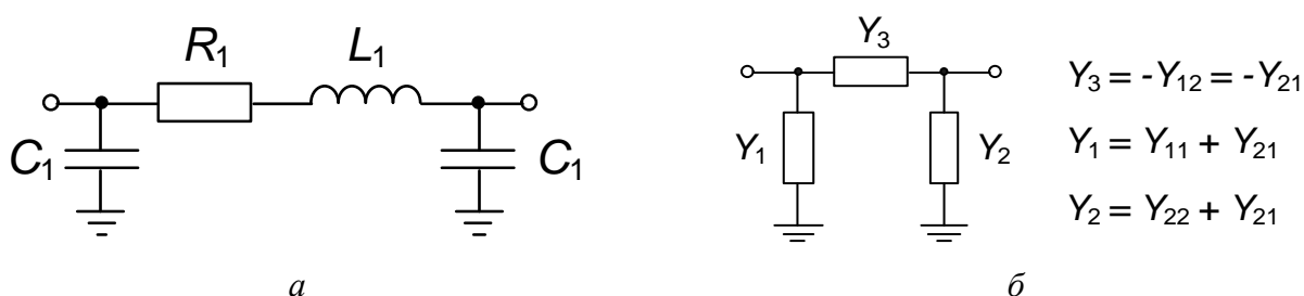
Рисунок 3.4 – ЭС-модель резистора (а) и её представление через Y -параметры в виде П-звена (б)
