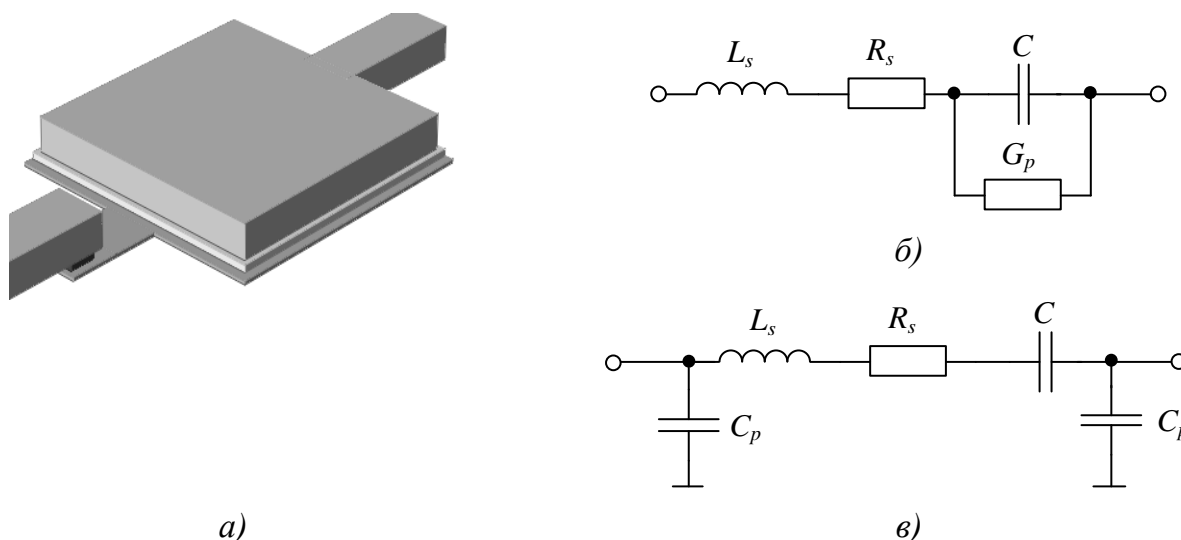
Рисунок 2.4 – Внешний вид (а) и структуры ЭС (б, в) МДМ конденсатора
