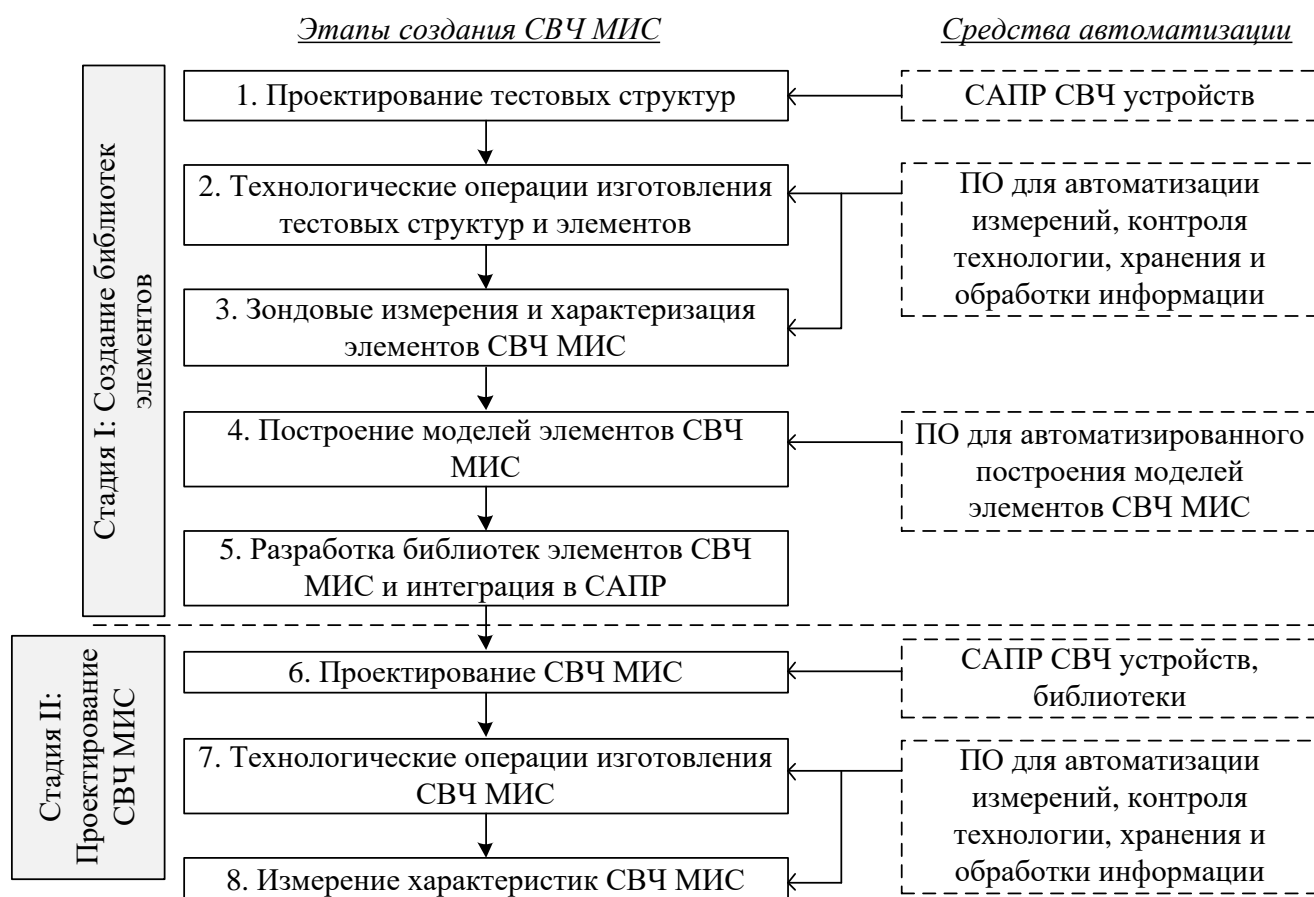
Рисунок 1.1 – Схема процесса проектирования и изготовления МИС на отечественной технологии и средства его автоматизации
