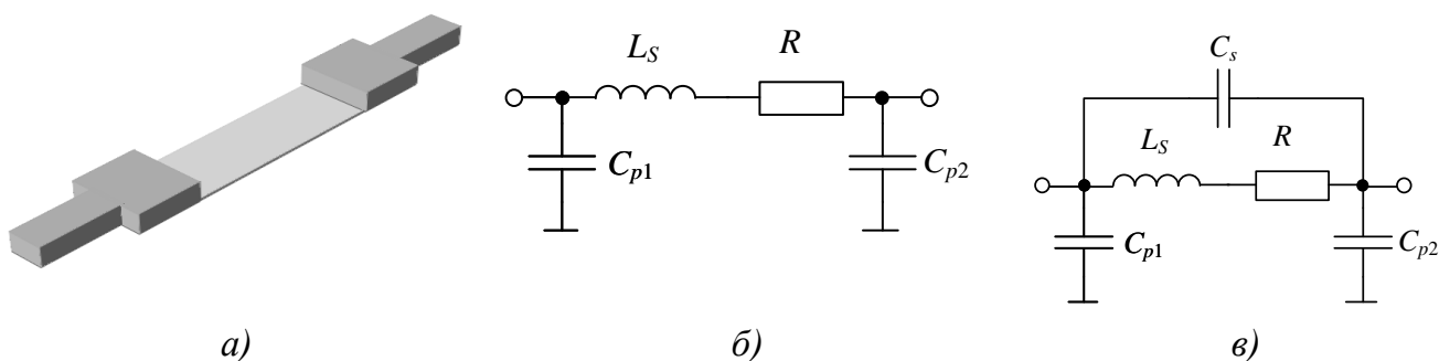
Рисунок 2.2 – Внешний вид (а) и структуры ЭС (б, в) монолитного резистора
