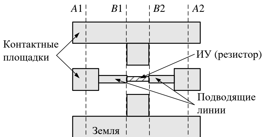
Рисунок 3.1 – Эскиз тестовой структуры с ИУ (тонкоплёночный резистор) для зондовых измерений S -параметров
