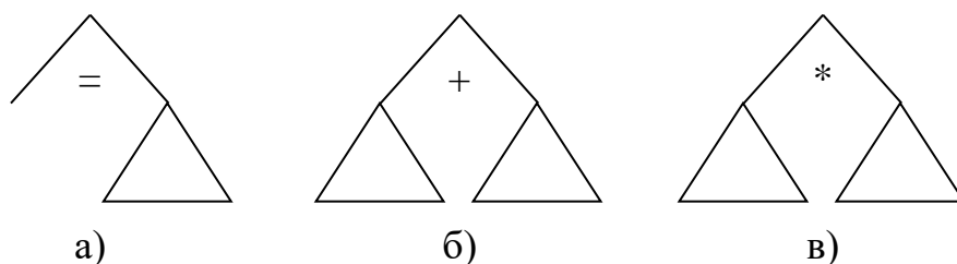
Рисунок 2.2 – Типы вершин
