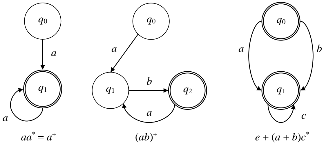
Рисунок 4.3 – Сопоставление графа переходов ДКА и РВ (окончание)
