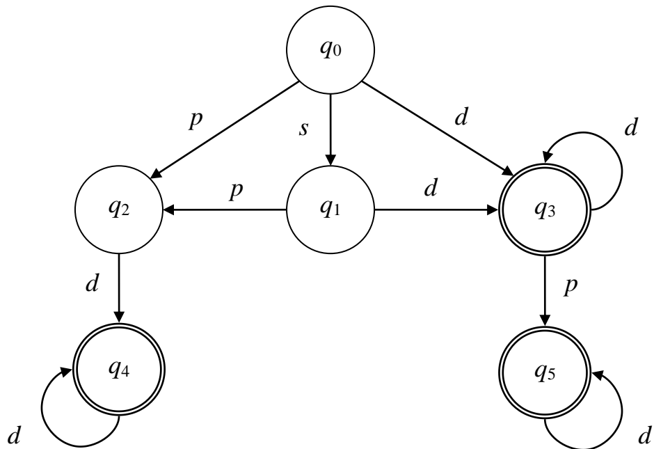
Рисунок 4.4 – Граф переходов ДКА, построенный по РВ
