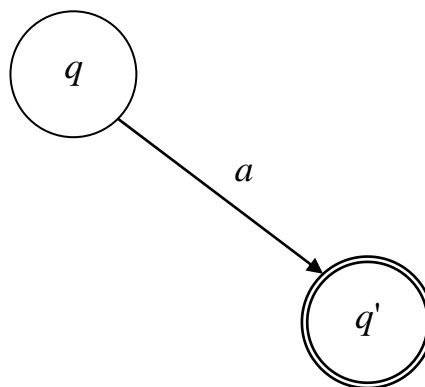
Рисунок 3.3 – Переход в конечное состояние ДКА
