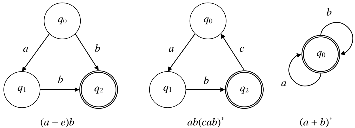
Рисунок 4.2 – Сопоставление графа переходов ДКА и РВ
