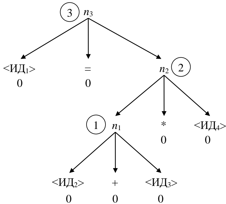
Рисунок 2.3 – Дерево с уровнями
