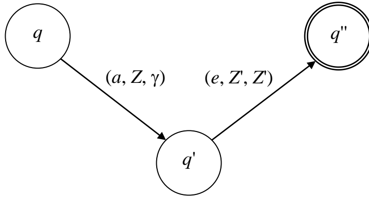
Рисунок 3.4 – Переход в конечное состояние ДМПА
