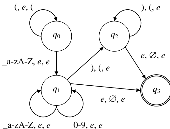
Рисунок 3.7 – Граф ДМПА, описывающего идентификатор в скобках
