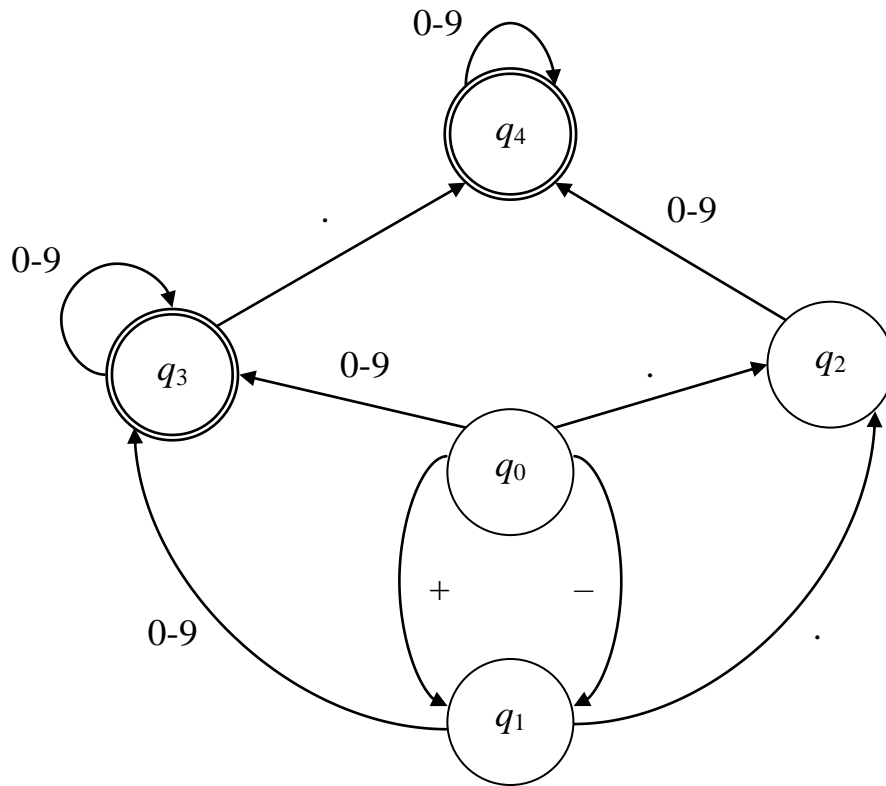
Рисунок 3.6 – Минимизированный граф ДКА, описывающего число с фиксированной точкой
