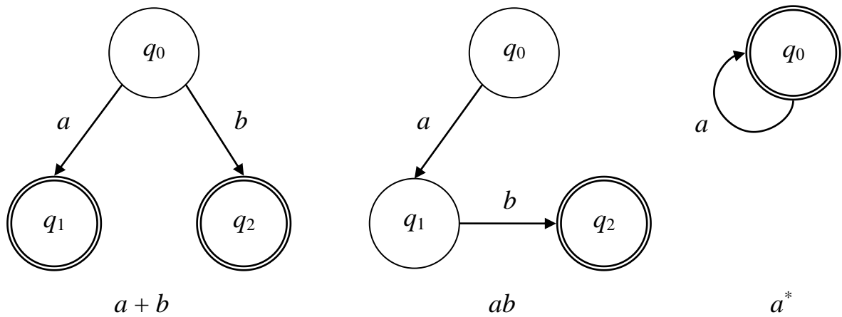
Рисунок 4.1 – Сопоставление графа переходов ДКА и базовых операций РВ
