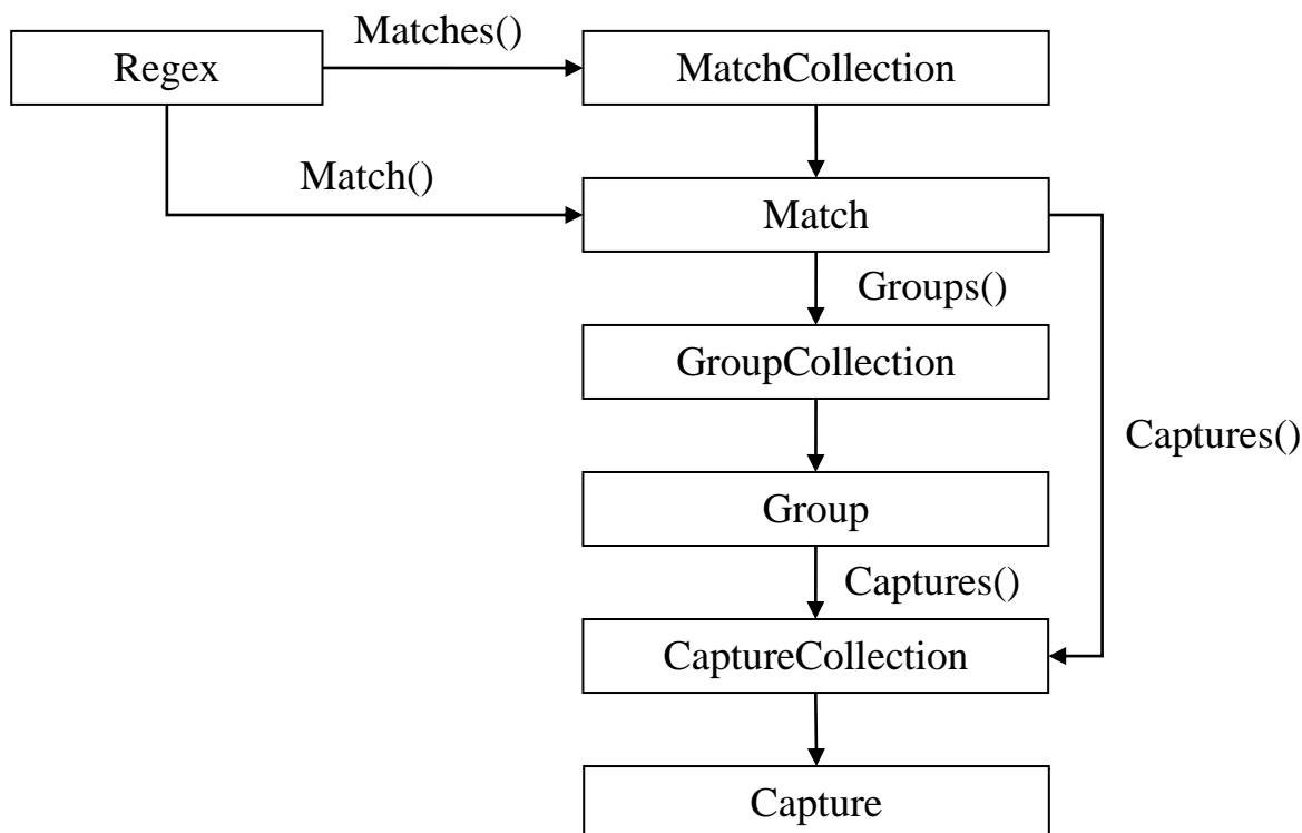
Рисунок 4.4 – Схема обработки соответствий при использовании класса Regex
