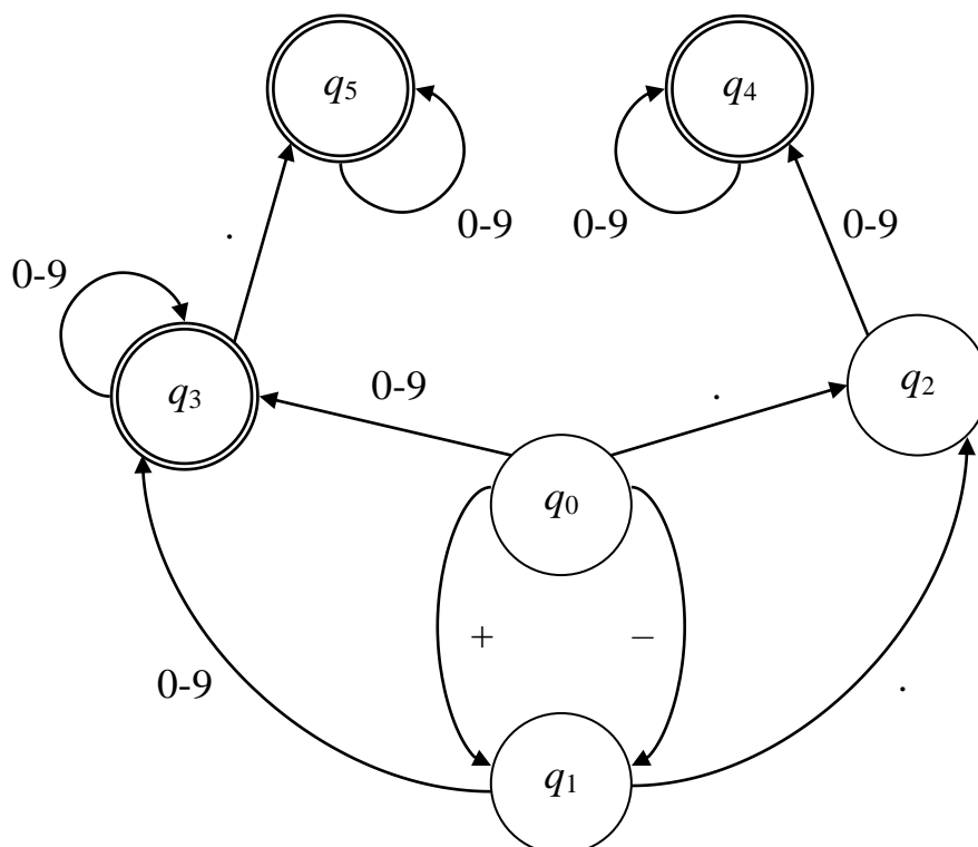
Рисунок 3.5 – Граф ДКА, описывающего число с фиксированной точкой
