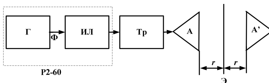
Рисунок 2.3 – Схема метода плоского экрана
