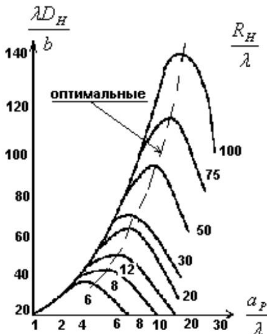
Рисунок 1.2 – Зависимость КНД H -секториального рупора D_H от размера раскрыва при постоянных длинах
