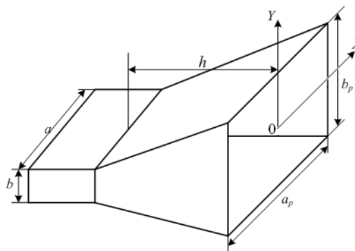
Рисунок 1.1 – Пирамидальная рупорная антенна
