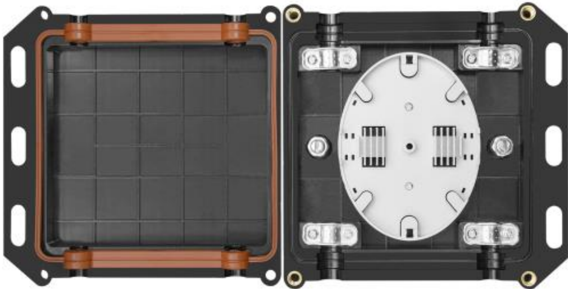
Рисунок 4.3.1 – Открытие муфты
