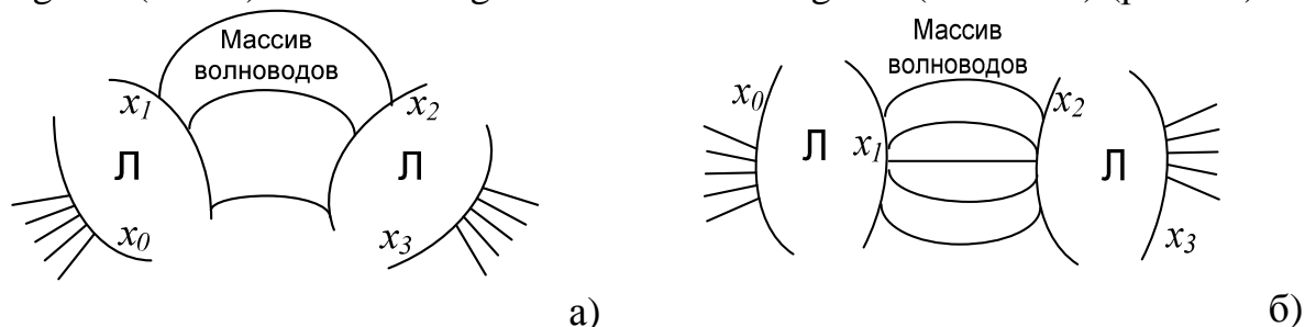
Рис. 2.2 – Конфигурация а) AWG, б) XWG
