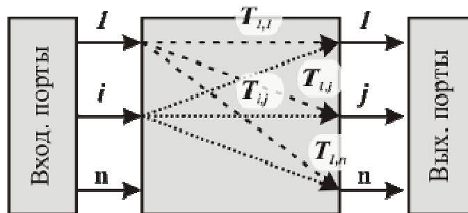
Рисунок 2.1 – Структурная схема распределителя
