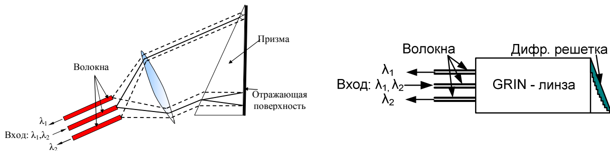
Рисунок 1.12 Схема демультиплексора WDM (а) – на отражательной призме, (б) – на отражательной плоской решетке
