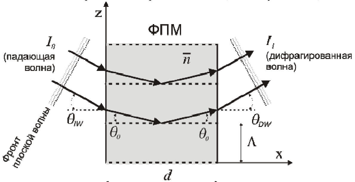
Рисунок 2.10 – Дифракция света на объёмной решётке
