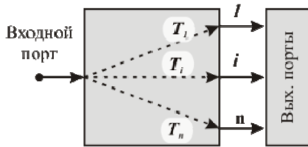
Рисунок 2.2 – Структурная схема демультиплексора
