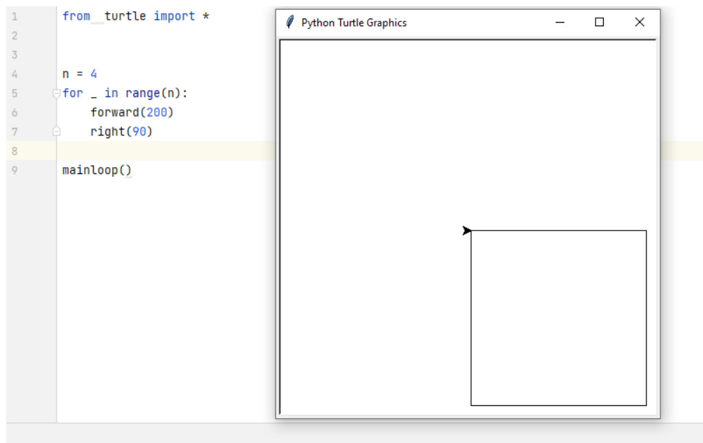
Рисунок 3.1 Программа рисования прямоугольника
