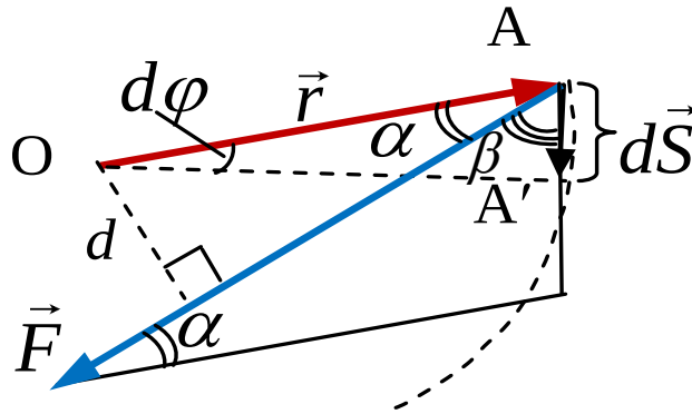
Рисунок 3.3 – Работа, необходимая для вращения твердого тела вокруг неподвижной оси: A - точка приложения силы \vec{F} в начале процесса, A' - точка приложения силы \vec{F} в конце процесса, d\vec{S} - модуль вектора перемещения, d\varphi - угловое перемещение, d –плечо силы.
