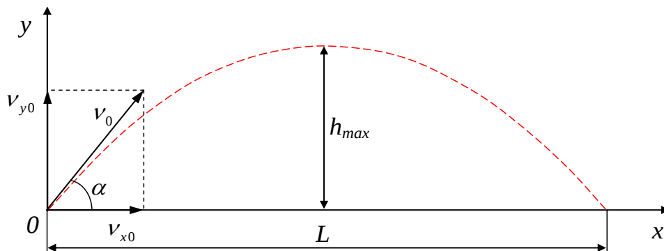
Рисунок 1.4 – Движение тела, брошенного под углом к горизонту.
