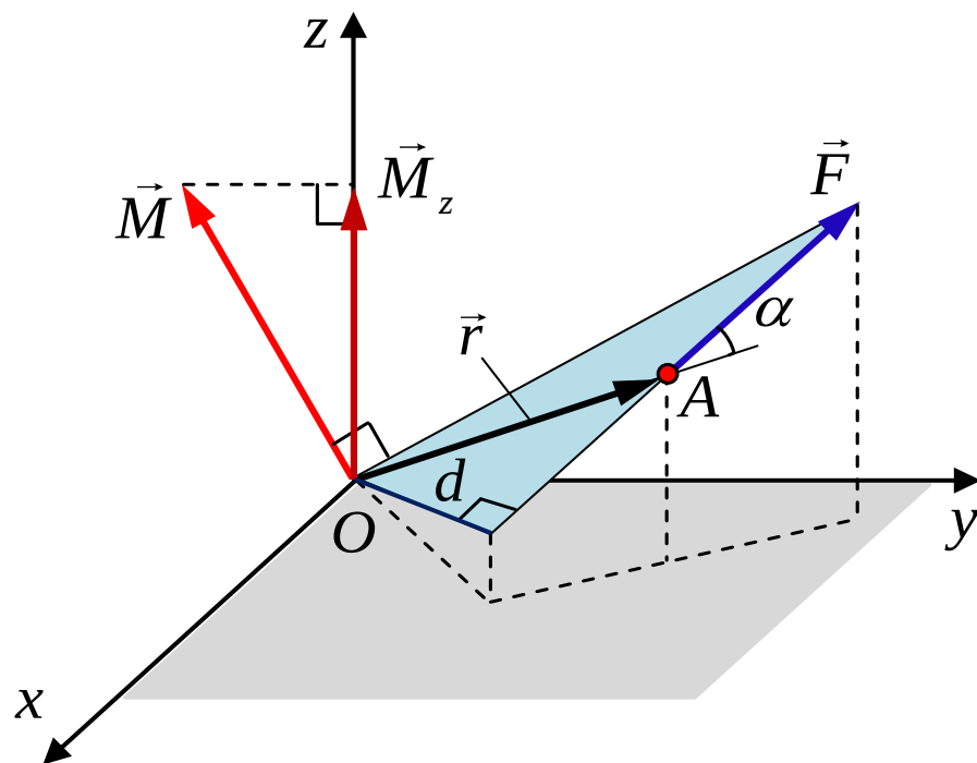
Рисунок 2.4 – Момент силы \vec{F} относительно точки O .
