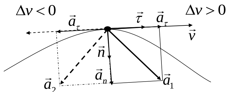
Рисунок 1.3 - Линейные ускорения при криволинейном движении, \vec{a}_1 - соответствует \Delta v > 0 , \vec{a}_2 - соответствует \Delta v < 0 .
