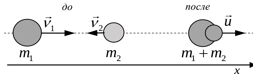
Рисунок 3.4 – Неупругий удар.
