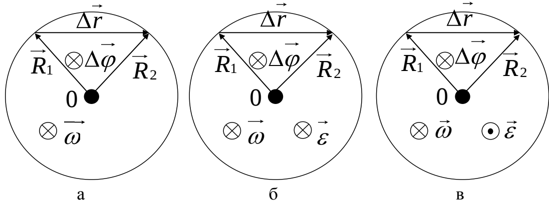
Рисунок 1.5 – Вращательное движение тела, |\vec{R}_1| = |\vec{R}_2| = R :
