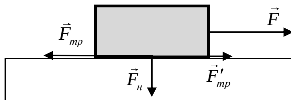
Рисунок 2.2 - \vec{F} - внешняя сила, \vec{F}_n - сила нормального давления, \vec{F}_{тр} , \vec{F}'_{тр} - силы трения.
