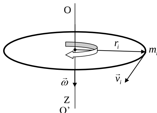
Рисунок 2.3 – Направление угловой скорости
