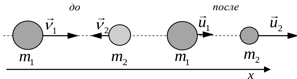
Рисунок 3.5 – Неупругий удар.
