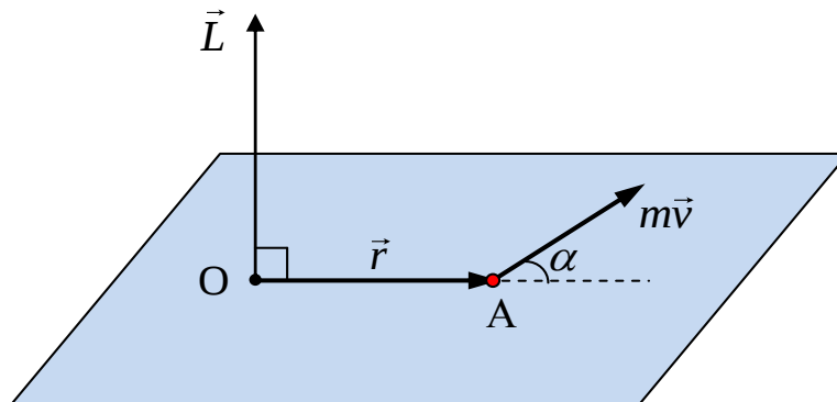
Рисунок 2.5 – Направление момента импульса.
