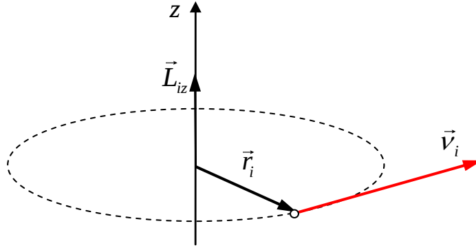
Рисунок 2.6 – Направление проекции момента импульса.
