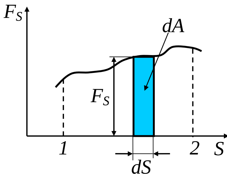
Рисунок 3.2 – Зависимость проекции силы от перемещения.
