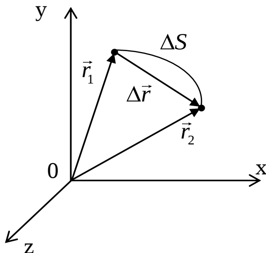
Рисунок 1.1 - Путь и перемещение
