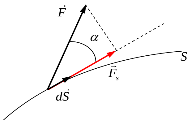
Рисунок 3.1 – Работа при бесконечно малом перемещении.
