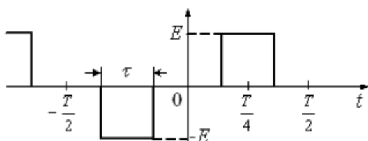
Рисунок 5 – Временные представления сигналов и основные параметры спектра
