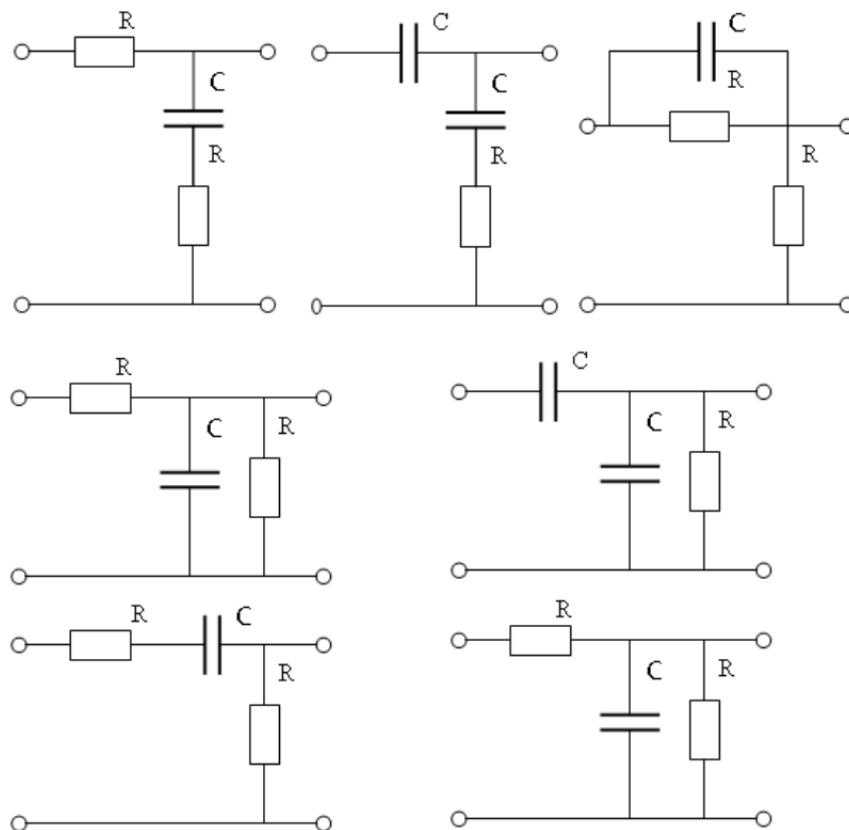
Рисунок 3 – Варианты схем линейной цепи к заданию 3
