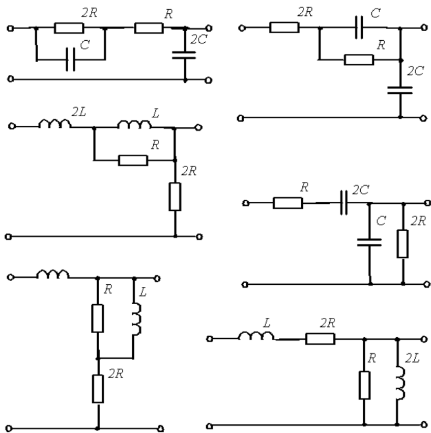
Рисунок 4 – Варианты схем линейной цепи к заданию 4
