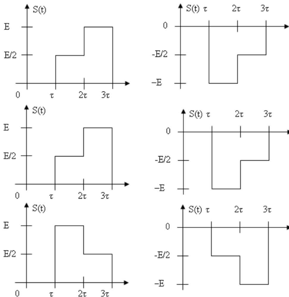
Рисунок 1 – Варианты временного представления сигналов к заданию 1
