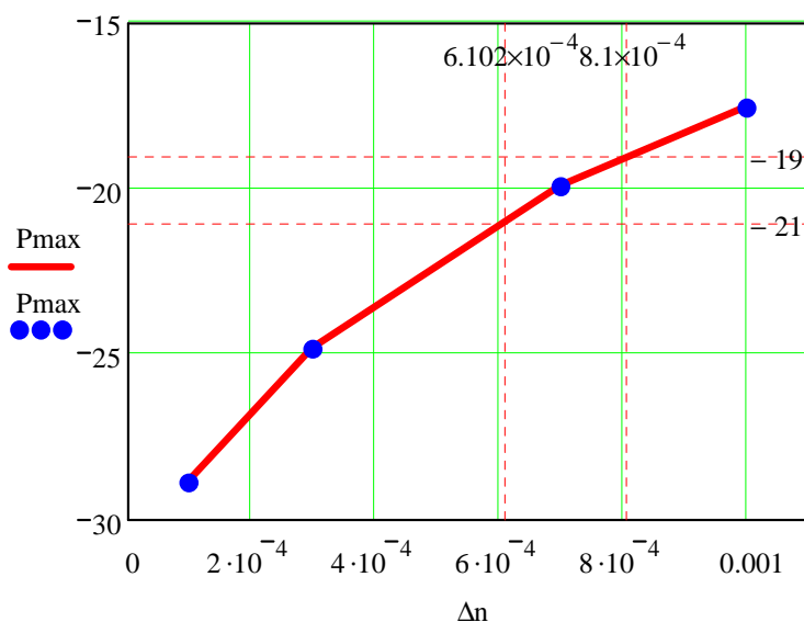
Рисунок 1.2 – График зависимости P_{\max}(\Delta n) .
