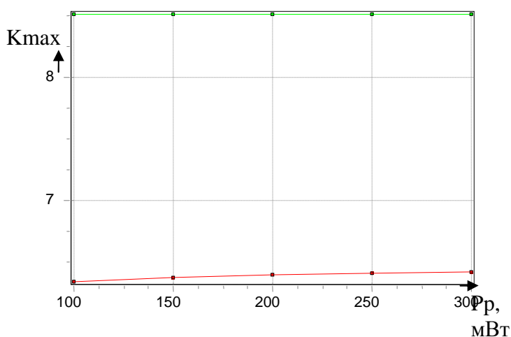
Рисунок 3.2.1 - Зависимость G_{\max}(P_p)
