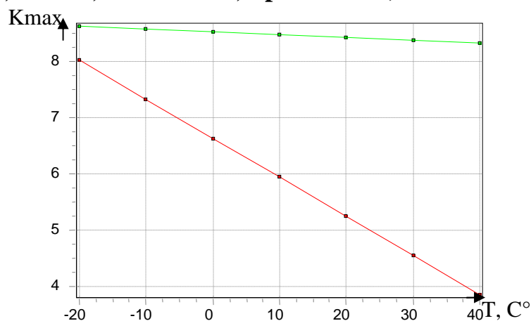
Рисунок 3.4.1 - Зависимость K_{max}(T)
