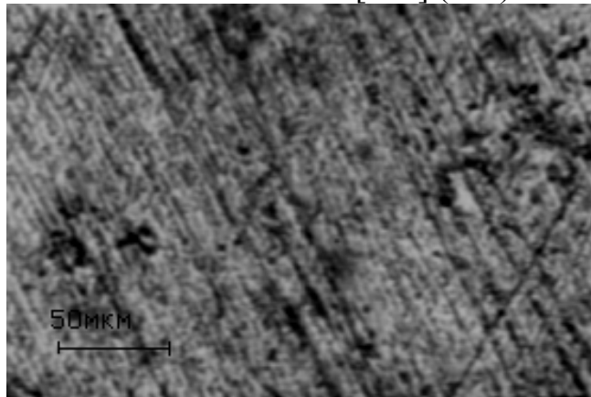
Рисунок 1.6 – Линии скольжения в германии, выращенном методом направленной кристаллизации
