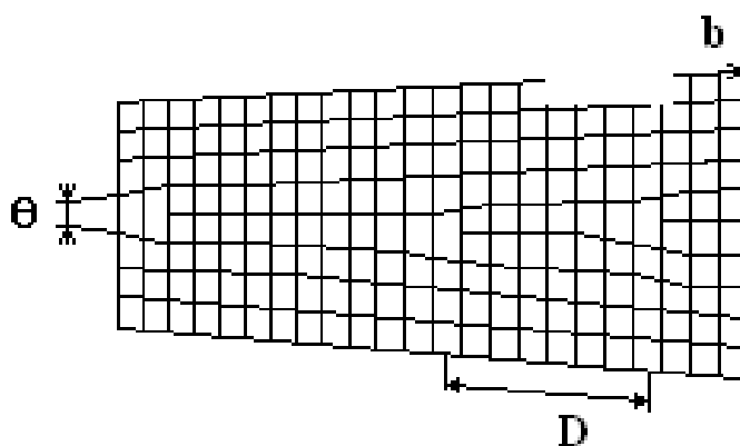
Рисунок 1.7 – Граница блоков с малым углом разориентации
