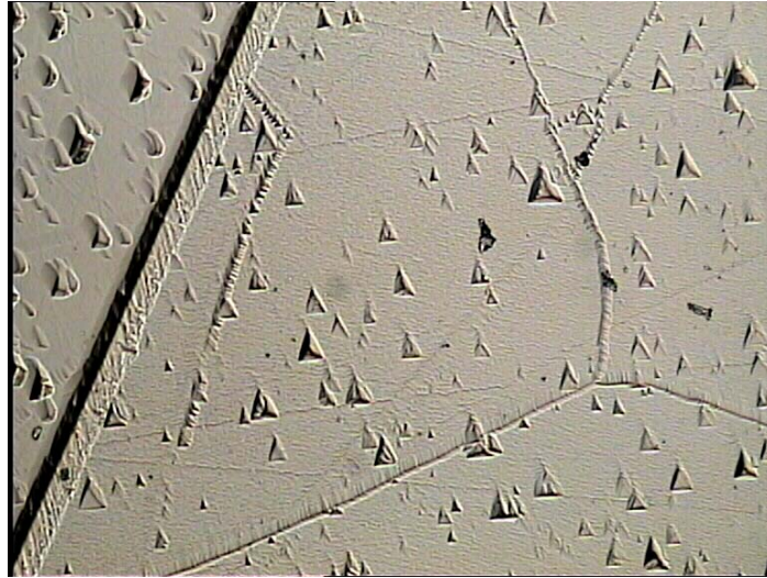
Рисунок 1.5 – Дислокационные ямки травления на поверхности флюорита, параллельной кристаллографической плоскости
