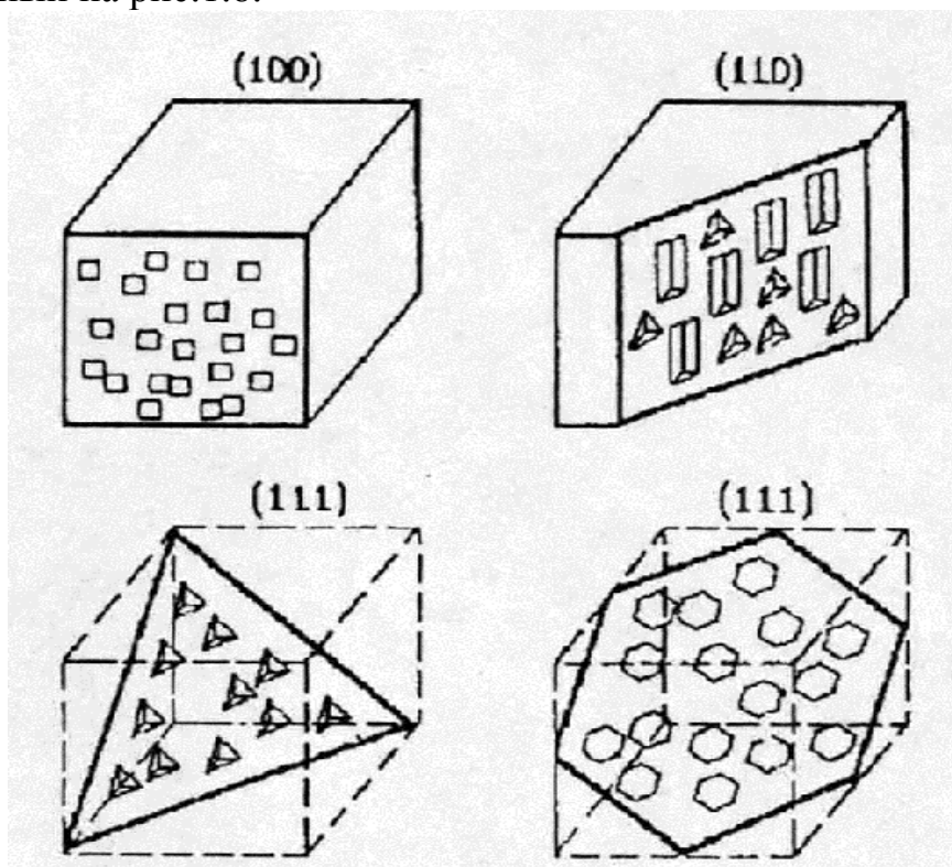
Рисунок 1.8 – Фигуры травления на основных кристаллографических плоскостях кубической решетки
