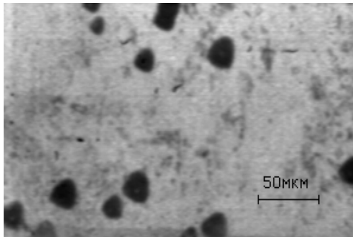
Рисунок 1.4 – Дислокационные ямки травления на поверхности германия, параллельной кристаллографической плоскости (111)
