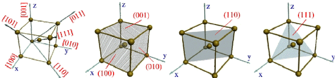
Рисунок 1.3 – Кристаллографические направления и плоскости в кристаллической решетке
