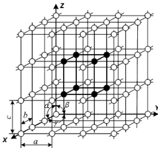
Рисунок 1.1 – Элементарная ячейка
