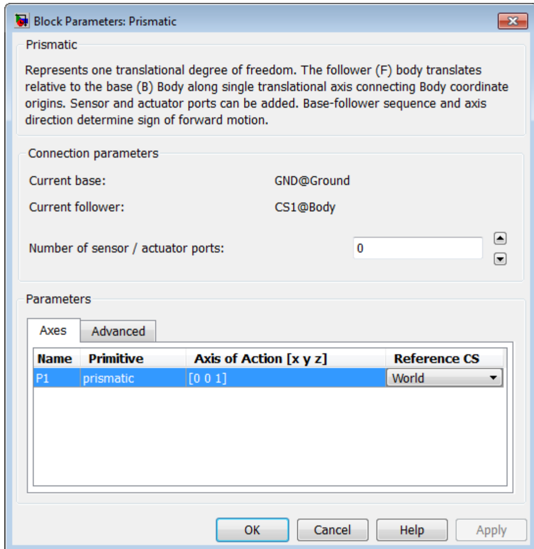
Рис. 11. Окно настройки подсоединенного блока Prismatic
