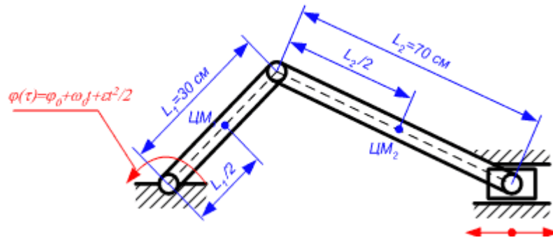
Рис. Кривошипно-шатунный механизм
