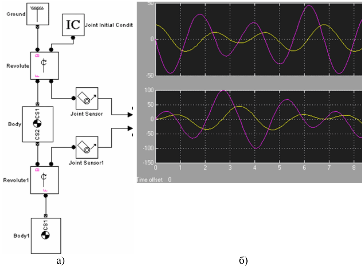
Рис. Модель двухзвенного физического маятника (а) для исследования законов движения его звеньев (б)
