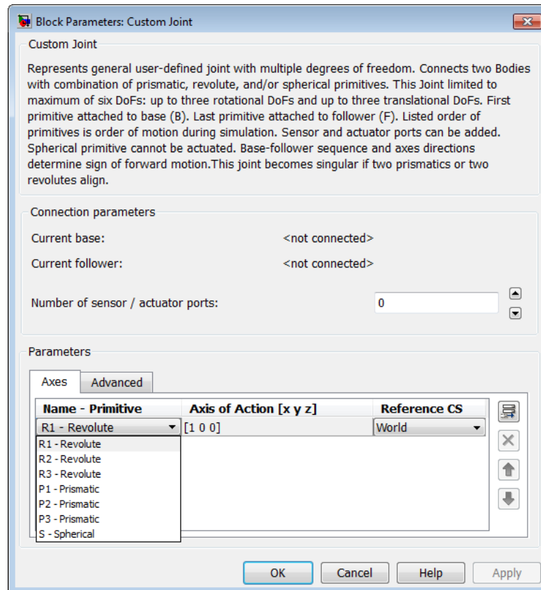
Рис. 14. Окно настройки блока CustomJoint
