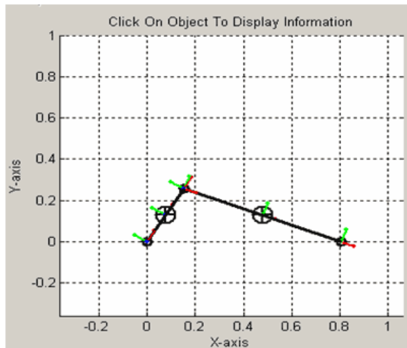
Рис. 9 Окончательная модель кривошипно-шатунного механизма
