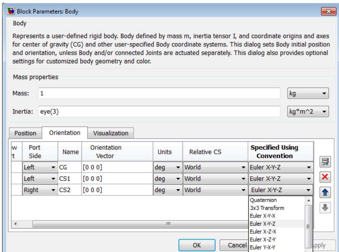
Рис. 7. Вкладка Ориентация окна настройки блока Body
