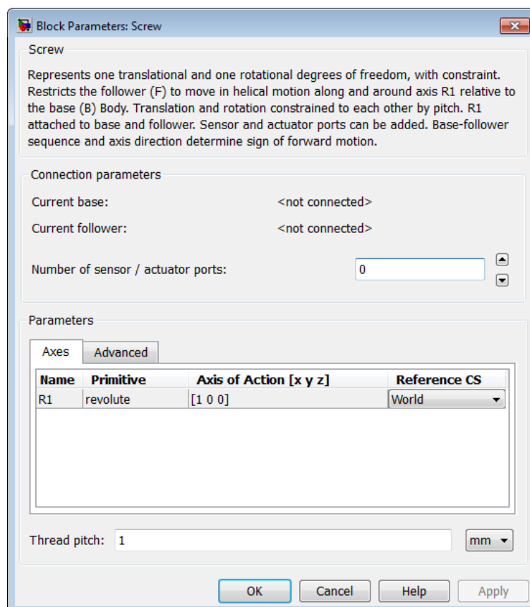
Рис. 15. ОкнонастройкиблокаScrew
