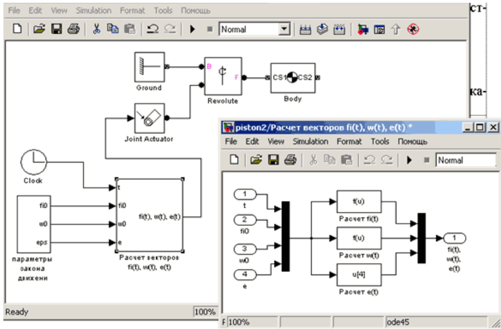
Рис. Добавление к модели привода и моделирование закона движения
