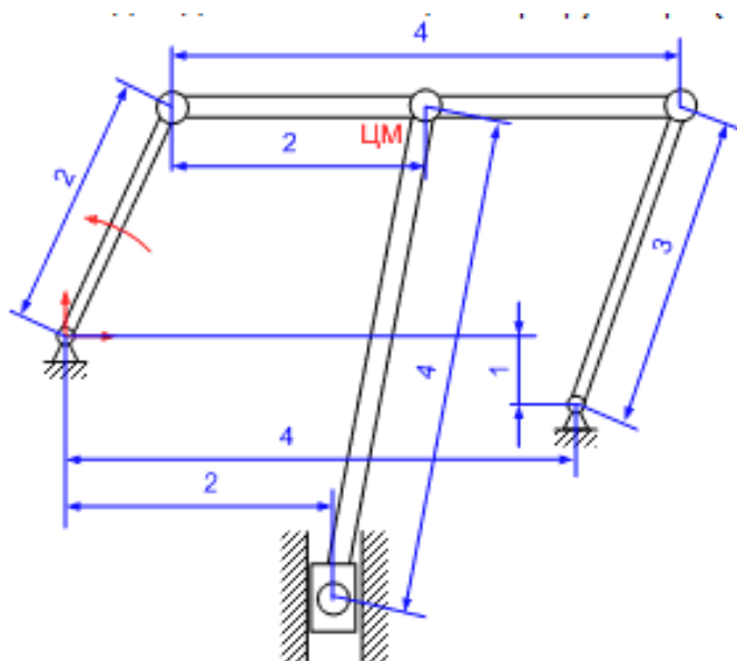
Рис. 10 - Механизм с одной степенью свободы
