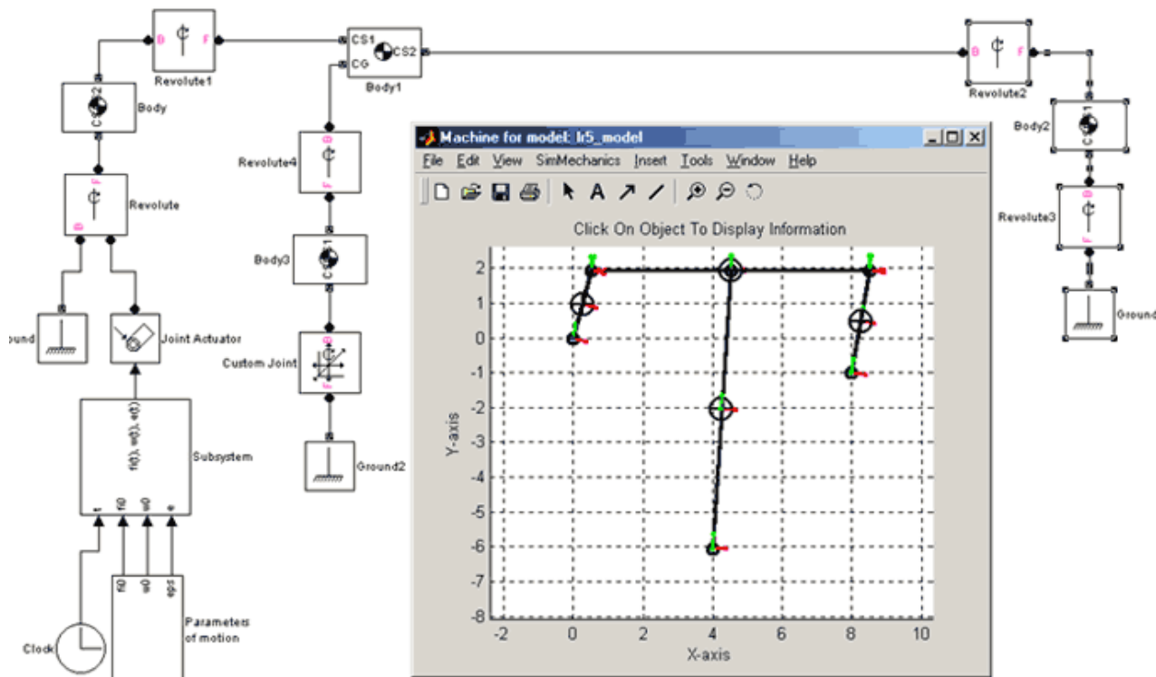
Рис. 11 - Вариант построения имитационной модели механизма, представленного на рис. 10
