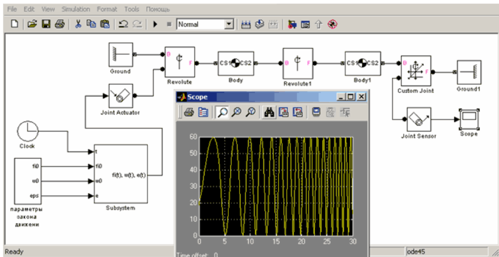
Рис. Добавление к модели привода и моделирование закона движения
