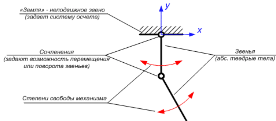
Рис. Модель двухзвенного физического маятника
