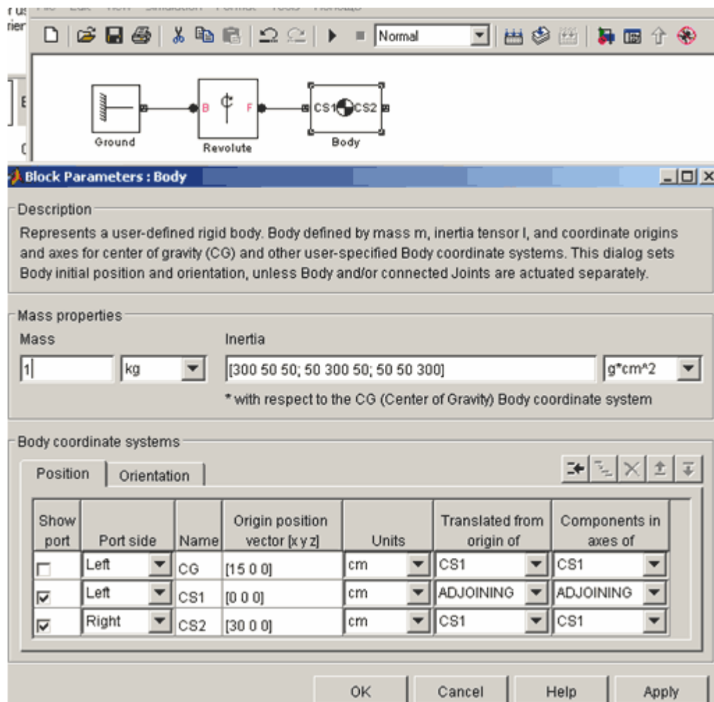
Рис. Параметры блока Body - при вводе данных о кривошипном звене
