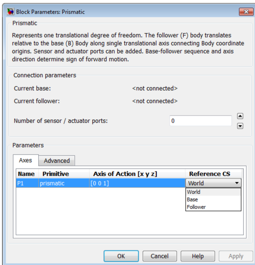
Рис. 9. Окно настройки блока Prismatic
