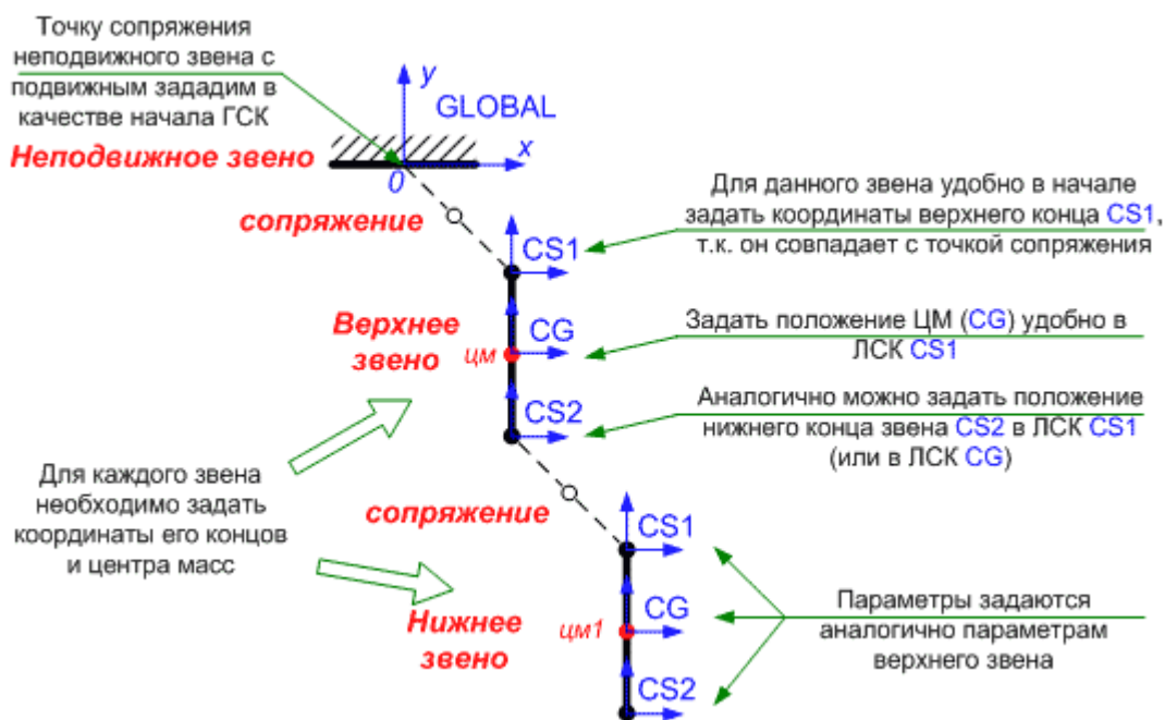
Рис. Системы координат двухзвенного физического маятника
