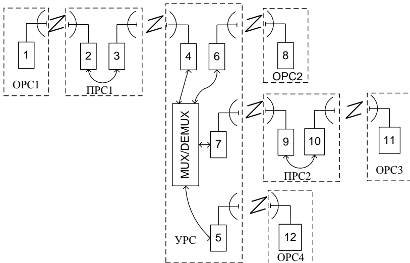
Рисунок 3.1 – Организация сети
