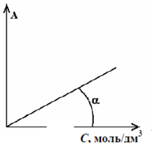
Рис. 1.4 Зависимость поглощения от концентрации раствора
