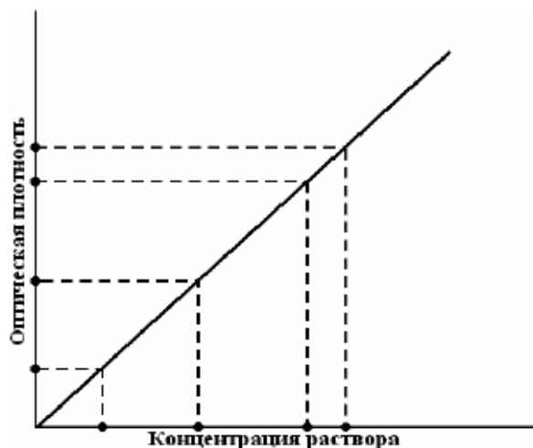
Рис. 1.2 Зависимость оптической плотности от концентрации раствора
