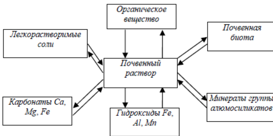
Рис. 2.1 Почвенный раствор
