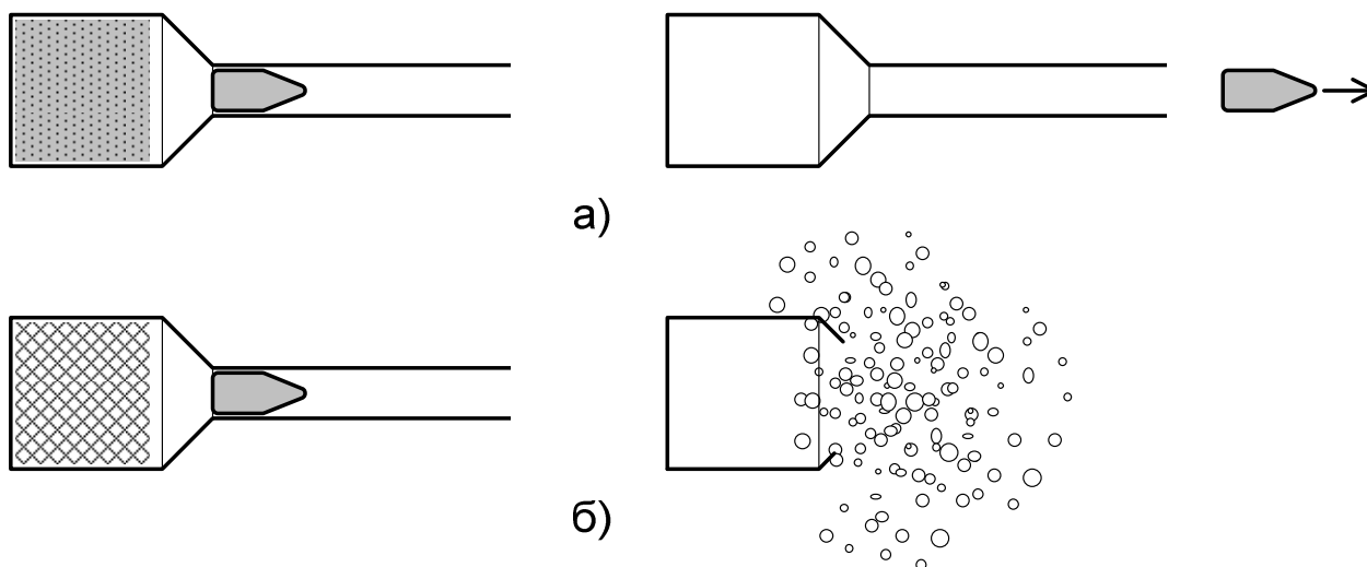
Рис. 6.2. Схема действия взрывчатого вещества на снаряд при горении: а – пороха; б – бризантного взрывчатого вещества
