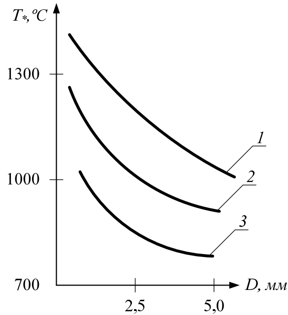
Рис. 2.2. Зависимость температуры самовоспламенения газов от диаметра нагретого шарика: 1 – пентан, 2 – светильный газ, 3 – водород
