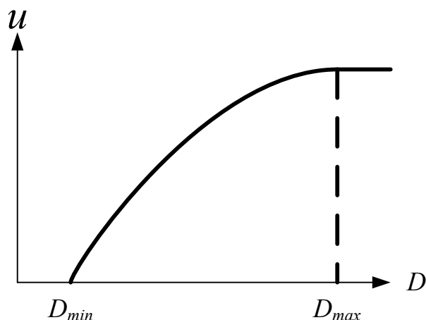
Рис. 3.8. Зависимость скорости распространения пламени от диаметра трубки
