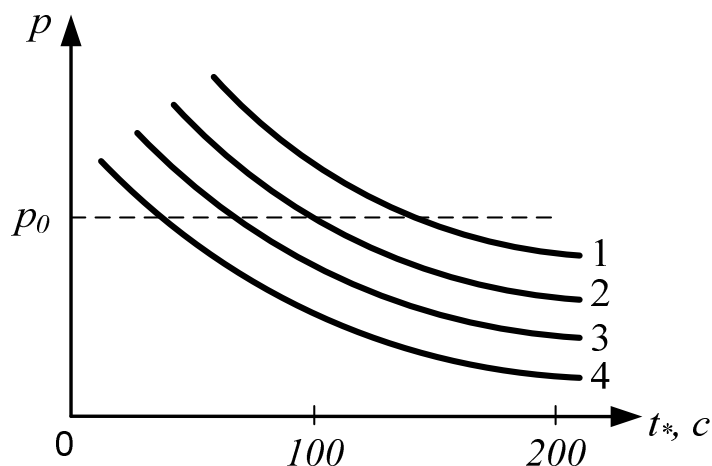
Рис. 2.6. Влияние температуры на величину периода индукции смеси ( \text{CH}_4 + \text{O}_2 ): 1 – T = 730^\circ\text{C} ; 2 – T = 750^\circ\text{C} ; 3 – T = 780^\circ\text{C} ; 4 – T = 800^\circ\text{C}
