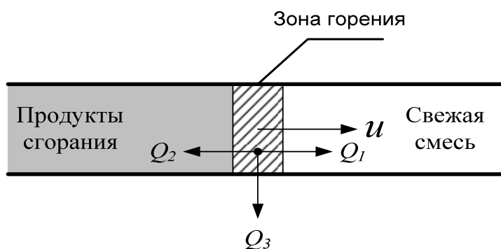
Рис. 3.9. Схема теплоотвода из зоны горения
