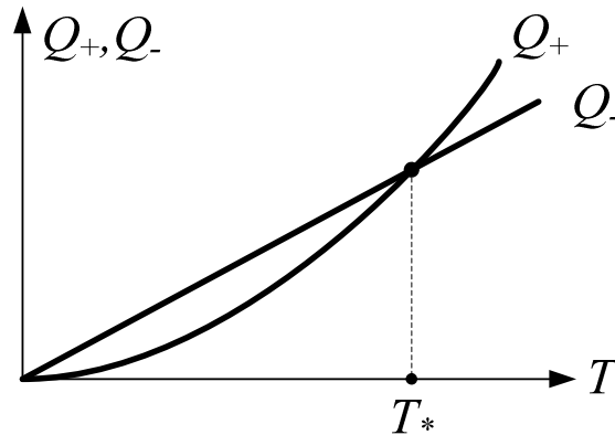
Рис. 2.1. Диаграмма Семенова
