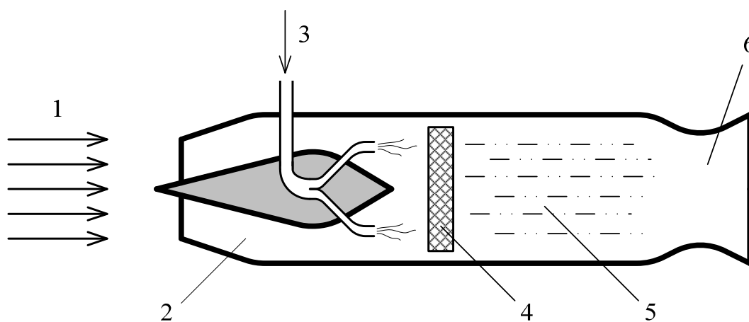
Рис. 1.1. Схема проточного воздушно-реактивного двигателя: 1 – воздух; 2 – диффузор; 3 – впрыск горючего; 4 – стабилизатор пламени; 5 – камера сгорания; 6 – сопло
