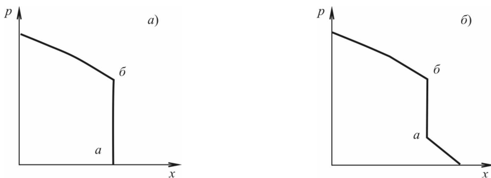
Рис. 3.17. Схема развития детонации в разные моменты времени
