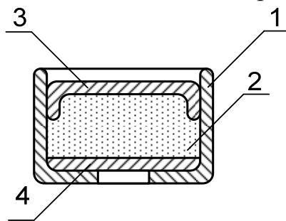
Рис. 6.4. Схема трубчатого капсюля-воспламенителя: 1 – колпачок с отверстием; 2 – ударный состав; 3 – фольговая чашечка; 4 – фольговая диафрагма
