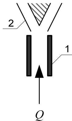
Рис. 3.4. Схема измерения нормальной скорости распространения пламени:
