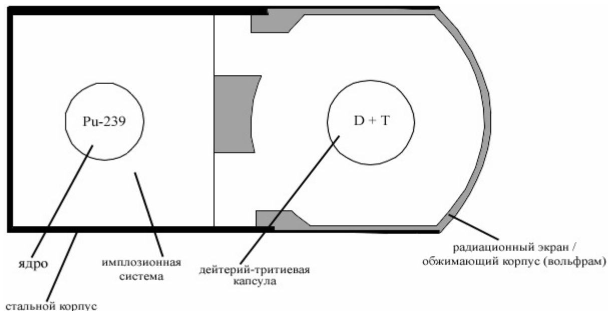
рис. 1 Примерная структура нейтронного заряда
