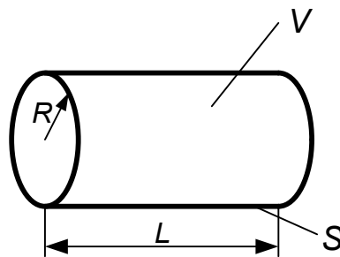
Рис. 3.10. Схема теплоотвода из цилиндрической трубки
