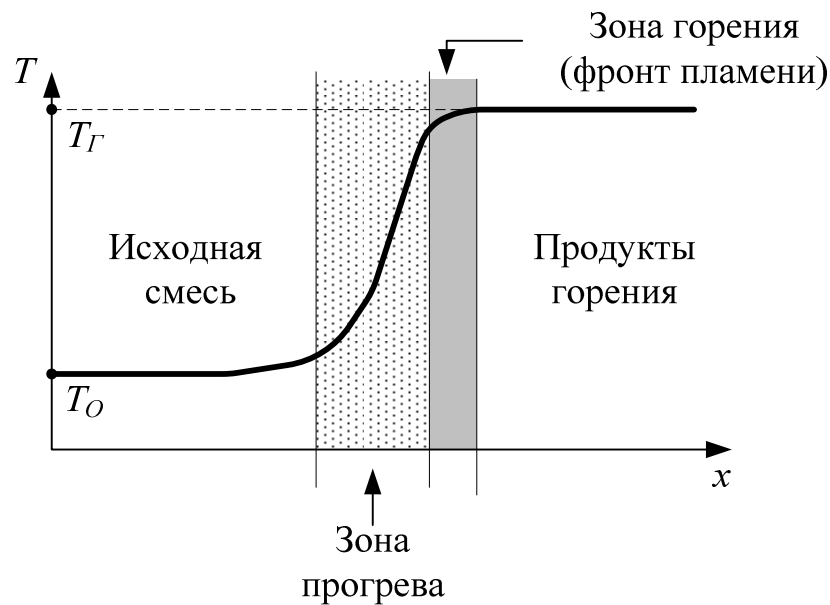
Рис. 9.1. Схема фронта пламени пылевоздушной смеси
