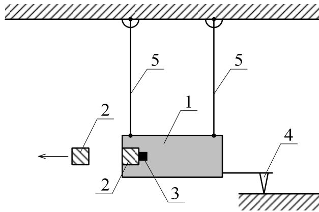
Рис. 7.4. Схема баллистической мортиры: 1-мортира, 2-снаряд, 3-заряд взрывчатого вещества, 4-измеритель отклонения, 5-подвес
