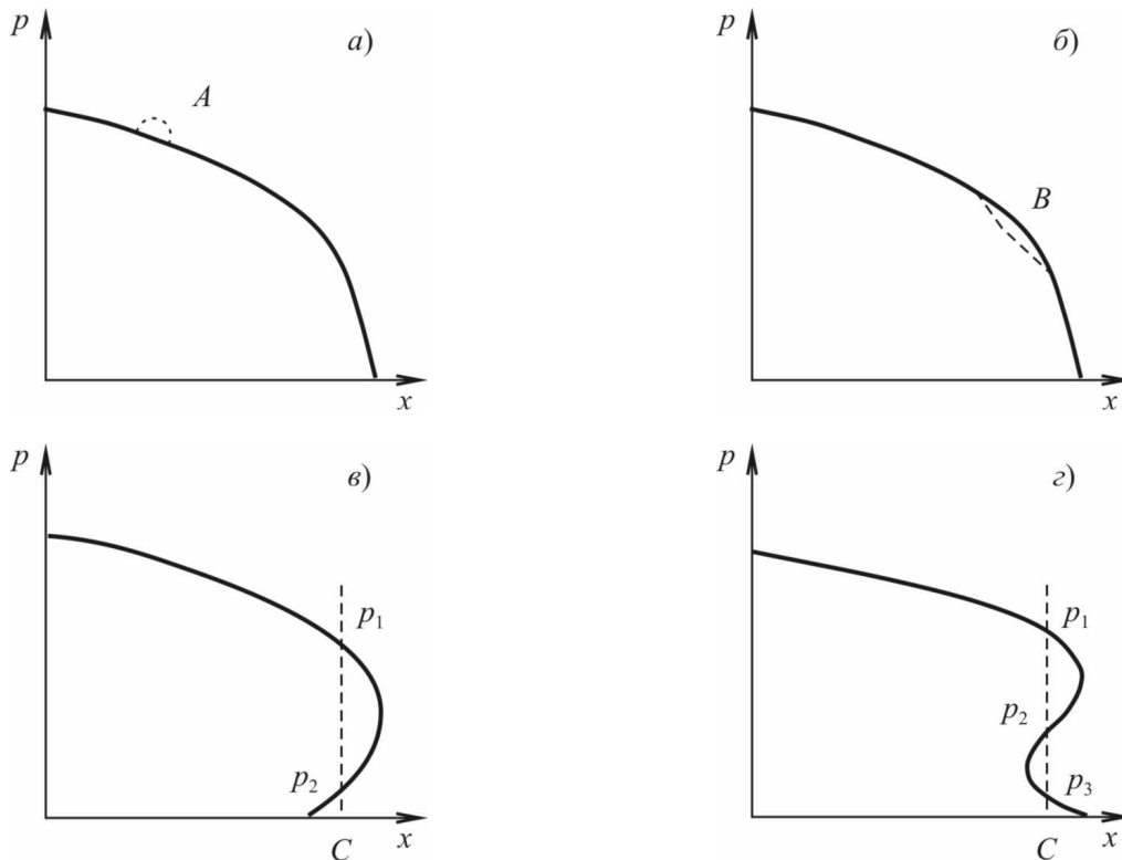
Рис. 3.15. Схема развития детонации
