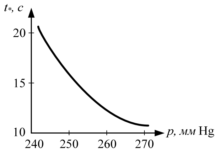
Рис. 2.5. Влияние давления на величину периода индукции смеси ( \text{CH}_3\text{OCH}_3 + \text{O}_2 ) при T = 245^\circ\text{C}
