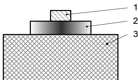
Рис. 6.1. Схема детонации бризантного взрывчатого вещества: 1 – капсюль (иницирующее взрывчатое вещество); 2 – детонатор; 3 – основной заряд бризантного взрывчатого вещества
