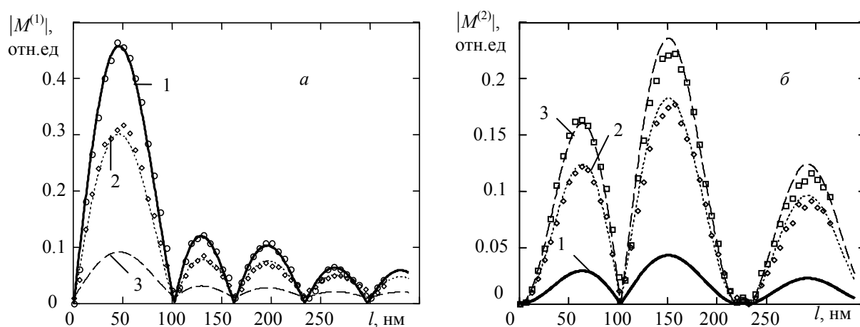
Рисунок 3.1 - Примеры амплитудных характеристик адаптивного голографического интерферометра:
