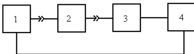
Рис.3.2. Структурная схема для измерения амплитудно-частотных характеристик (АЧХ) ЛЗ.
