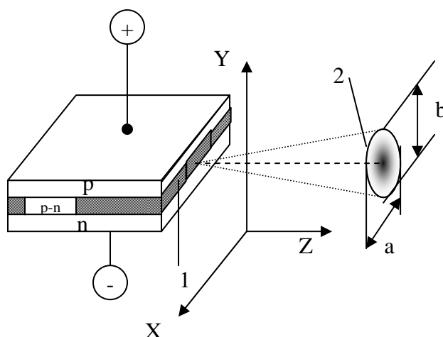
Рис. 2. Принципиальная схема лазера на p-n-переходе. 1 – область p-n перехода (активный слой); 2 – сечение лазерного пучка в плоскости X-Y.
