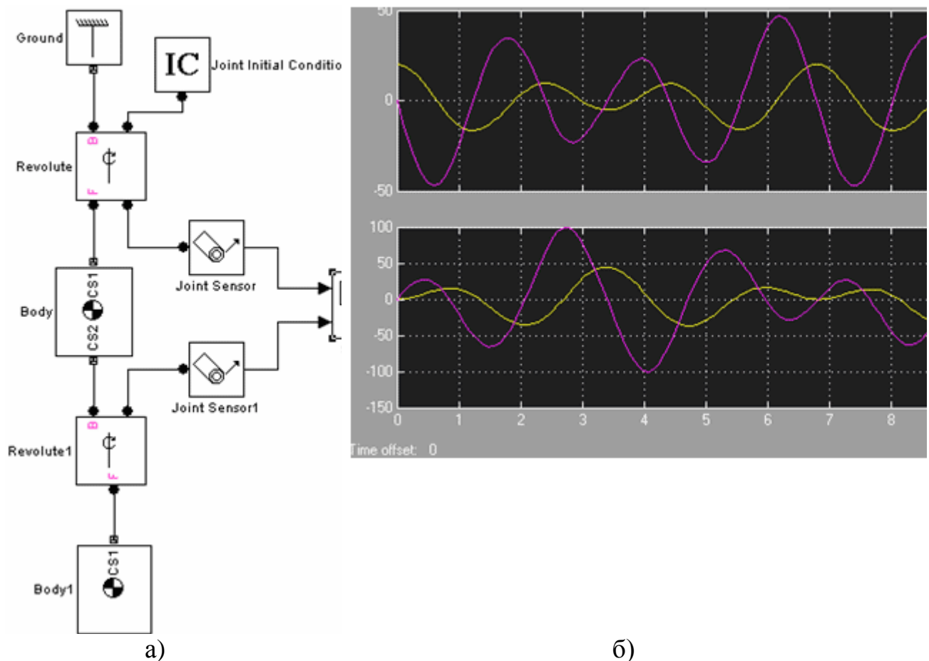
Рис. 22. Модель двухзвенного физического маятника (а) для исследования законов движения его звеньев (б)
