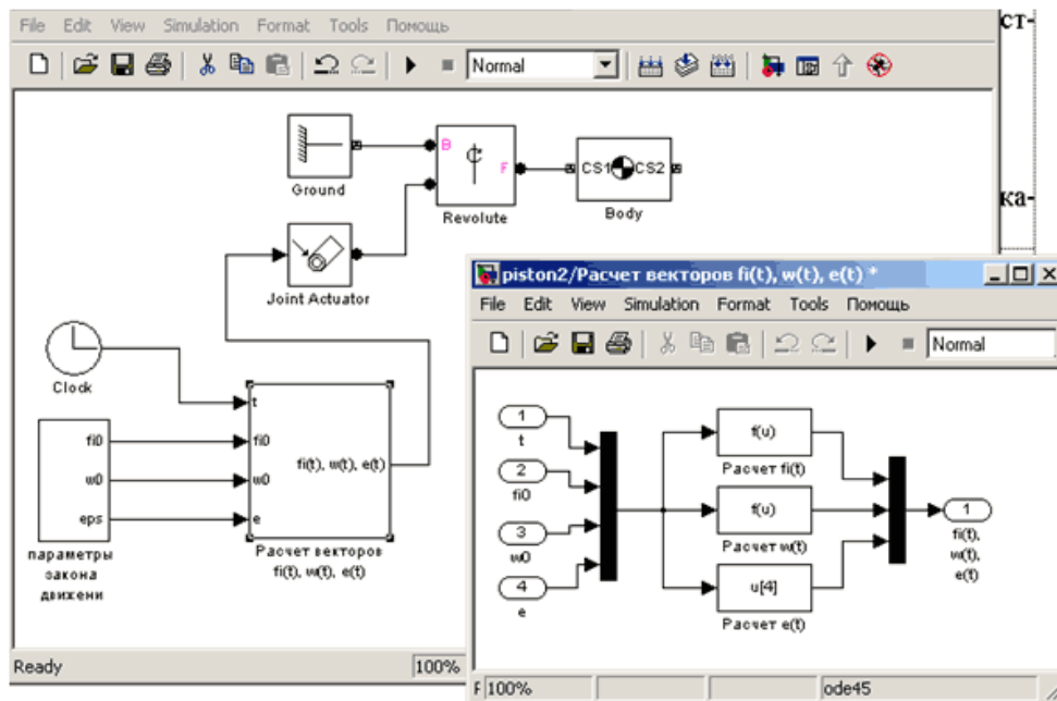
Рис. 26. Добавление к модели привода и моделирование закона движения
