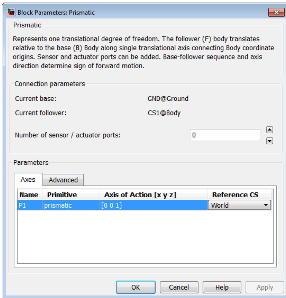
Рис. 11. Окно настройки подсоединенного блока Prismatic
