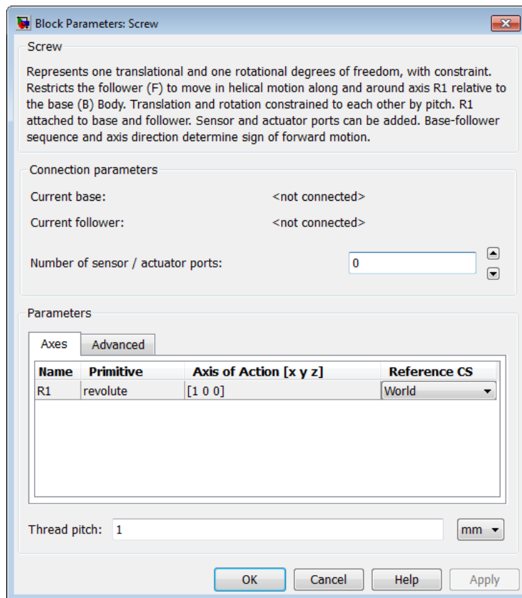
Рис. 15. Окно настройки блока Screw
