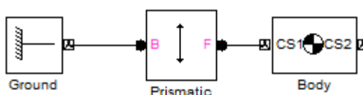
Рис. 10. Простейшая механическая цепь
