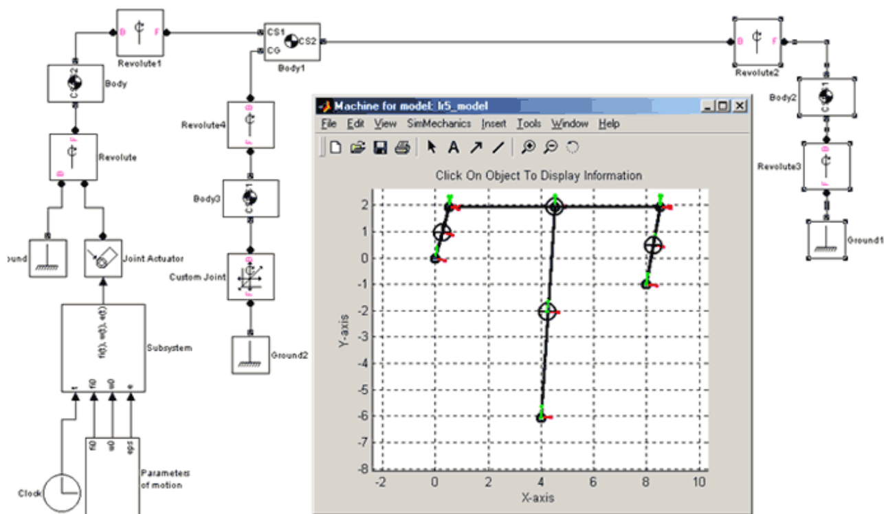
Рис. 29. Вариант построения имитационной модели механизма, представленного на рис. 28
