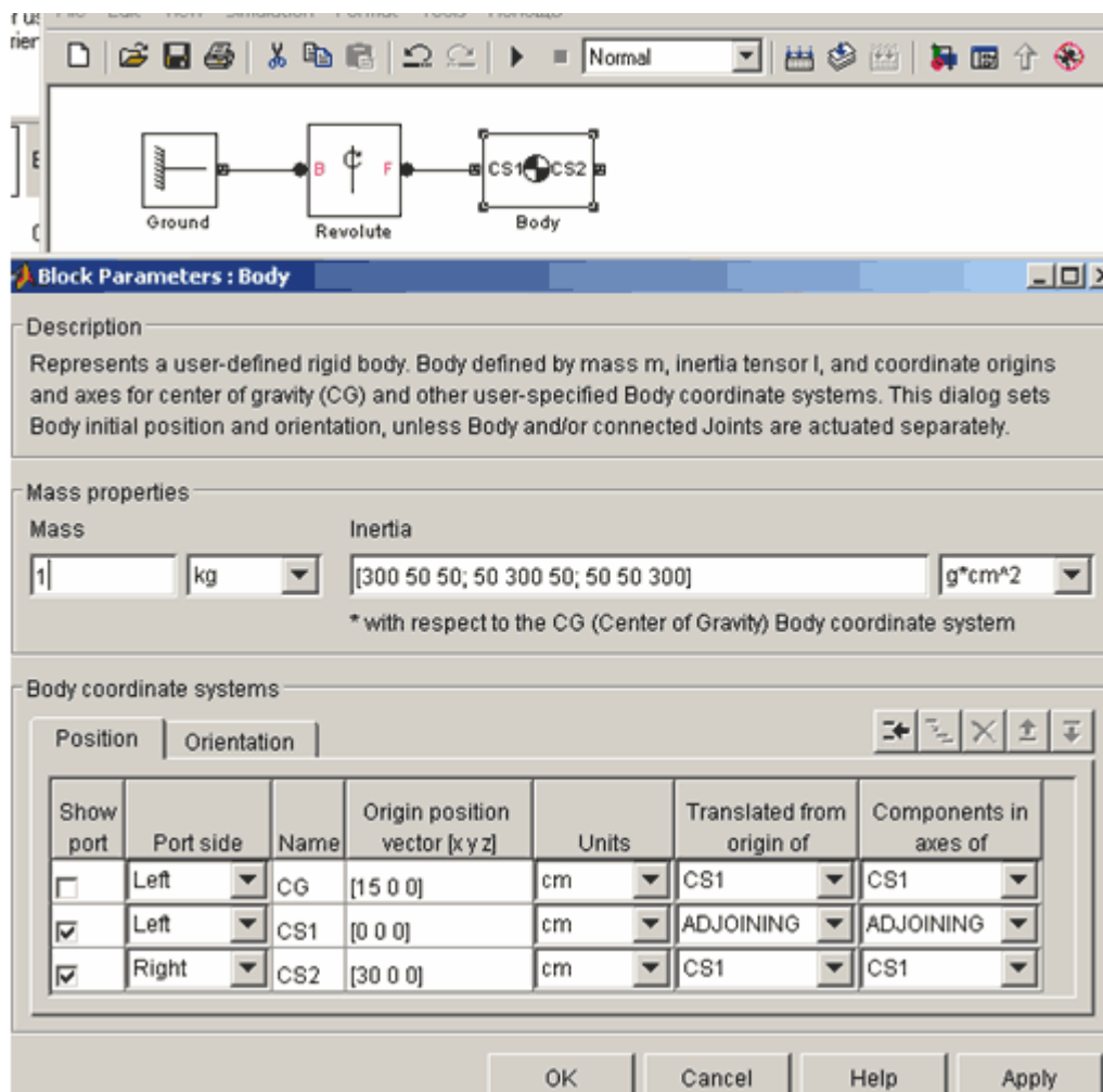
Рис. 25. Параметры блока Body – при вводе данных о кривошипном звене
