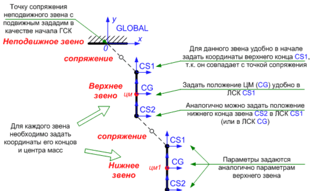
Рис. 21. Системы координат двухзвенного физического маятника
