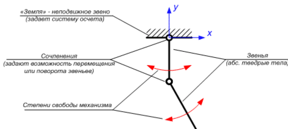
Рис. 19. Модель двухзвенного физического маятника
