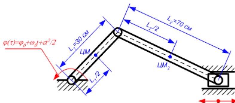
Рис. 24. Кривошипно-шатунный механизм
