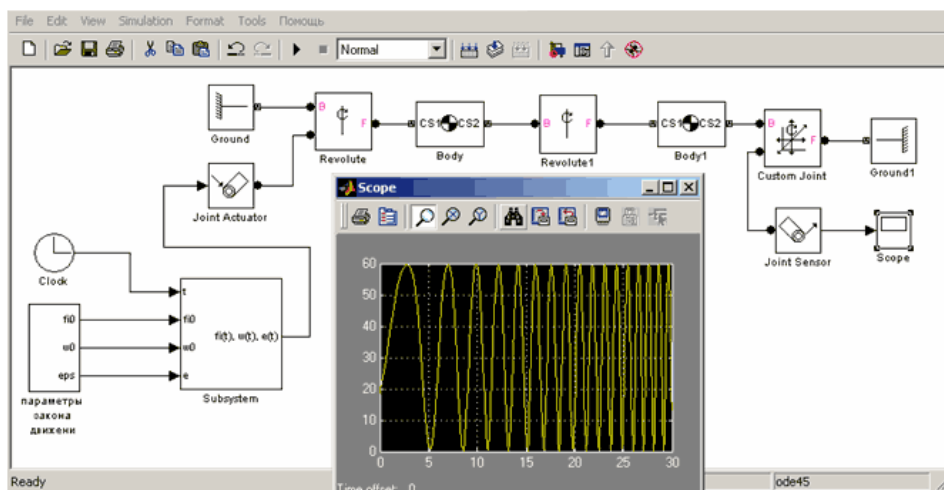
Рис. 26. Добавление к модели привода и моделирование закона движения
