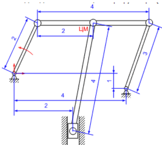
Рис. 28. Механизм с одной степенью свободы
