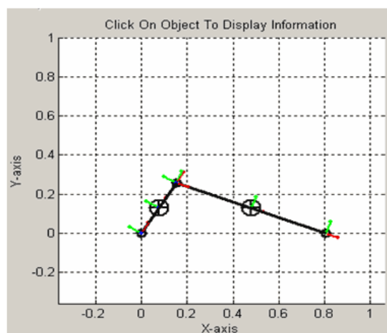
Рис. 27. Окончательная модель кривошипно-шатунного механизма
