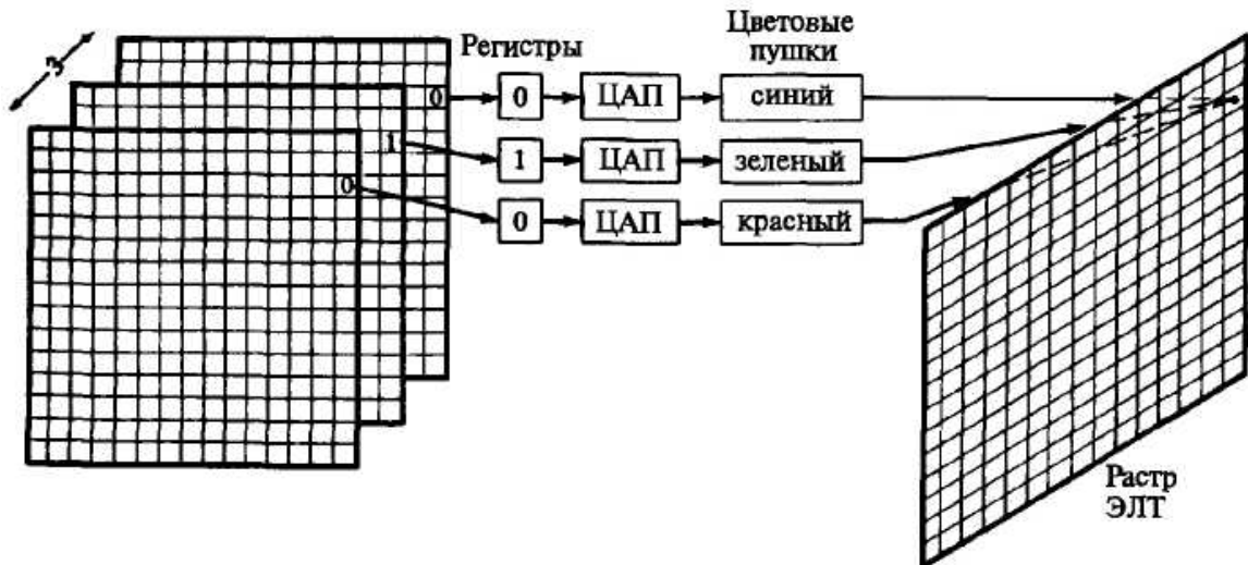
Рис. 16. Простой цветовой буфер кадра.
