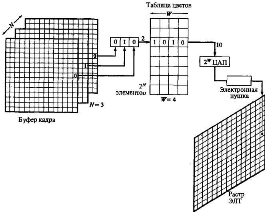
Рис. 15. Полутоновый черно-белый буфер кадра с N битовыми плоскостями и W -разрядной таблицей цветов.
