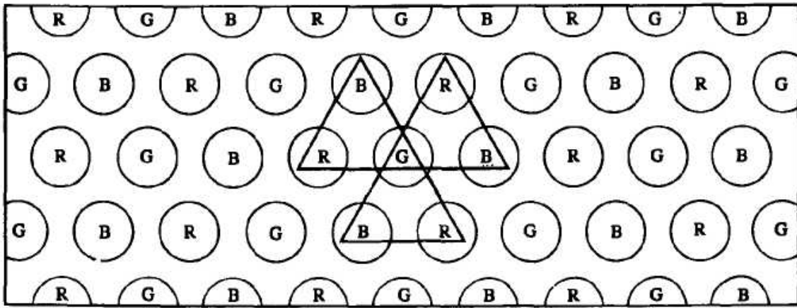
Рис. 19. Точечный люминофорный растр для ЭЛТ с теневой маской.
