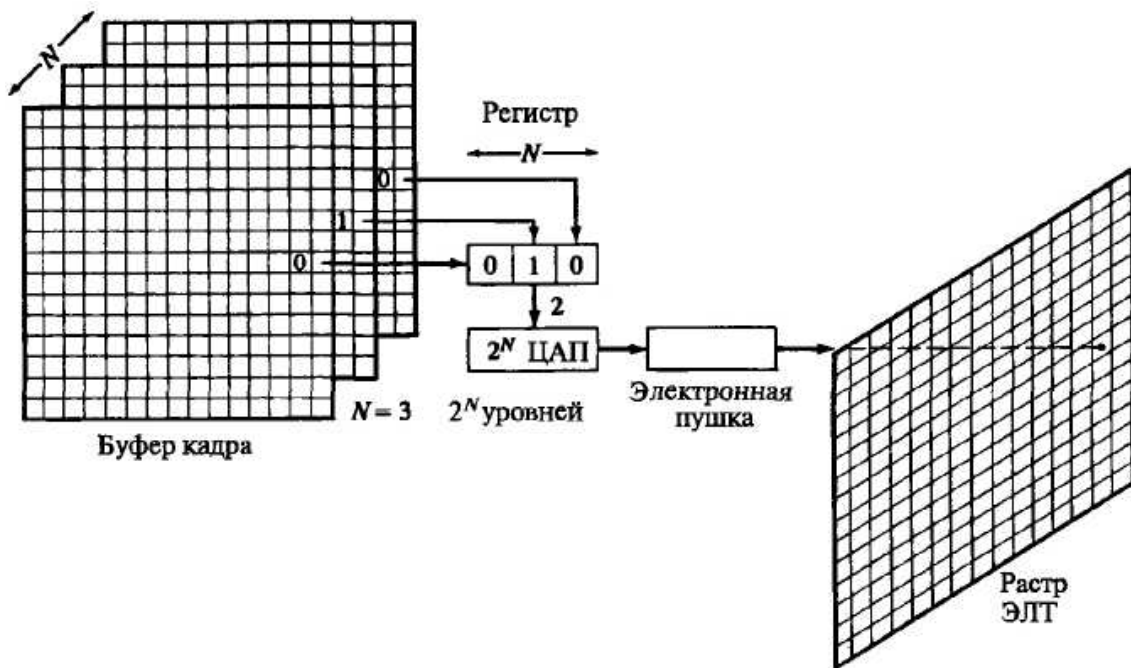
Рис. 14. Полутоновый черно-белый буфер кадра с N битовыми плоскостями.
