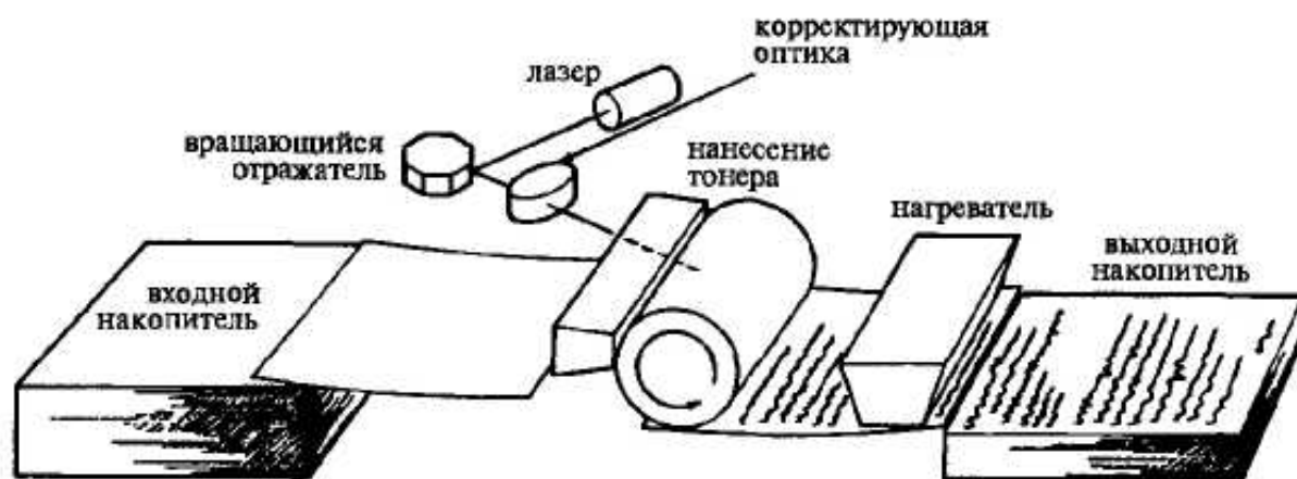
Рис. 23. Схема устройства лазерного принтера.
