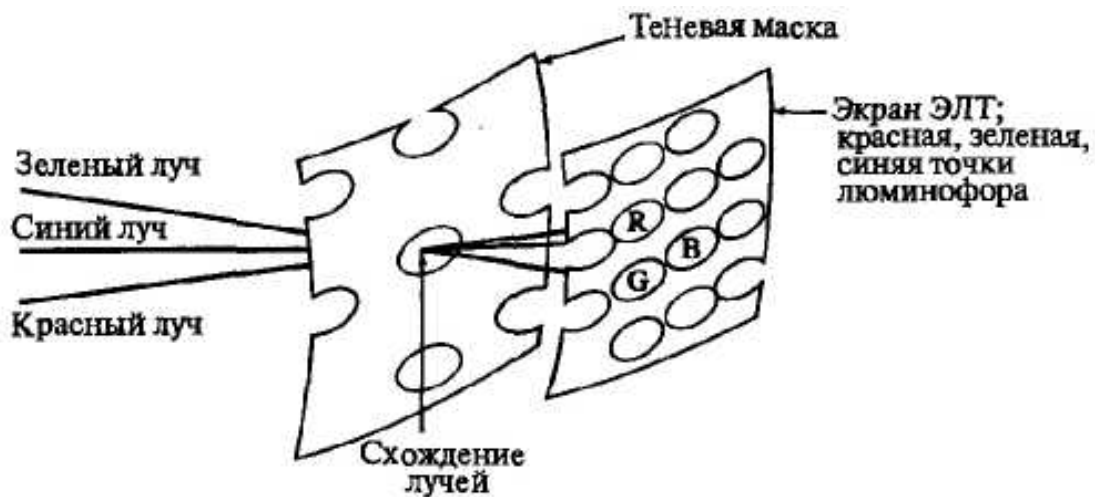
Рис. 20. Расположение электронной пушки и теневой маски цветной ЭЛТ.
