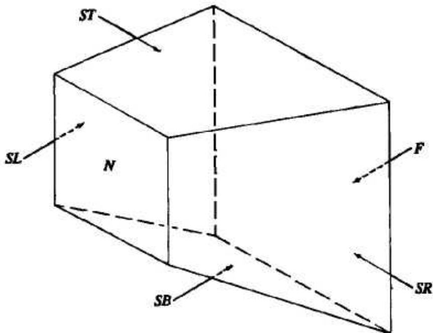
Рис. 3. Трехмерная пирамида видимости.
