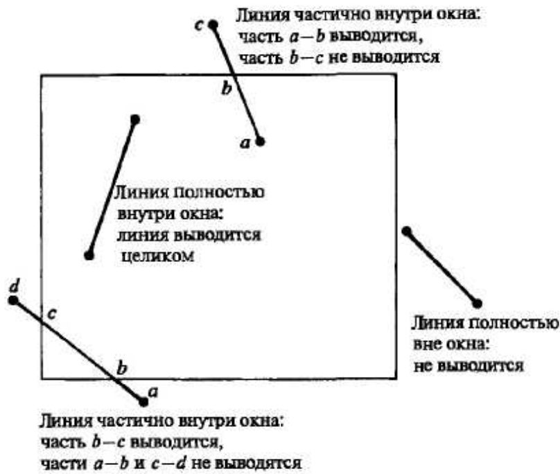
Рис. 2 Двумерное отсечение.
