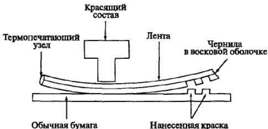
Рис. 27. Технология с косвенным тепловым воздействием.
