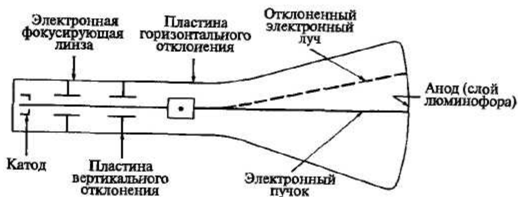
Рис. 18. Электронно-лучевая трубка.
