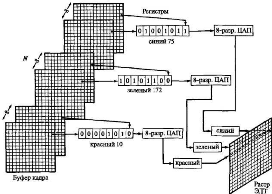
Рис. 17. Цветовой буфер кадра с 24 битовыми плоскостями.
