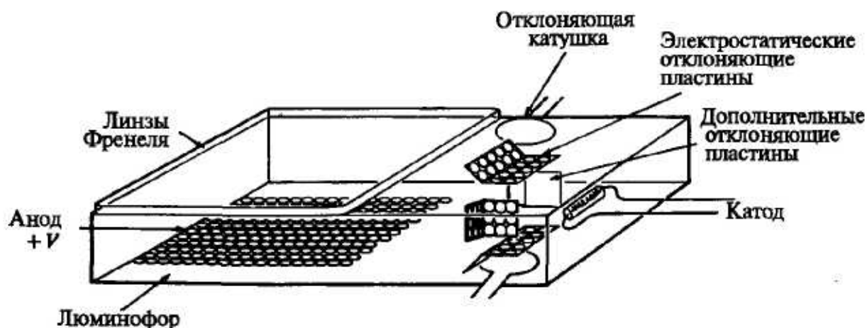
Рис. 21. Схема ЭЛТ.
