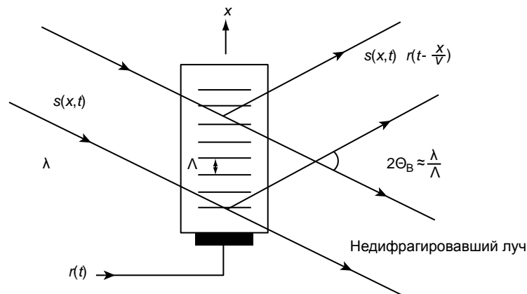
Схематическое изображение акустооптического модулятора
