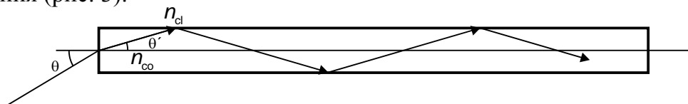
Рис. 3. Полное внутренне отражение света в оптоволоконне.
