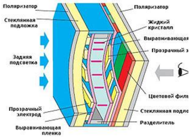
Рис. 9. Структура ячейки жидкокристаллического дисплея.
