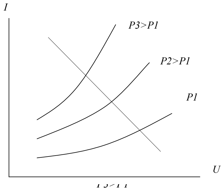
Рисунок 2.7 - Нагрузочная характеристика распыления материалов в разряде
