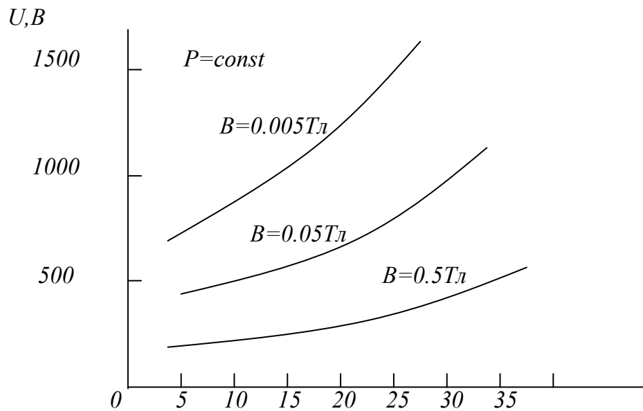
Рисунок 2.5 - Зависимость напряжения разряда от плотности тока для различной индукции магнитного поля
