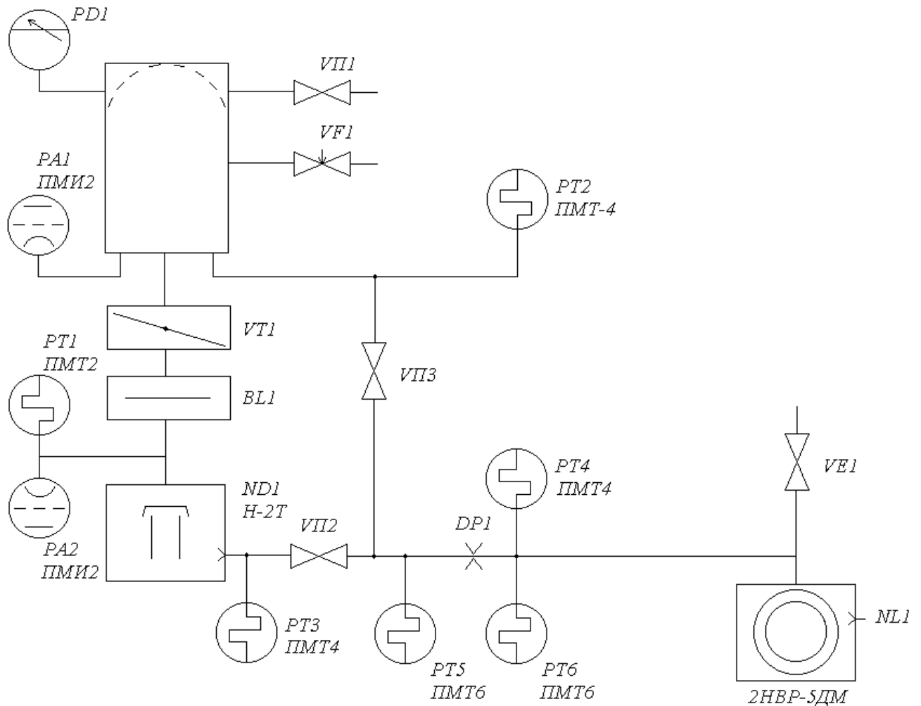
Рисунок 3.1 – Вакуумная схема установки УВН-2М
