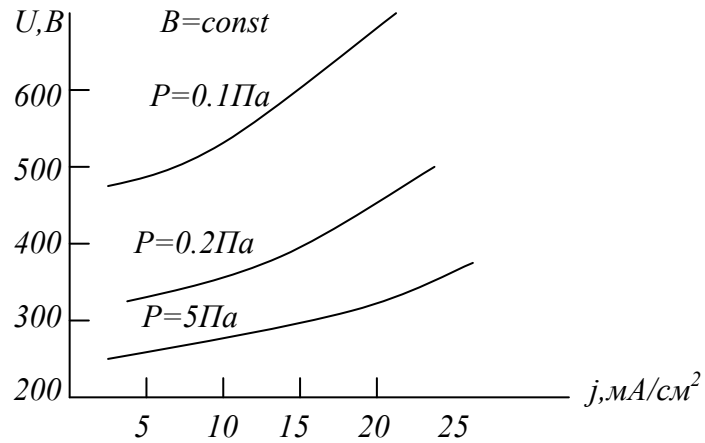
Рисунок 2.4 - Зависимость напряжения разряда от плотности тока для различных давлений
