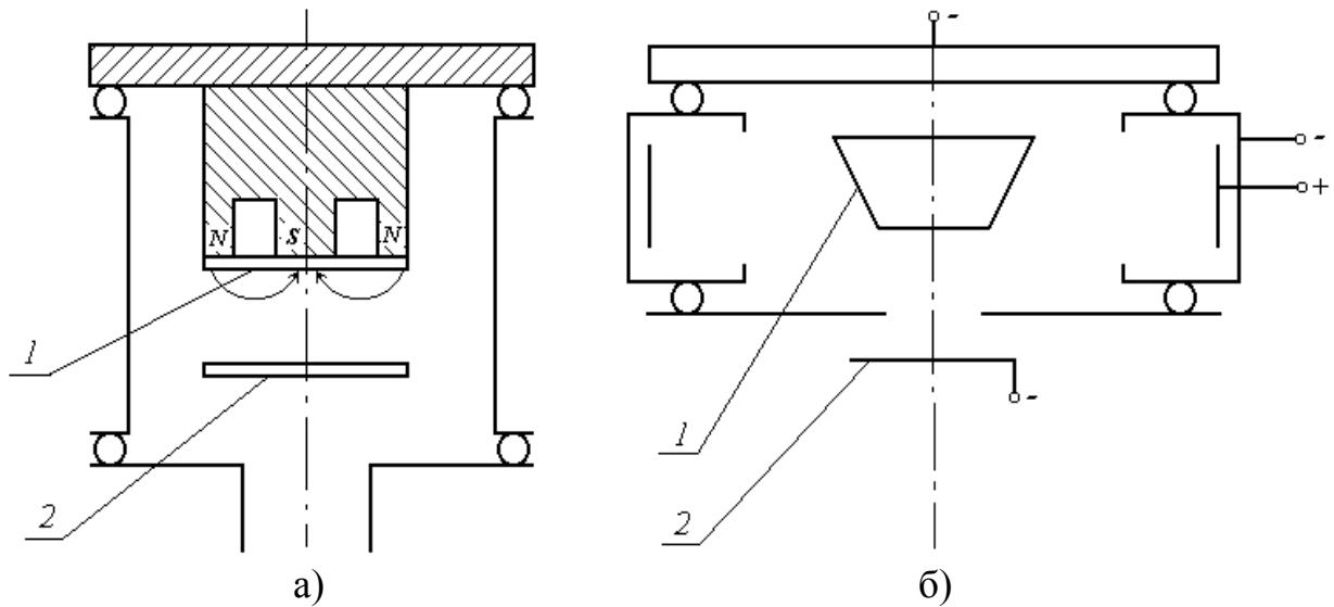
Рисунок 2.9 - Схемы магнетронных систем
