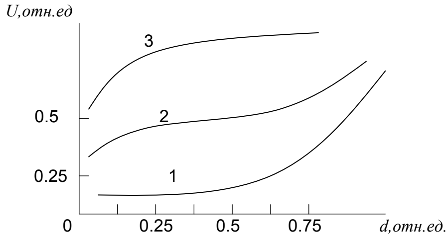
Распределение потенциала в магнетронной системе Рисунок 2.10 - Распределение потенциала в магнетронной системе
