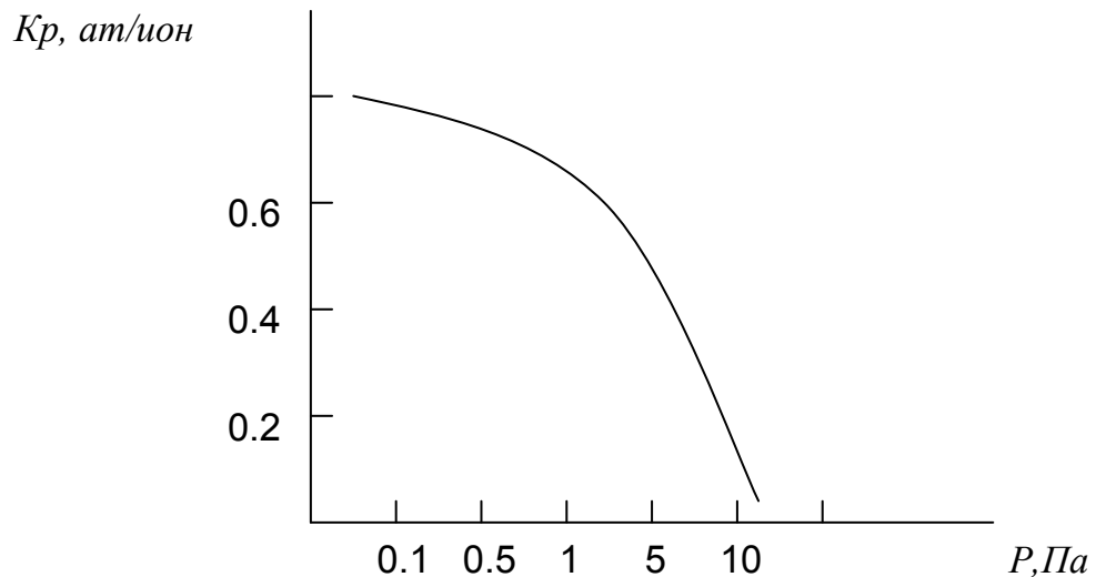
Рисунок 2.8 - Зависимость коэффициента распыления от давления
