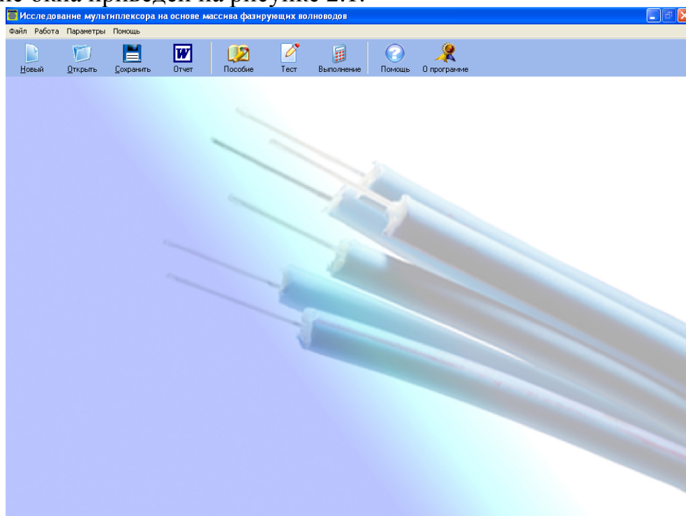
Рисунок 2.1 – Главное окно
