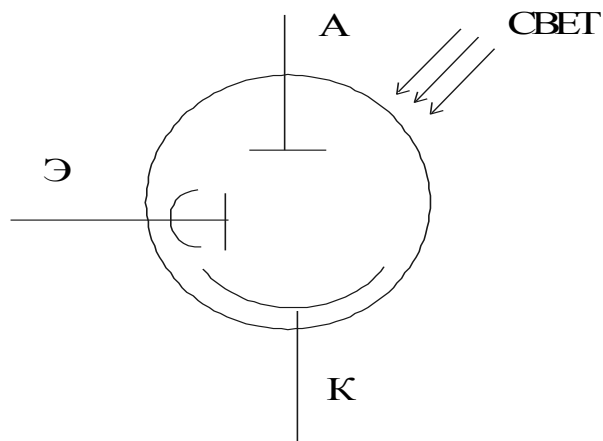
Рисунок 2.5 - Однокаскадный фотоумножитель
