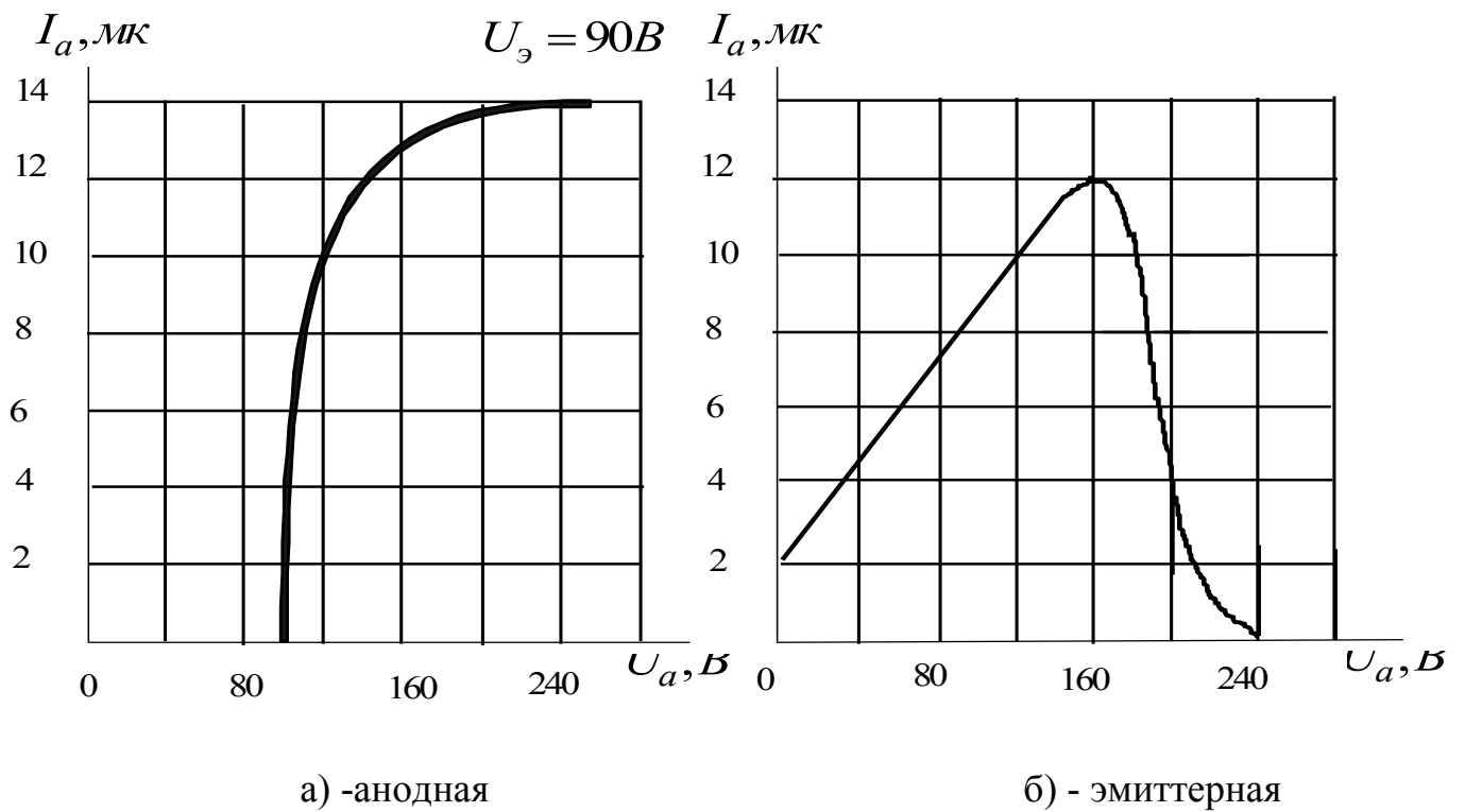
Рисунок 2.6 - Характеристики ФЭУ-1
