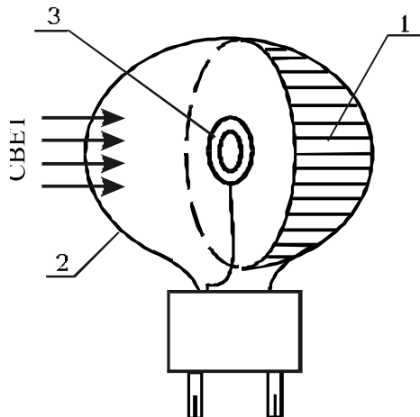
1 – фотокатод; 2 – баллон; 3 – анод
