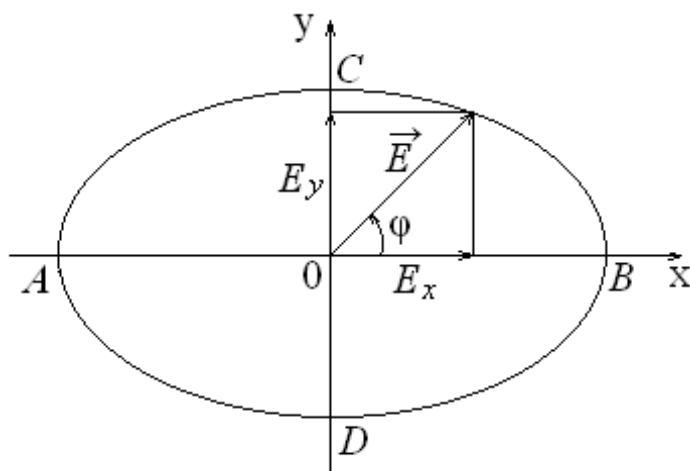
Рисунок 4 – Эллипс поляризации
