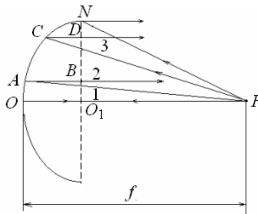
Рисунок 2 – Ход лучей в параболической антенне (фазовый центр облучателя совмещён с фокусом зеркала)
