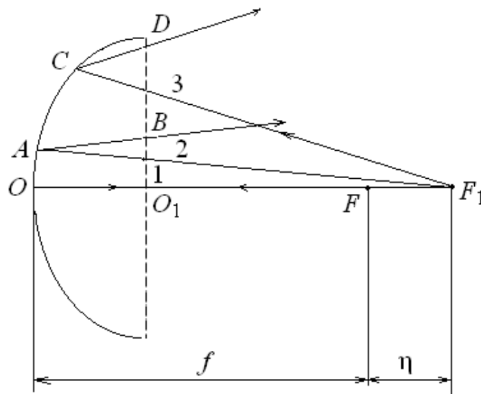
Рисунок 3 – Ход лучей в параболической антенне при вынесенном из фокуса облучателе
