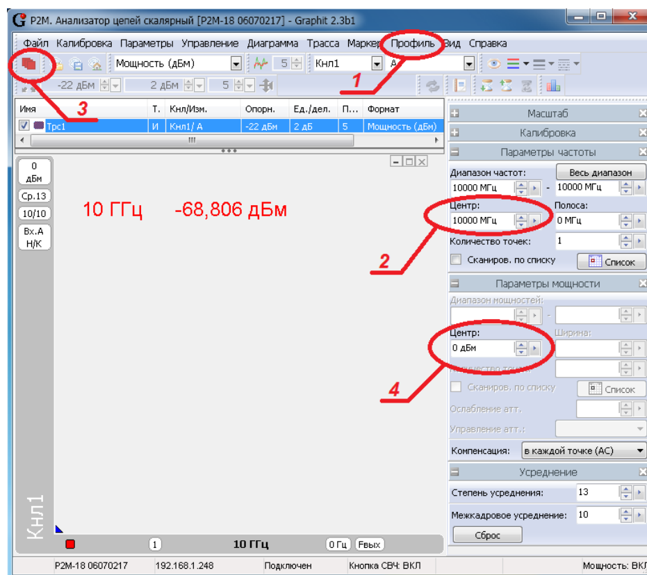
Рисунок 6. Окно программы Graphit
