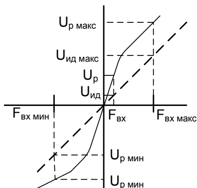
Рис. 2.1. Идеальная и реальная характеристики измерительного устройства.
