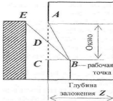
Рисунок 4.1 - Схема для определения основных характеристик освещенности (характерный разрез помещения)
