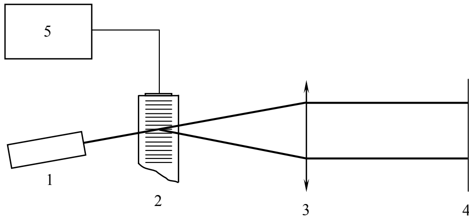
Рисунок 3.2 - Схема эксперимента 1 – лазер, 2 – АОМ, 3 – линза, 4 – экран, 5 – генератор сигналов,
