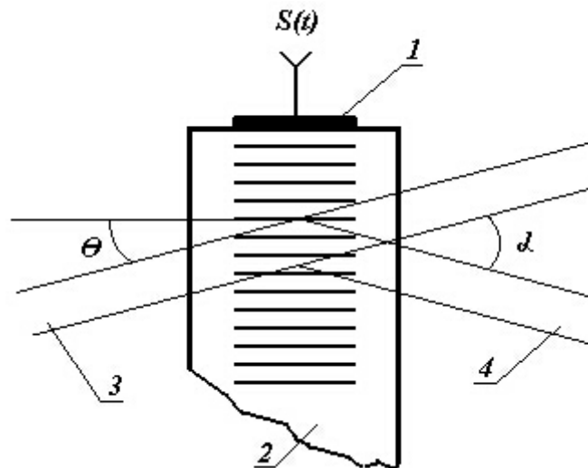
Рисунок 2.1 - Акустооптический модулятор
