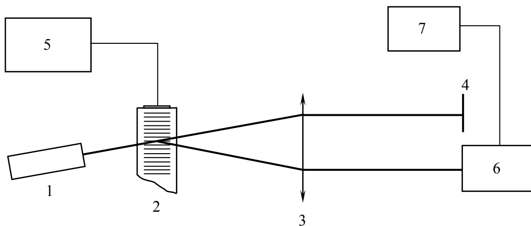
Рисунок 3.1 - Схема эксперимента
