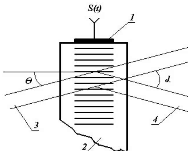
Рисунок 2.1 - Акустооптический модулятор
