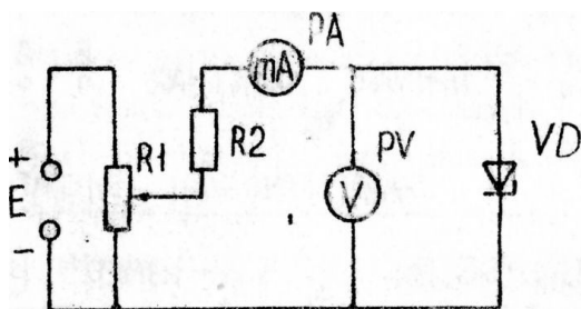
Рисунок 3.2 - Схема для снятия прямой характеристики прибора
