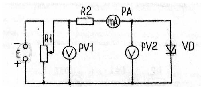
Рисунок 3.3 - Схема для снятия обратной характеристики
