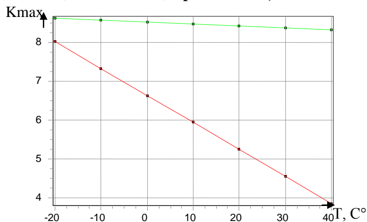
Рисунок 3.4.1 - Зависимость K_{\text{max}}(T)
