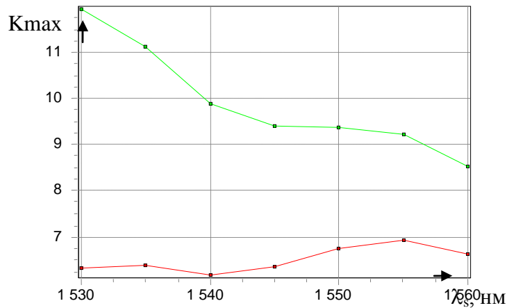
Рисунок 3.3.1 - Зависимость K_{\text{max}}(\lambda_s)
