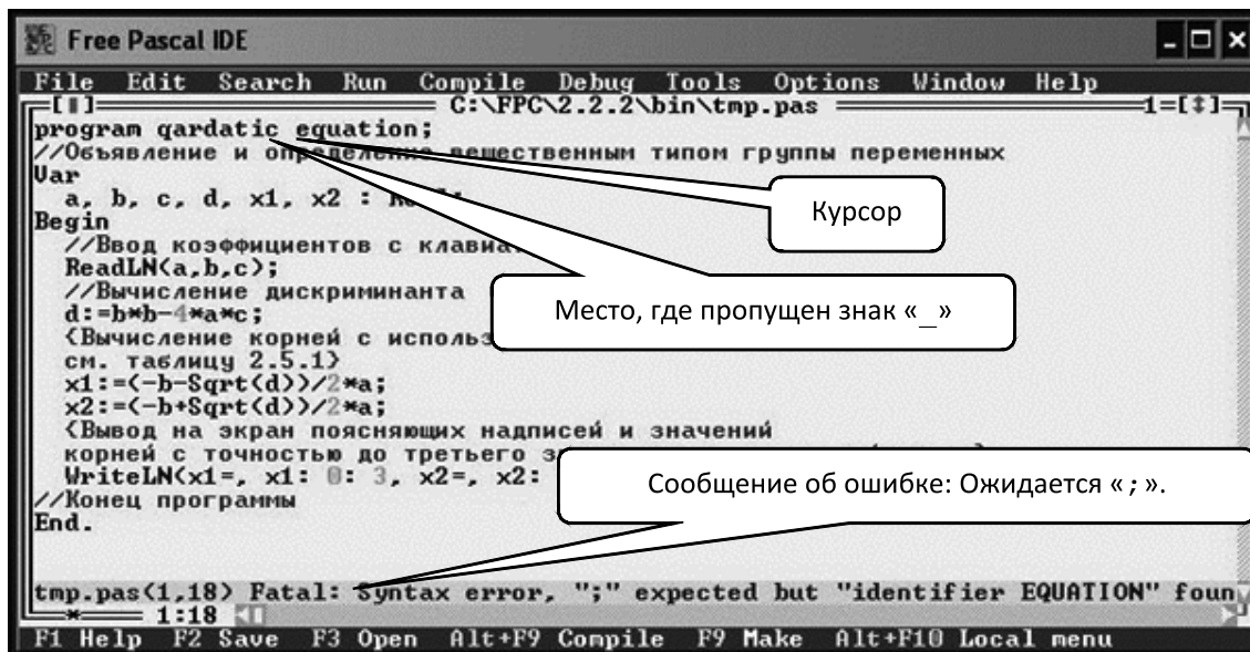
Рис. 2.4 – Экран IDE с первой ошибкой в программе quadratic_equation
