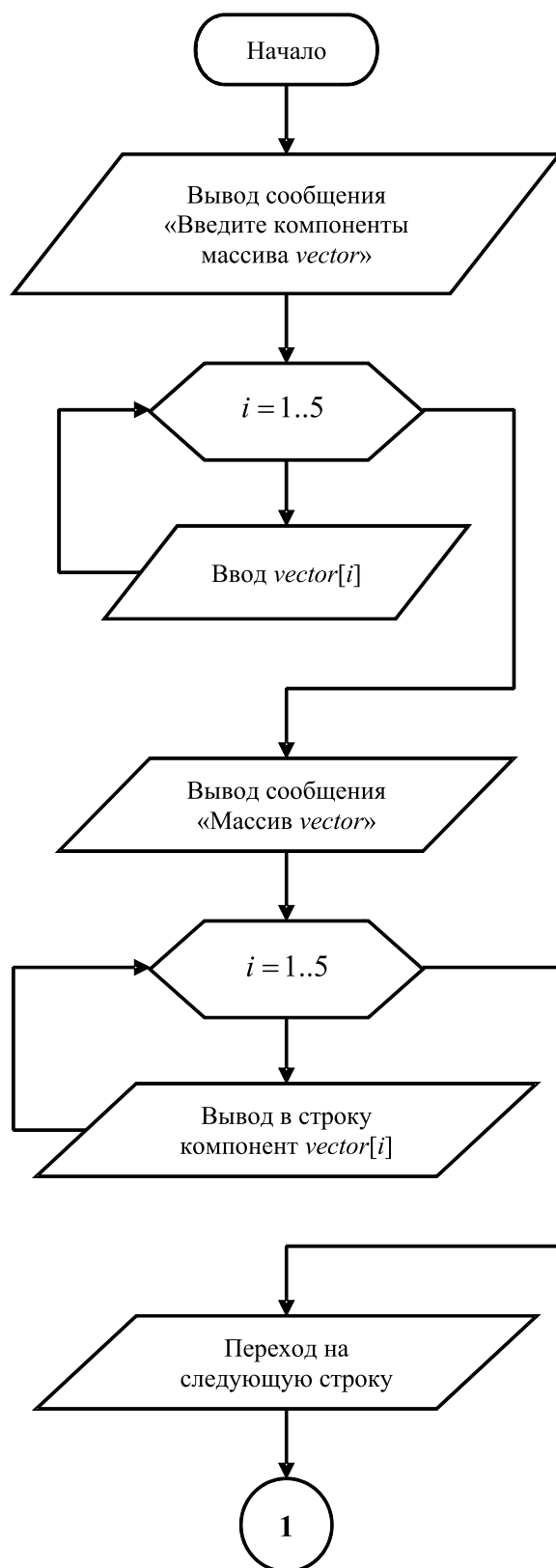
Рис. 3.1 – Блок-схема алгоритма ввода с клавиатуры и вывода на экран одномерного массива
