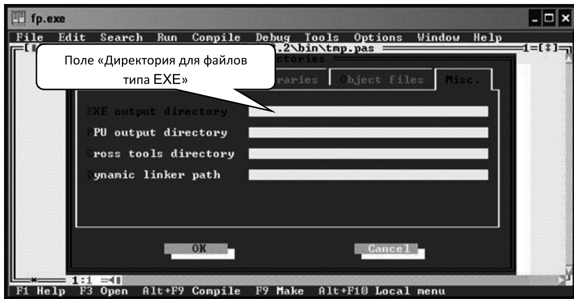
Рис. 5.3 – Экран IDE с окном Directories (директории)
