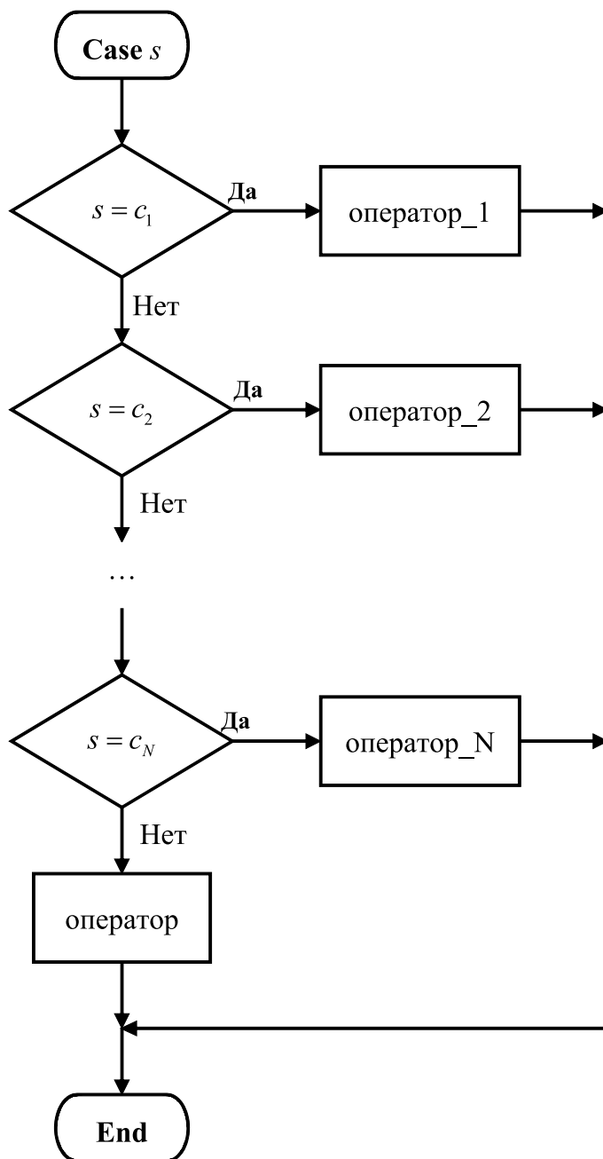
Рис. 2.10 – Блок-схема оператора выбора Case
