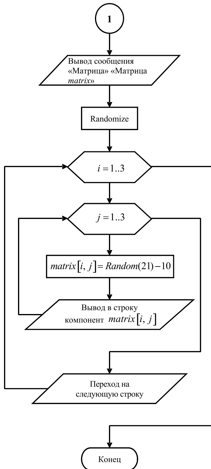
Рис. 3.2 – Блок-схема алгоритма ввода случайным образом и вывода на экран двухмерного массива
