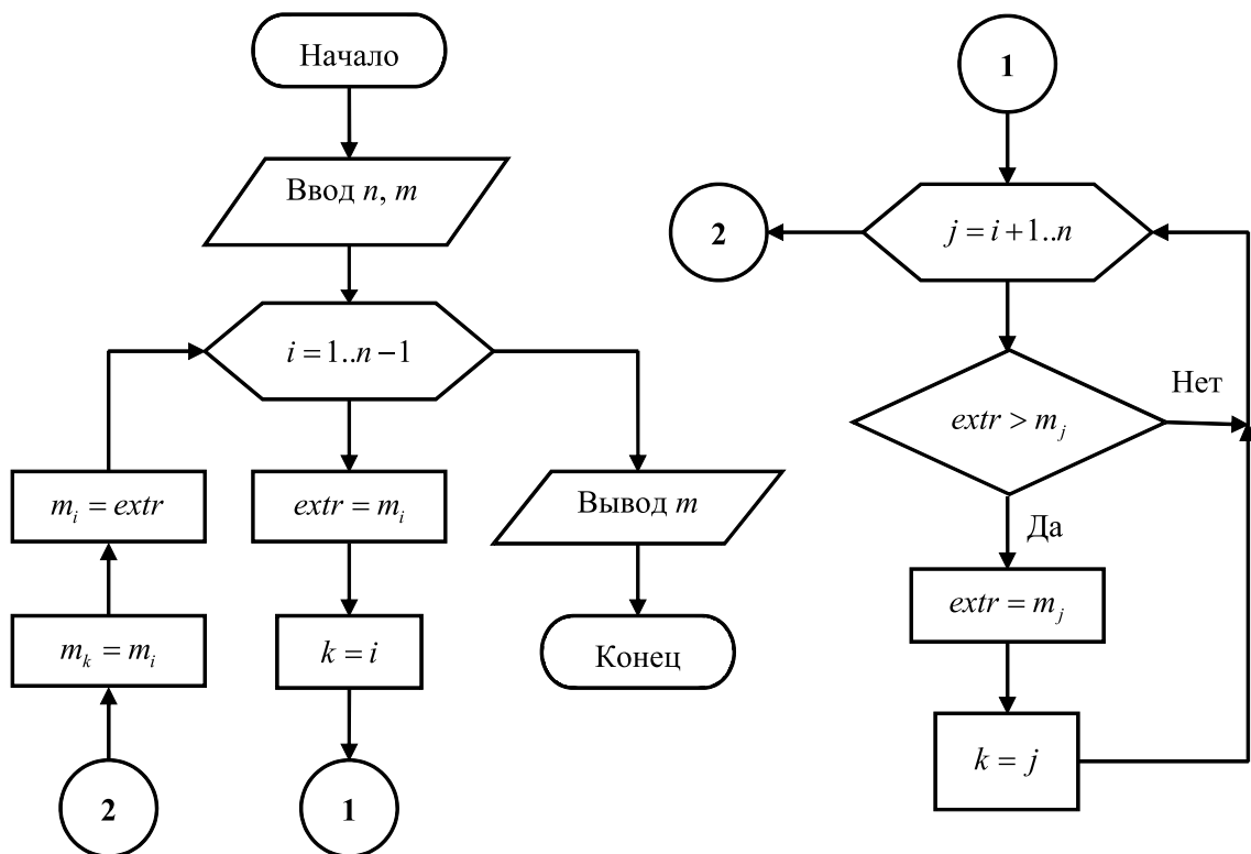
Рис. 3.3 – Блок-схема метода простого выбора
