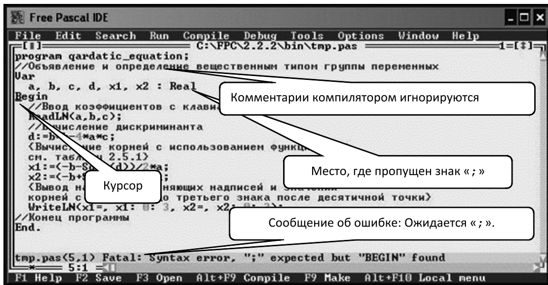
Рис. 2.5 – Экран IDE со второй ошибкой в программе quadratic_equation
