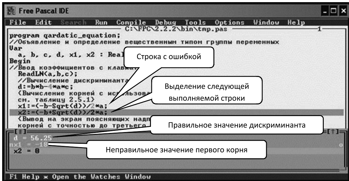
Рис. 2.8 – Экран IDE с трассировкой программы quadratic_equation и с окном Watches
