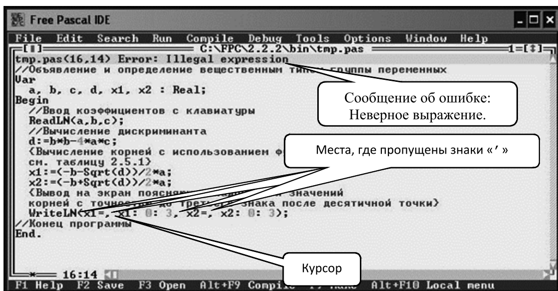
Рис. 2.6 – Экран IDE с третьей ошибкой в программе quadratic_equation
