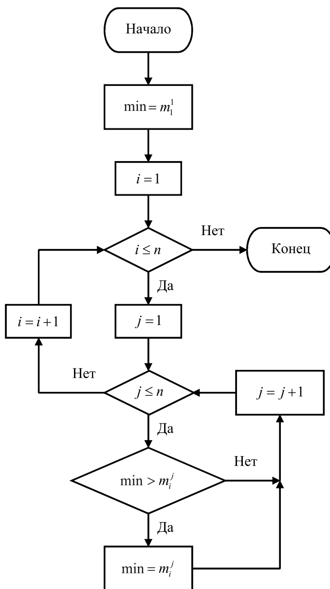
Рис. 1.2 – Блок-схема алгоритма поиска минимального элемента двухмерной матрицы
