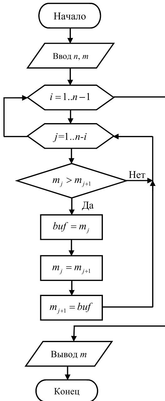
Рис. 3.4 – Блок-схема метода простого обмена
