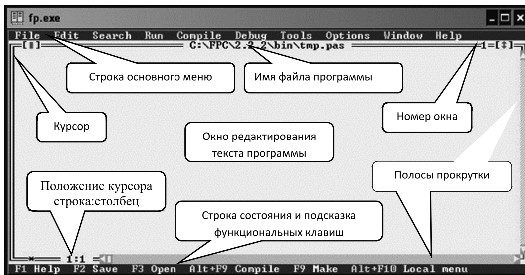
Рис. 5.1 – Экран интегрированной среды Free Pascal
