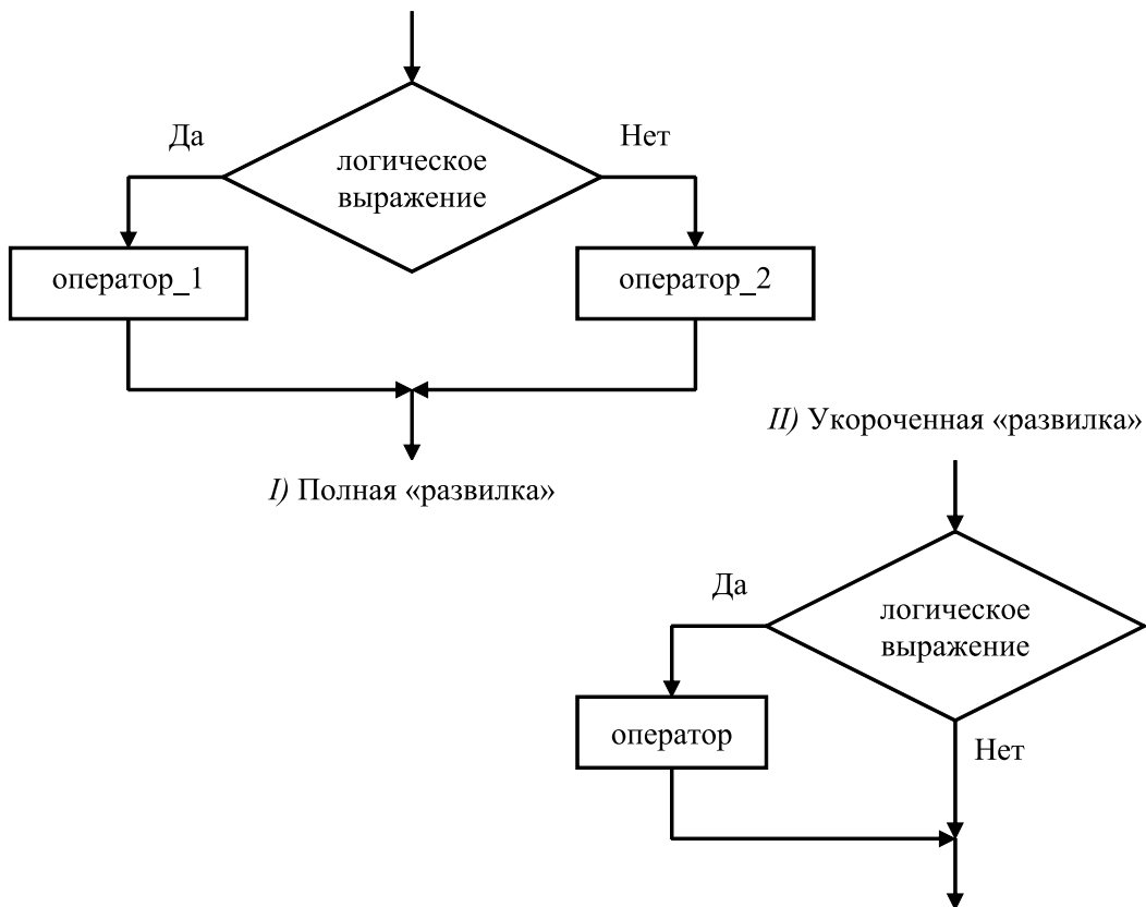
Рис. 2.2 – Блок-схемы двух видов условного оператора If
