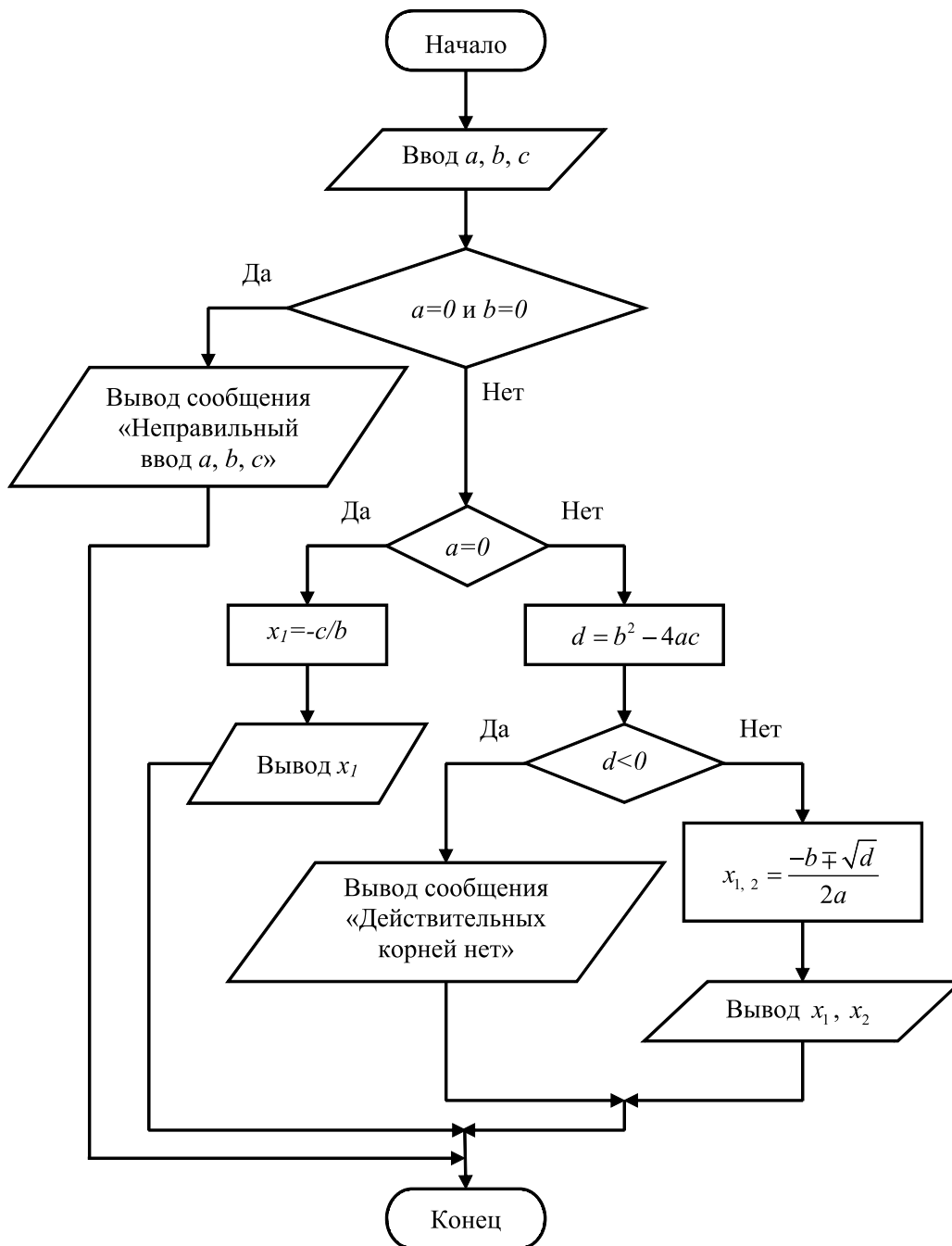
Рис. 2.9 – Блок-схема улучшенного алгоритма решения квадратного уравнения
