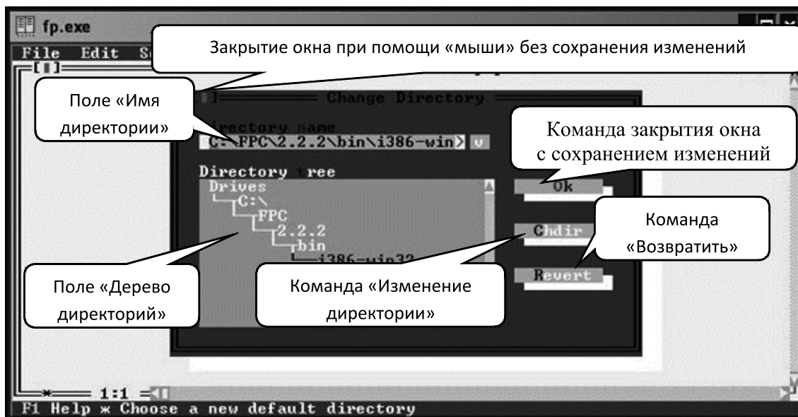
Рис. 5.2 – Экран IDE с окном Change Directory (изменение директории)
