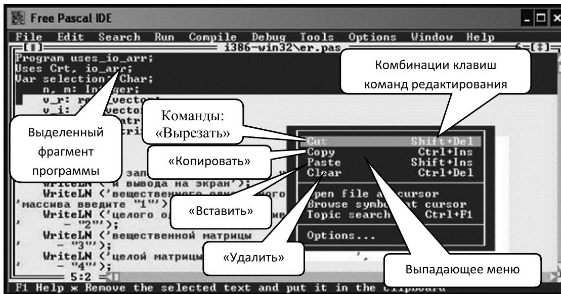
Рис. 5.4 – Экран IDE с выпадающим, при нажатии правой кнопки «мыши», меню
