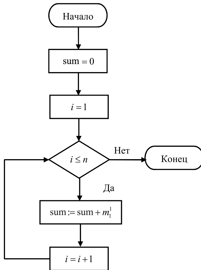
Рис. 1.3 – Блок-схема алгоритма вычисления суммы элементов главной диагонали матрицы
