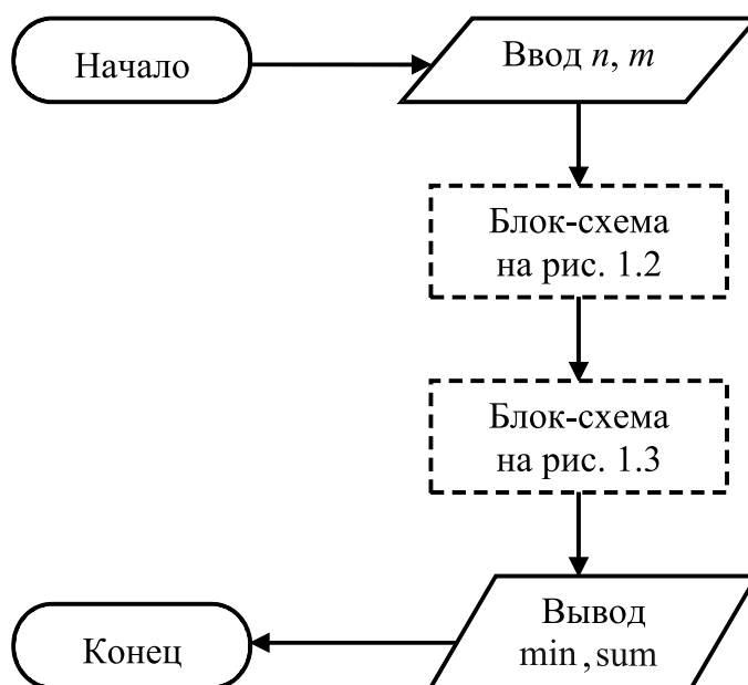
Рис. 1.4 – Блок-схема алгоритма решения задачи из примера 1.1
