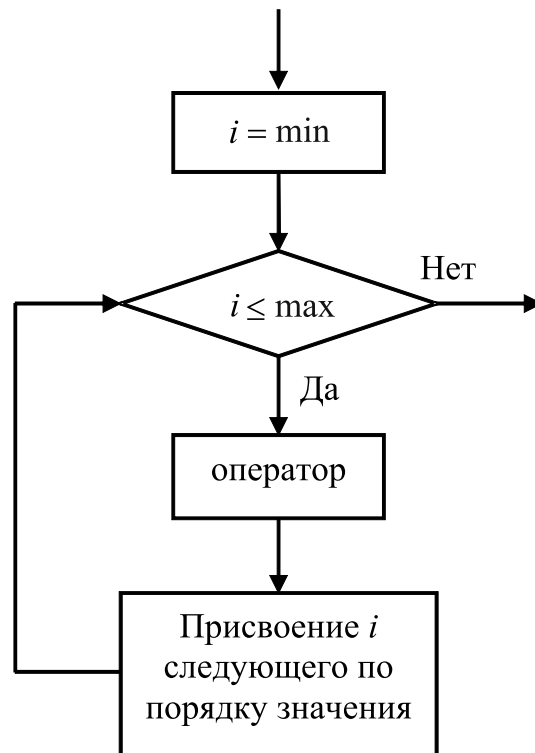
Рис. 2.13 – Блок-схема оператора цикла For
