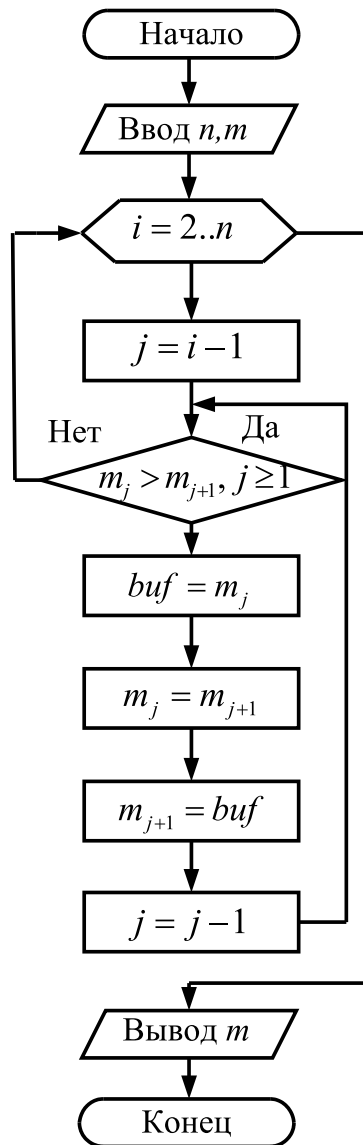
Рис. 3.5 – Блок-схема метода простых вставок
