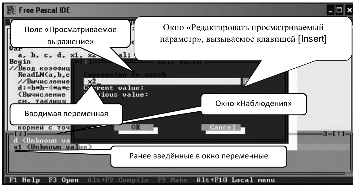
Рис. 2.7 – Экран IDE с окнами Watches и Edit Watch
