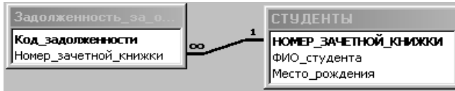
Рис. 23 Схема данных
