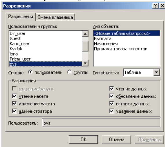
Рис. 1.8. Окно разрешения
