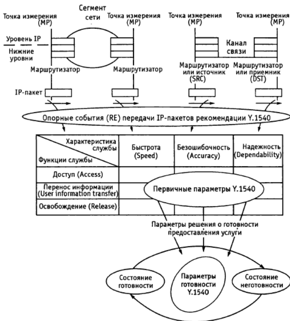
Рис. 6.1. Эталонная модель и область действия рекомендации Y.1540
