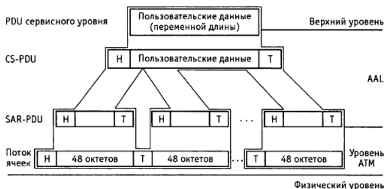
Рис. 3.22. Операции протокола ATM
