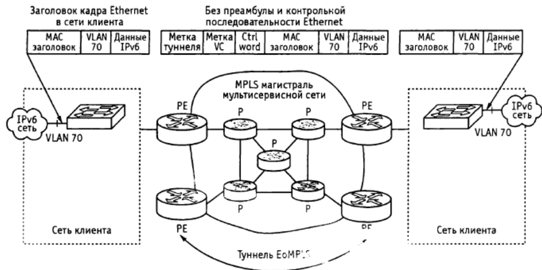
Рис. 6.7. IPv6 по «Ethernet to MPLS»
