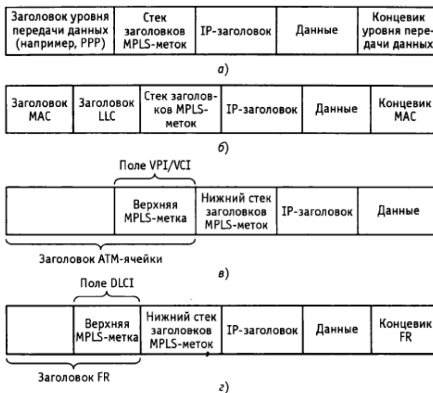
Рис. 4.5. а) Стеки заголовков меток MPLS в протоколе PPP; б) стек заголовков меток в кадре сети стандарта 802.x; в) стек заголовков меток MPLS в поле VPI/VCI; з) стек заголовков меток MPLS в поле DLCI
