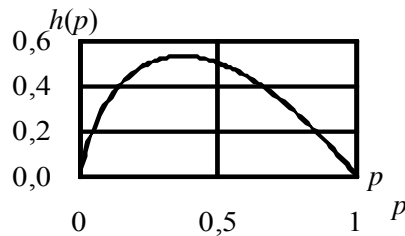
Рис. 4.1. Вспомогательная функция h(p) = -p \log_2 p
