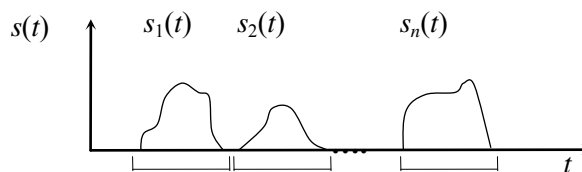
Рис. 6.2 Канальные сигналы, не перекрывающиеся во времени
