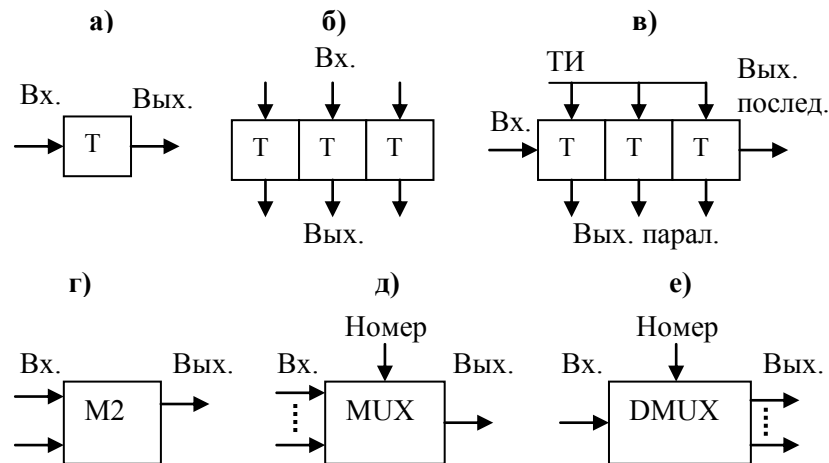
Рис. 2.2. Элементы преобразователей сигналов:
