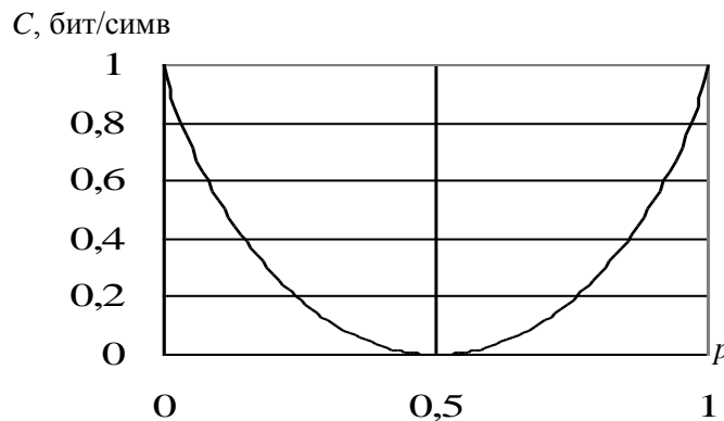
Рис. 4.5. Пропускная способность двоичного симметричного канала без памяти
