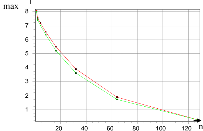
Рисунок 3.5.1 - Зависимость K_{\max}(n, \text{количество каналов})
